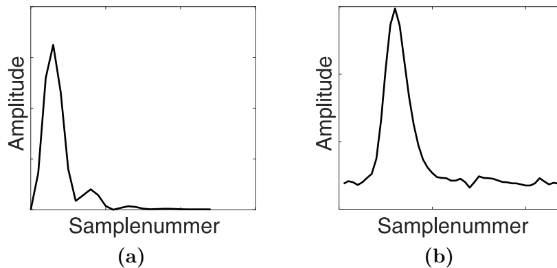
Abb. 2.8 Systemwaveform a des RIEGL VQ-880 (exemplarisch; bereitgestellt durch AHM GmbH) und b des AHAB Chiroptera.
