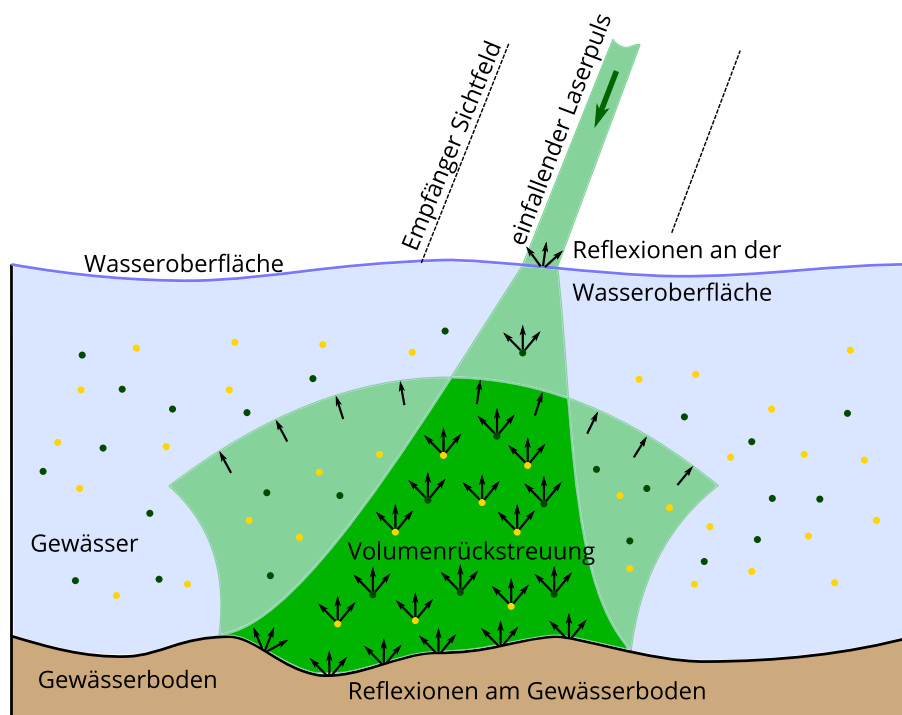
Abb. 2.6 Ausbreitung des Laserpulses in Wasser (Abbildung in Anlehnung an Guenther et al. (2000)). Gewässertrübung wird durch gelbe Punkte (Gelbstoffe) und grüne Punkte (Phytoplankton) repräsentiert. Schwarzen Pfeile symbolisieren die Rückstreuung an der Gewässeroberfläche, an den Partikeln in der Wassersäule und am Gewässerboden.
