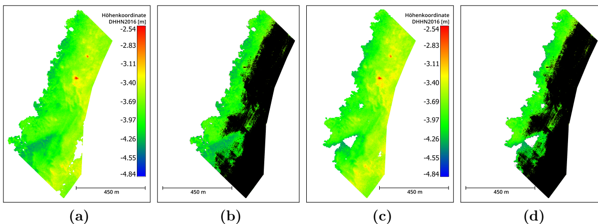
Abb. 4.5 Visualisierung der Prozessierungsergebnisse des signalbasierten ( a, b ) und des volumetrischen Full-Waveform Stackings ( c, d ). a und c zeigen die Ergebnispunktwolke der Full-Waveform Stacking-Prozessierung farbkodiert bzgl. der Höhenkoordinate (DHHN2016). Der mittlere Wasserspiegel lag zum Zeitpunkt der Befliegung zwischen -1,38 m und -1,45 m (DHHN2016). b und d stellt den Flächenvergleich zwischen Abb. a bzw. c und den OWP-Daten (schwarze Punkte) dar.
