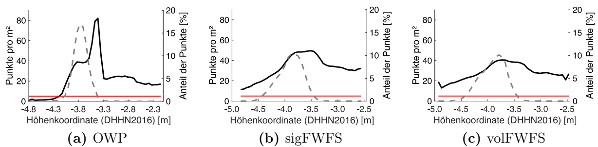
Abb. 4.11 Mittlere Punktdichte in Abhängigkeit der Gewässertiefe. Die horizontale rote Linie stellt die Grenze von 5 Punkte/m 2 dar. Der Anteil der Punkte bezieht sich auf die Gesamtpunktzahl der jeweiligen Punktwolke. Die Anzahl der Punkte pro m 2 ist in schwarz und der Anteil der Punkte als gestrichelte graue Linie dargestellt.
