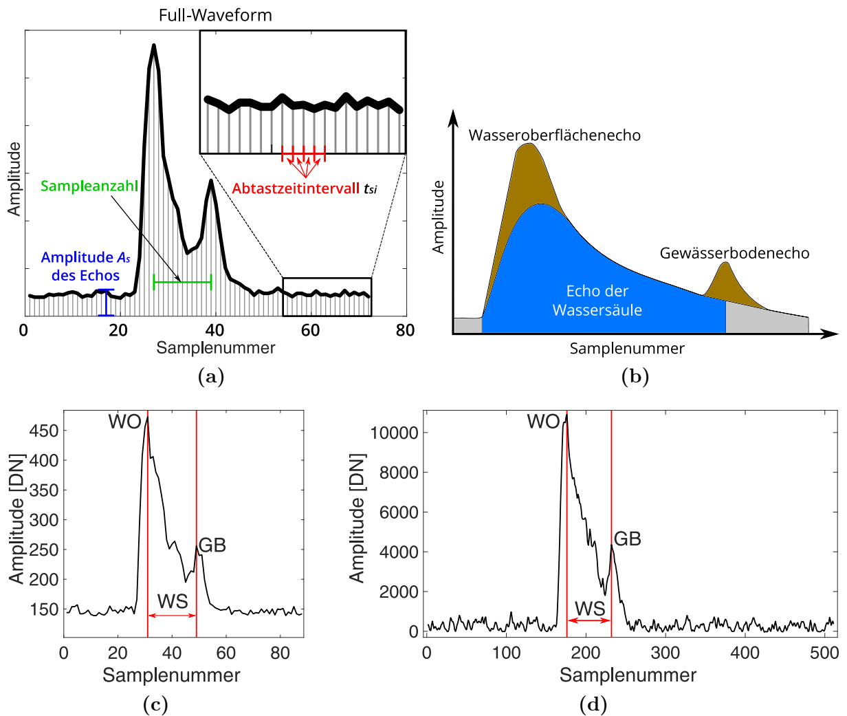
Abb. 2.7 Aufbau einer Full-Waveform a mit zwei Objektechos. b zeigt schematisch eine bathymetrische Full-Waveform mit den drei Signalkomponenten nach Guenther et al. (2000). Beispielhafte Full-Waveform eines c RIEGL VQ-880 ALB-Systems und eines d AHAB Chiroptera ALB-Systems. WO = Wasseroberflächenecho; WS = Echo der Wassersäule; GB = Gewässerbodenecho.
