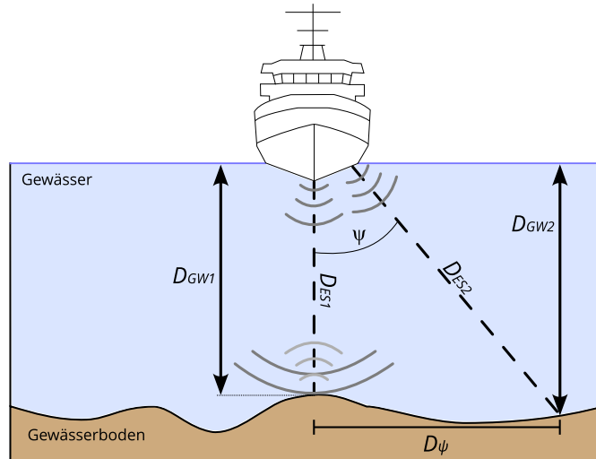
Abb. 2.10 Messprinzip der hydroakustischen Messung für vertikale und schräge Echolotung.
