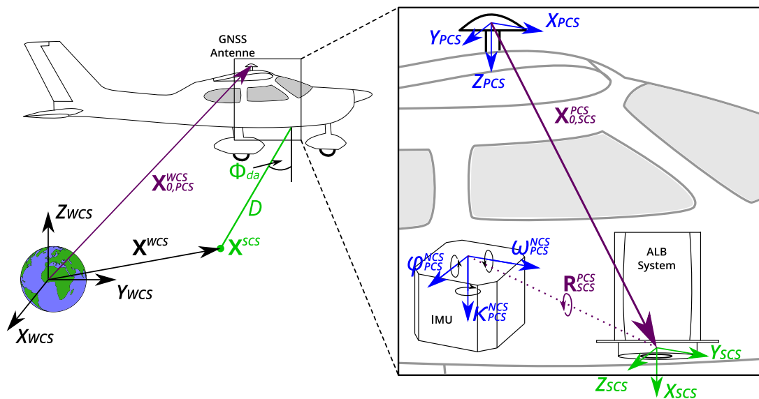
Abb. 2.3 Relevanten Koordinatensysteme vom ALB-Sensor bis zum globalen Koordinatensystem.
