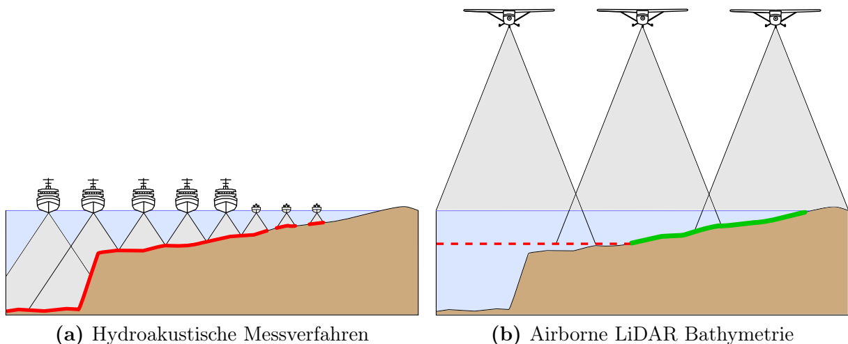
Abb. 2.1 Messverfahren für bathymetrische Messungen (Abbildung in Anlehnung an Guenther et al. (2000)). Hydroakustische Messverfahren können jede Gewässertiefe erreichen, sind aber in der Effizienz der Flächenabdeckung von der Gewässertiefe abhängig. Mit der Airborne LiDAR Bathymetrie kann innerhalb kurzer Zeit sehr viel Fläche gescannt werden, dieses Verfahren ist jedoch limitiert bzgl. der Eindringtiefe in den Wasserkörper (rote gestrichelte Linie in b . Die rote Linie in a und die grüne Linie in b symbolisieren die erfassten Teile des Gewässerbodens.
