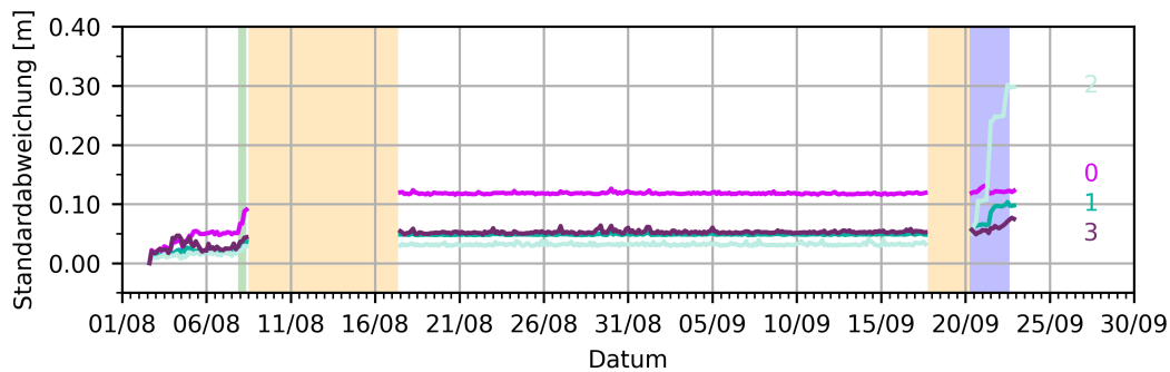
Abb. 6.30.: Standardabweichung aller Zeitreihen als Ergebnis der Segmentierung im limitierten Bereich (4 Cluster).
