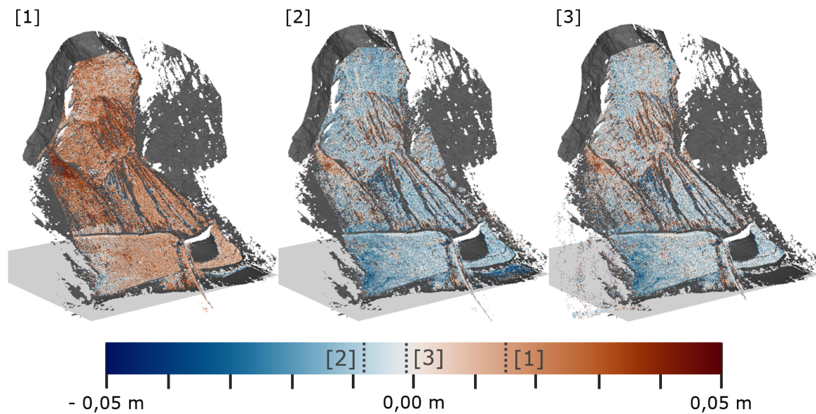
Abb. 5.26.: Der Vergleich verschiedener Registrierungsansätze als «Impact Map». [1]: Keine Registrierung, [2]: Onboard-Registrierung und [3] Helmert-Transformation.
