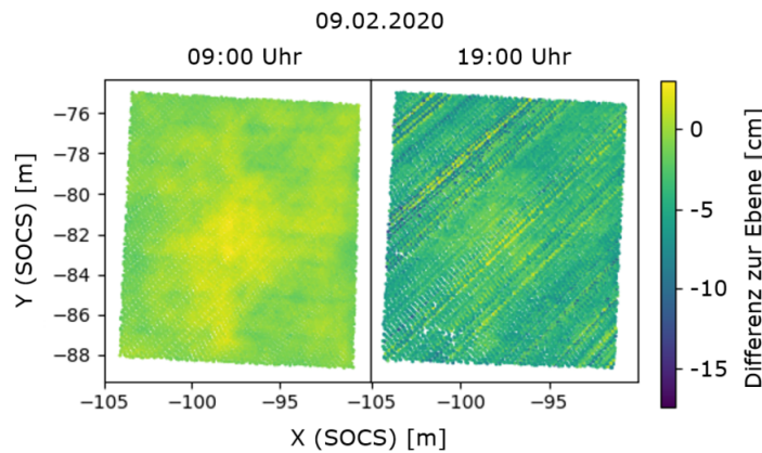
Abb. 5.1.: Darstellung der Residuen auf dem Hubschrauberlandeplatzes am 09.02.2020, um 09:00 (links) und um 19:00 Uhr (rechts).
