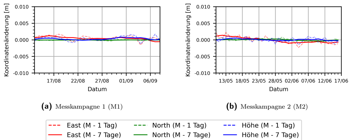
Abb. 5.10.: Messergebnisse der Totalstation. Tages- und Wochenmittel der Koordinaten und zusätzliche Mittelbildung über alle Prismen in den Zeiträumen M1(links) und M2 (rechts). Gestrichelt = Tagesmittel; Durchgezogen = Wochenmittel.
