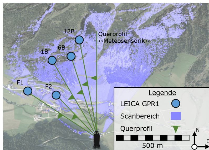
Abb. 5.13.: Draufsicht auf das Messgebiet mit Darstellung des Laserscanners, der ausgewählten Prismen und der zugehörigen Querprofile einschließlich der jeweiligen Blickrichtung auf die Profilzeichnungen (Abb. 5.23 und 5.24). Orthofoto: Land Tirol - « data.tirol.gv.at ».
