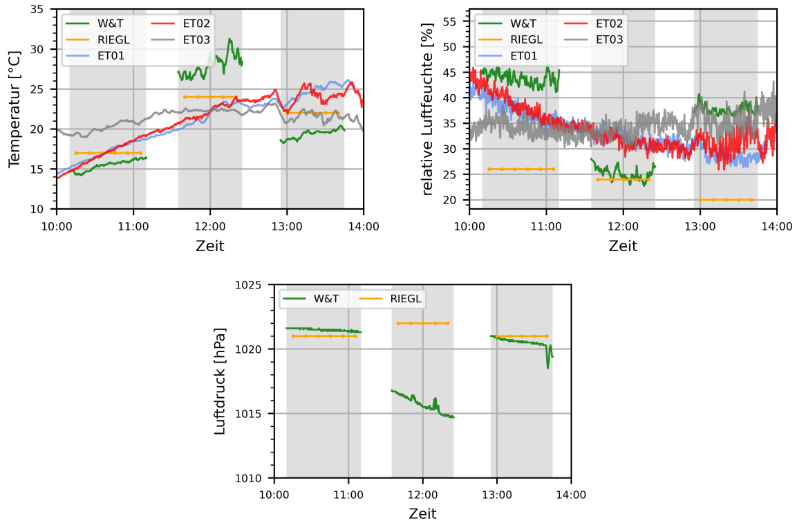
Abb. 5.9.: Meteorologische Messwerte am 21.03.2022 an der Kalibrierbasis in Unna-Hemmerde. Darstellung der internen Messwerte des Scanners und W&T #57713 während der Aufstellungen STP1, STP2 und STP3 (Graue Zeitfenster) sowie die kontinuierlichen Messreihen der Sensoren ELITECH #RC-51H (ET01 bis ET03) an den Messpfeilern entsprechend Abb. 5.8. Die Daten von «ET04» sind nicht verfügbar.
