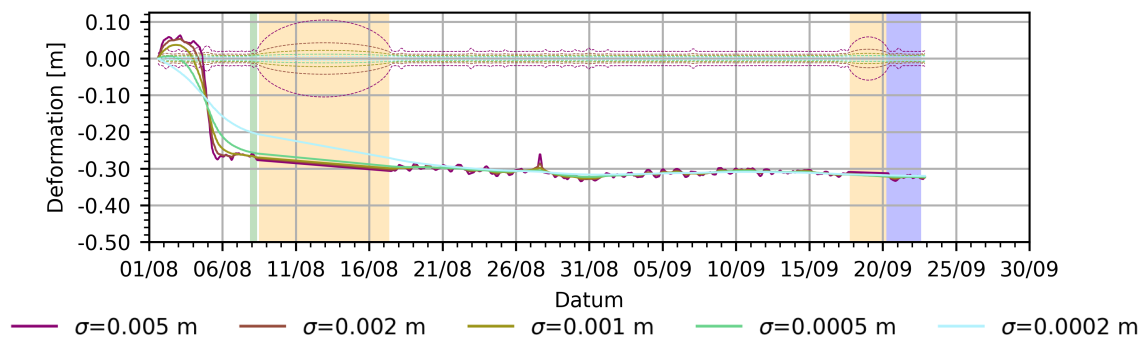
Abb. 6.35.: Ergebnisse der Kalman-Filterung an Corepoint 4.
