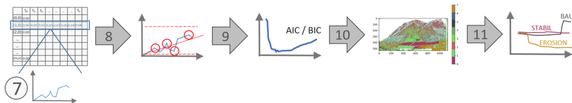
Abb. 6.18.: Workflow zur Zeitreihensegmentierung mittels tsfresh und GMM.
