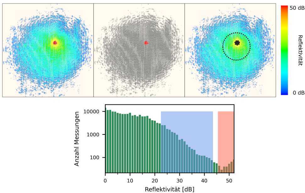
Abb. 5.7.: Detektion von Corner Cube Prismen aus den hochauflösenden Scandaten. Oben Links: Prismenscan eingefärbt nach der Reflektivität. Oben Mitte: Darstellung der Punkte oberhalb von «Cut high». Oben Rechts: Darstellung der Punkte zwischen «Cut low» und «Cut high». Unten: Darstellung der Reflektivitäten eines Prismenscans als Histogramm. Im blauen Bereich liegen die Werte zwischen «Cut low» und «Cut high». Im roten Bereich liegen die Werte oberhalb von «Cut high».
