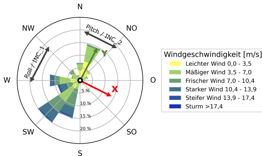
Abb. 5.3.: Relative Ausrichtung der Neigungssensoren in Bezug auf das SOCS des PLS im Zentrum der Grafik. Zusätzlich sind die Hauptwindrichtungen im Beobachtungszeitraum dargestellt.
