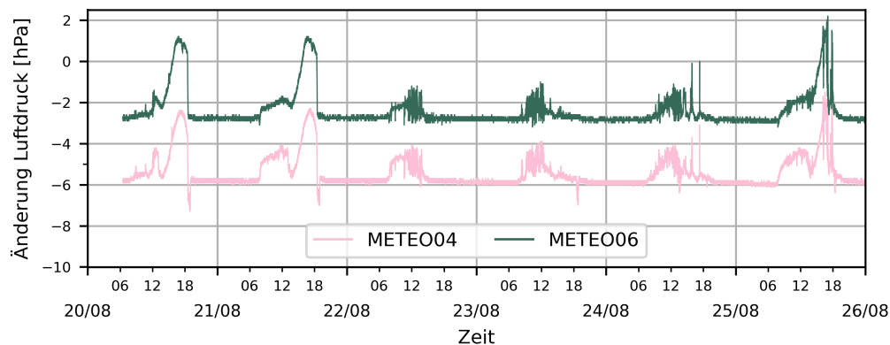
Abb. 5.21.: Differenz des Luftdrucks von «METEO04» und «METEO06» im Vergleich zu «METEO05».
