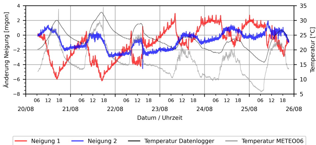
Abb. 5.16.: Messwerte der Neigungssensorik an der Inklinometerplatte am Laserscanner in vergleichender Darstellung mit der Temperatur des Datenloggers und an «METEO06».
