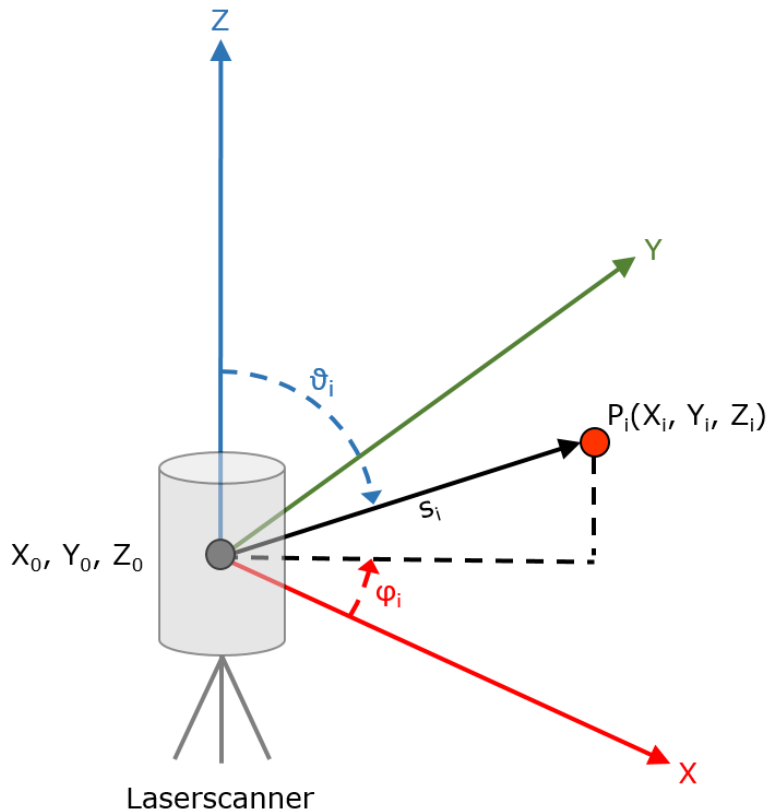
Abb. 2.5.: Koordinatensystem des TLS ausgedrückt im SOCS. Darstellung eines Punktes P_i in polaren und kartesischen Koordinaten.
