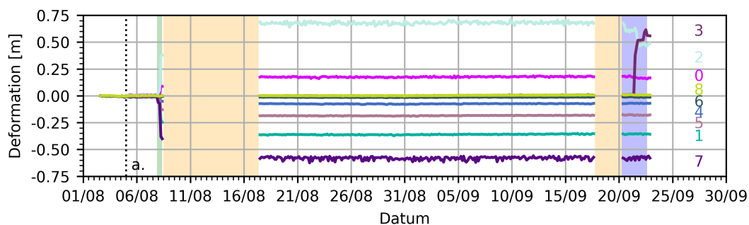
Abb. 6.17.: Median aller Zeitreihen als Ergebnis der Segmentierung im limitierten Bereich ( k=9 ).
