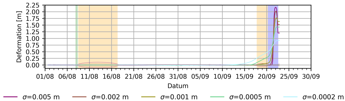
Abb. 6.37.: Ergebnisse der Kalman-Filterung an Corepoint 6.
