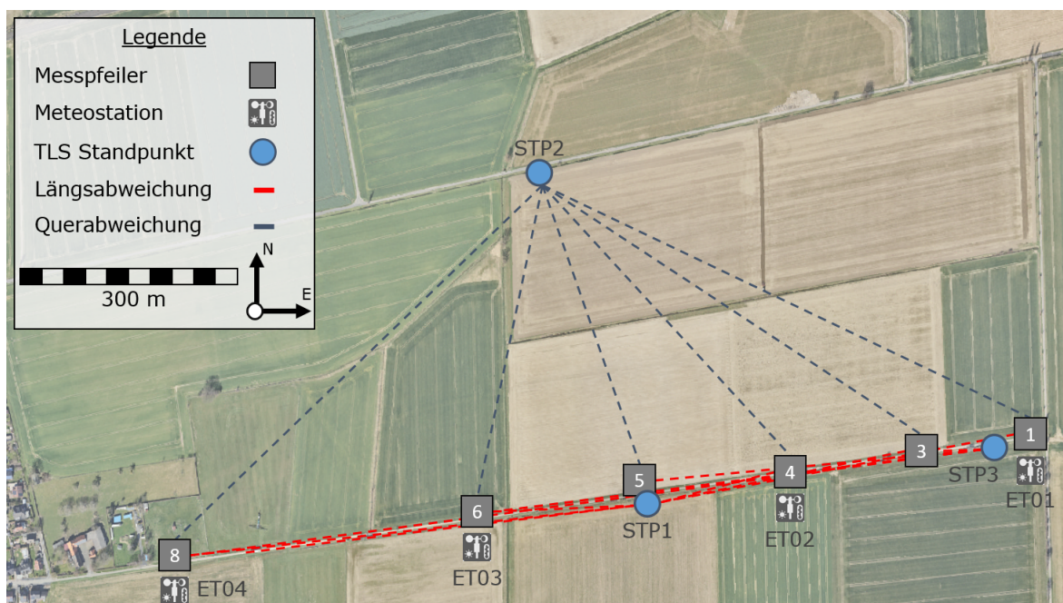
Abb. 5.8.: Räumliche Darstellung der Kalibrierbasis in Unna-Hemmerde. Es werden die Scannerstandpunkte (blaue Punkte) in Bezug zu den Messpfeilern (graue Vierecke) mit den entsprechenden Anzielungen (gestrichelt) visualisiert.
