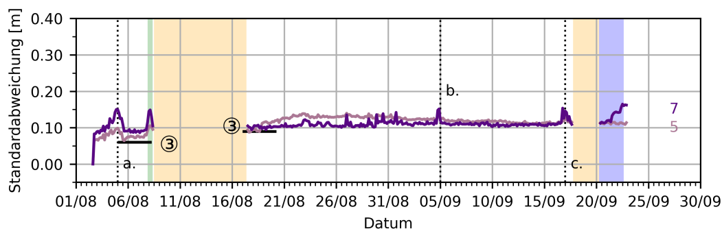
Abb. 6.22.: Standardabweichung der Zeitreihen von Klasse C. (5) und D. (7) für 12 Cluster.
