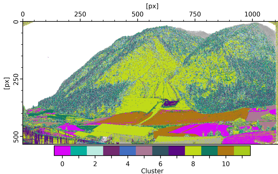
Abb. 6.20.: Räumliche Darstellung des Segmentierungsergebnis für 12 Cluster.
