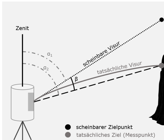
(a) Refraktionswinkel (pos.), Strahl ist zur Erde hin gekrümmt.
