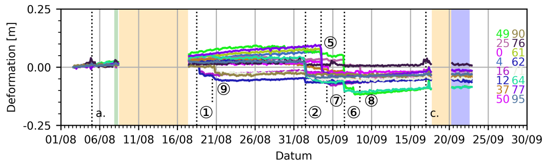
Abb. 6.24.: Mittelwert der Zeitreihen von Klasse B. für 100 Cluster.
