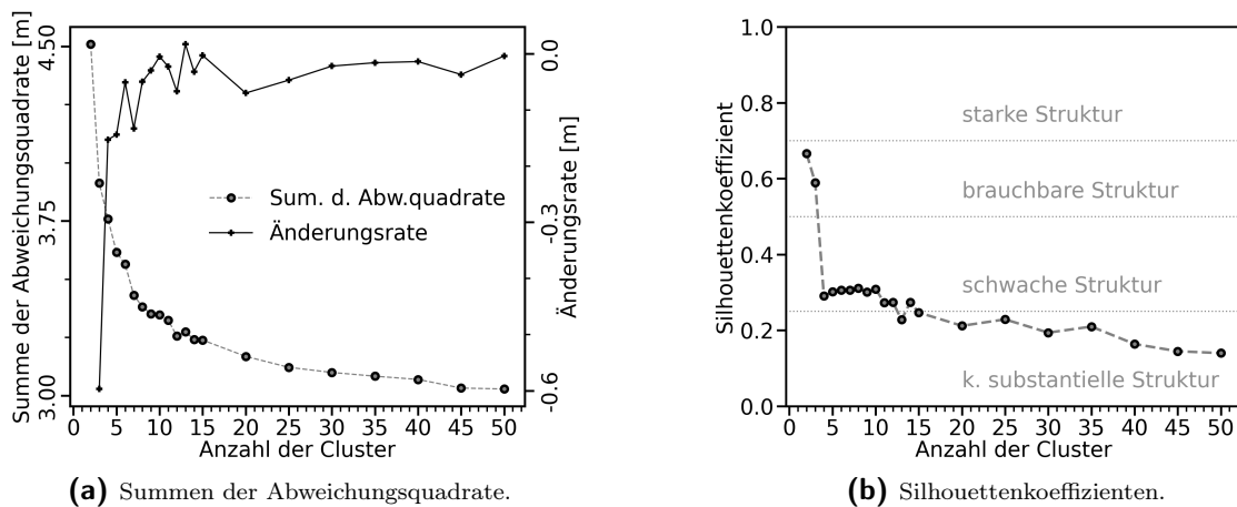
Abb. 6.7.: Kombinierte Betrachtung der beiden Auswahlkriterien - Summen der Abweichungsquadrate und Silhouettenkoeffizient.
