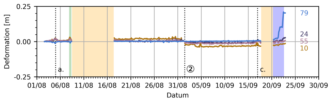
Abb. 6.25.: Mittelwert der Zeitreihen von Klasse D. für 100 Cluster.
