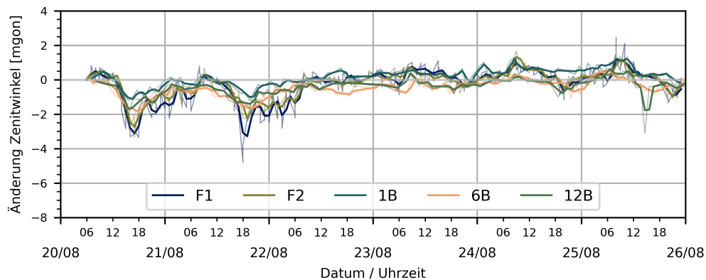
Abb. 5.19.: Zeitreihen der Zenitwinkeländerungen - erfasst mittels Totalstation.
