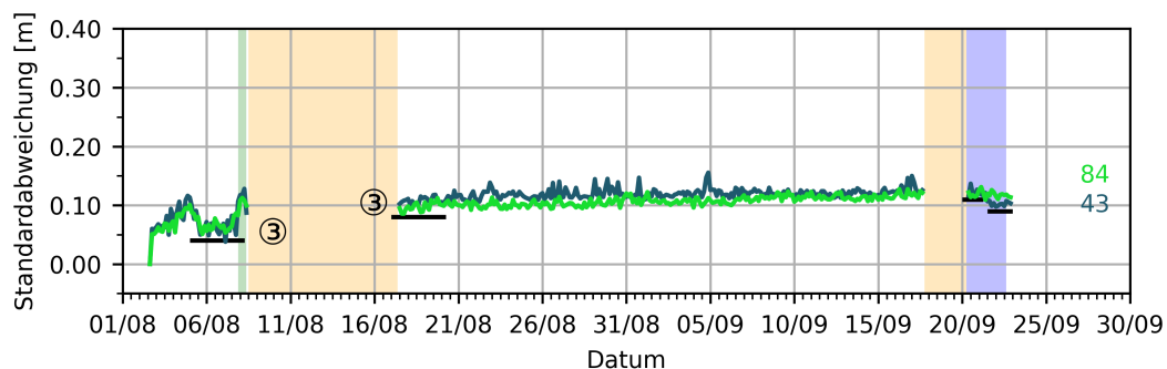
Abb. 6.26.: Standardabweichung der Zeitreihen von Klasse C. für 100 Cluster.
