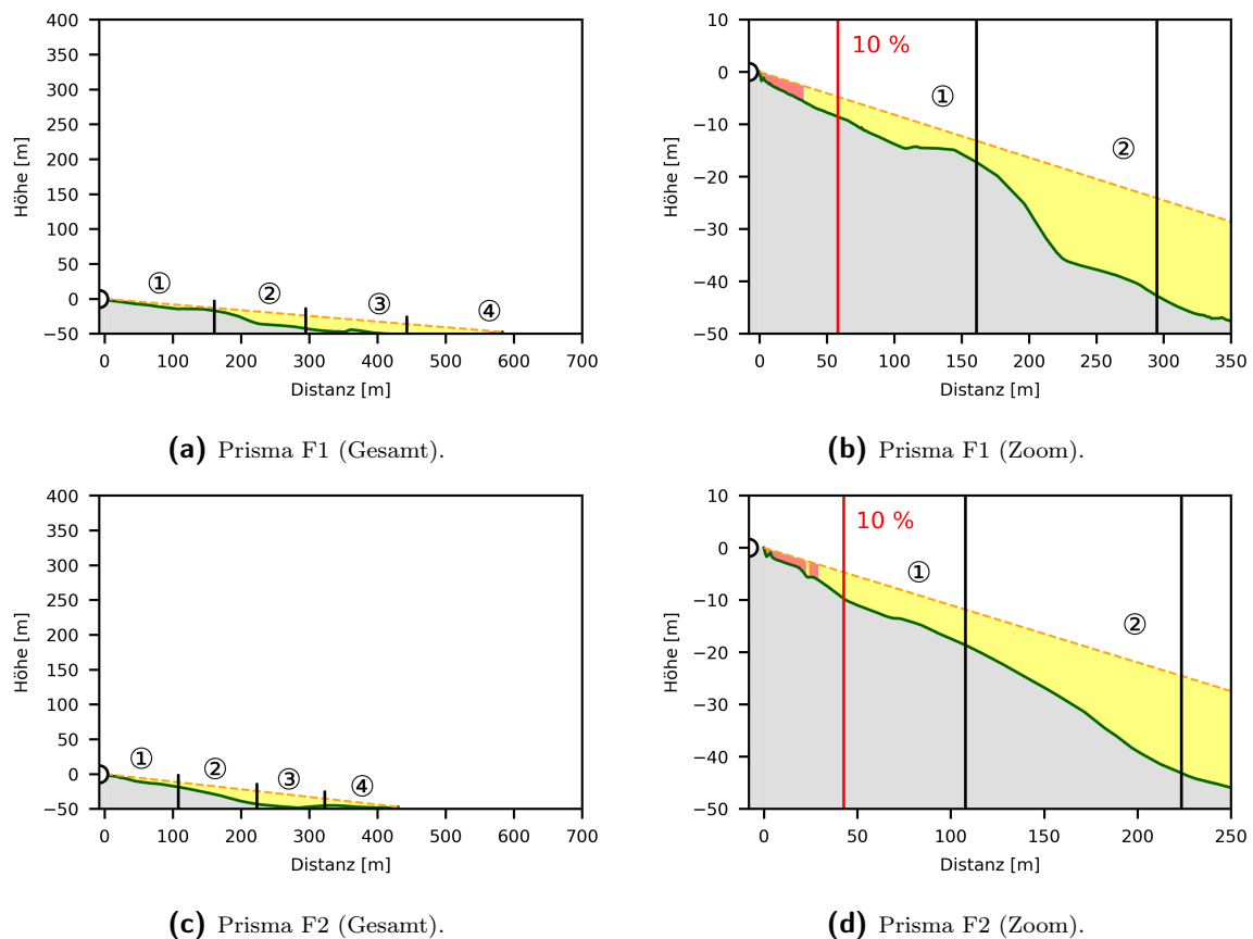
Abb. 5.23.: Messdaten in Bezug zur Topographie im Valsertal. Vertikalschnitte entlang der Querprofile (Abb. 5.13) - Teil I. Links: Vertikalschnitt des gesamten Messwegs, gleichartig skaliert. Rechts: Zoom auf die ersten beiden Viertel im Vertikalschnitt und Darstellung der ersten 10 % des Messwegs.
