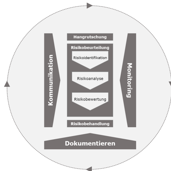
Abb. 2.3.: Darstellung des Risikomanagementprozess für eine Hangrutschung u.a. als systematische Anwendung von Grundsätzen. Darstellung auf Basis der DIN ISO 31000:2018-10 (2018).
