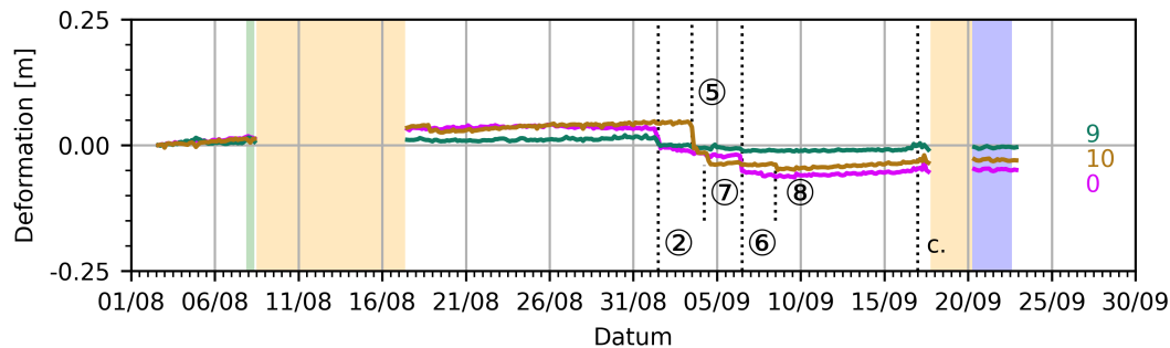
Abb. 6.21.: Mittelwert der Zeitreihen von Klasse B. für 12 Cluster.
