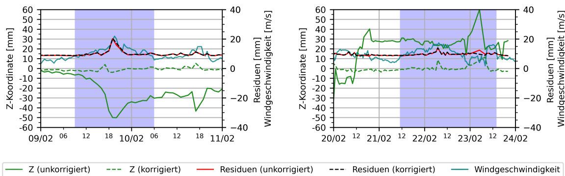
Abb. 5.5.: Berechnung der Ebene am Hubschrauberlandeplatz und Vergleich der Parameter mit den Wetterdaten während der Stürme «Ciara» (links) und «Yulia» (rechts). Die Zeiträume der Stürme sind blau markiert. Der Sprung in der mittleren Z-Koordinate des Hubschrauberlandeplatzes um die Mittagszeit am 20.02.2020 wurde durch Wartungsarbeiten verursacht.
