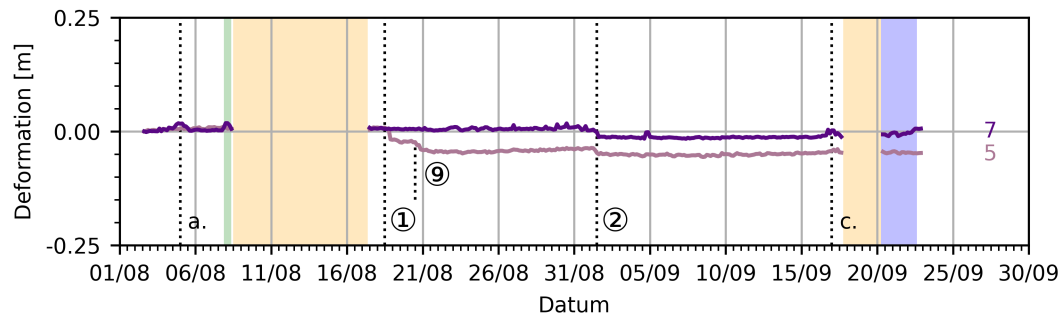
Abb. C.8.: Mittelwert der Zeitreihen von Klasse C. und D. für 12 Cluster.
