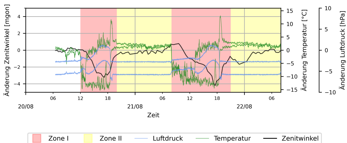
Abb. 5.22.: Vergleichende Darstellung der Zenitwinkeländerung an Prisma «F1» zusammen mit der Änderung von Temperatur und Luftdruck als Differenz der Stationen «METEO04» und «METEO06» gegenüber der Station «METEO05» am 20. und 21.08.2020.
