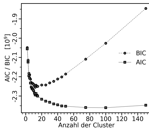
Abb. 6.19.: BIC und AIC für verschiedene Modellberechnungen mittels GMM.
