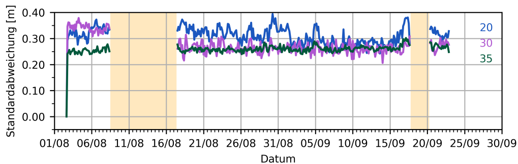
Abb. B.20.: Standardabweichung aller Zeitreihen als Ergebnis der Segmentierung für k=50 .
