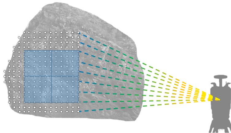
Abb. 6.2.: Transformation der 3D-Punktdaten in eine rasterbasierte Repräsentation.
