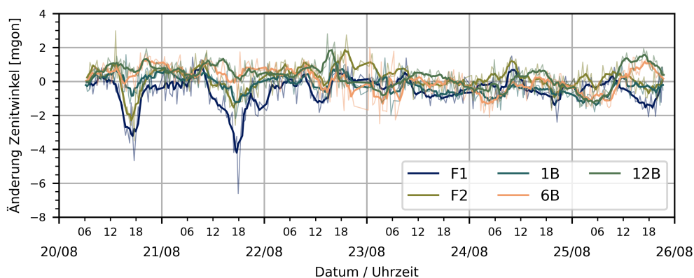
Abb. 5.18.: Zeitreihen der korrigierten Zenitwinkeländerungen - erfasst mittels Laserscanner.
