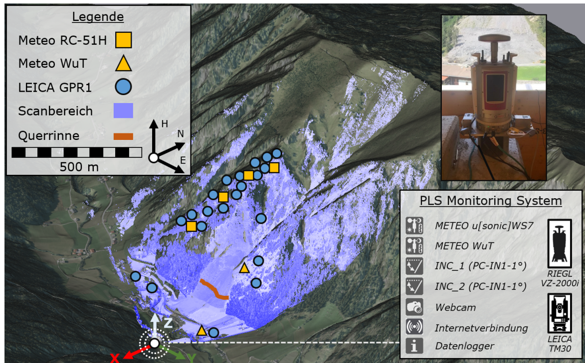
Abb. 5.11.: Dreidimensionale Darstellung des Testgebietes am Felssturz im Valsertal mit integrierter Sensortechnik, deren räumliche Lage zueinander sowie Darstellung der hergestellten Querrinne. DGM und Orthofotos: Land Tirol - «data.tirol.gv.at» .
