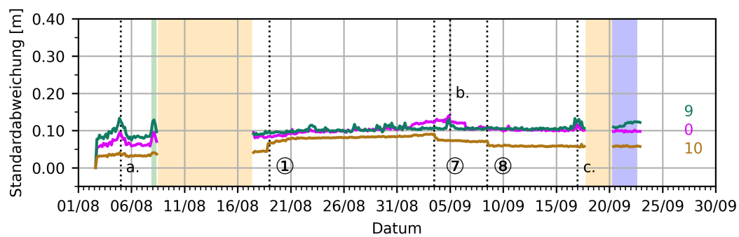
Abb. C.7.: Standardabweichung der Zeitreihen von Klasse B. für 12 Cluster.
