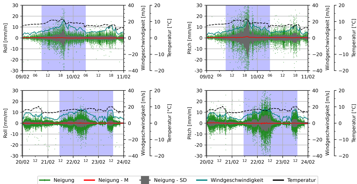
Abb. 5.4.: Messwerte der internen Inklinometer im Zeitraum von Sturm «Ciara» (Oben) und den Sturm «Yulia» (Unten). Die Zeiträume der Stürme sind blau markiert. Messwerte, Mittelwerte und Standardabweichungen der Neigungsdaten werden mit Temperatur und Windgeschwindigkeit verglichen.
