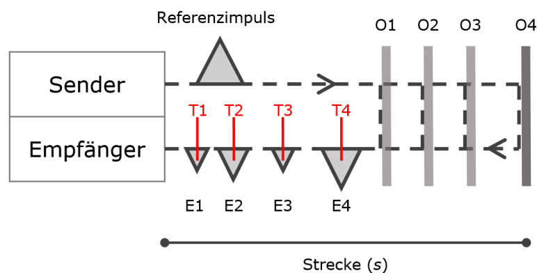
Abb. 2.8.: Schema der Wellenformanalyse mittels «Full waveform data». Basierend auf Ullrich und Pfennigbauer (2011).
