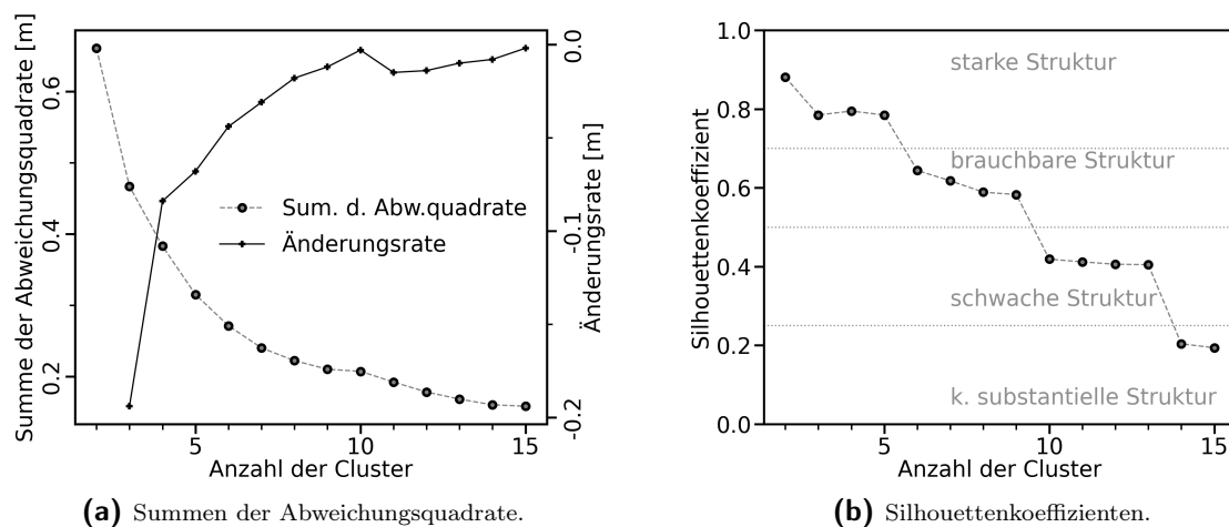
Abb. 6.15.: Kombinierte Betrachtung der beiden Auswahlkriterien - Summen der Abweichungsquadrate und Silhouettenkoeffizient - im räumlich reduzierten Bereich.
