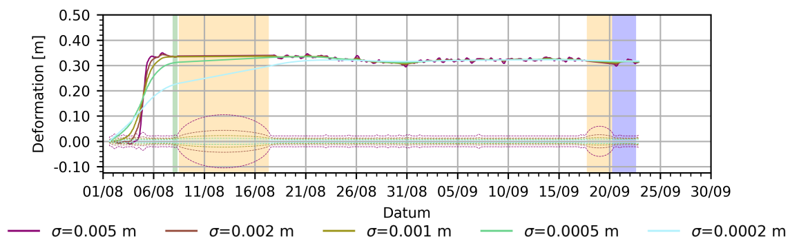
Abb. 6.36.: Ergebnisse der Kalman-Filterung an Corepoint 5.
