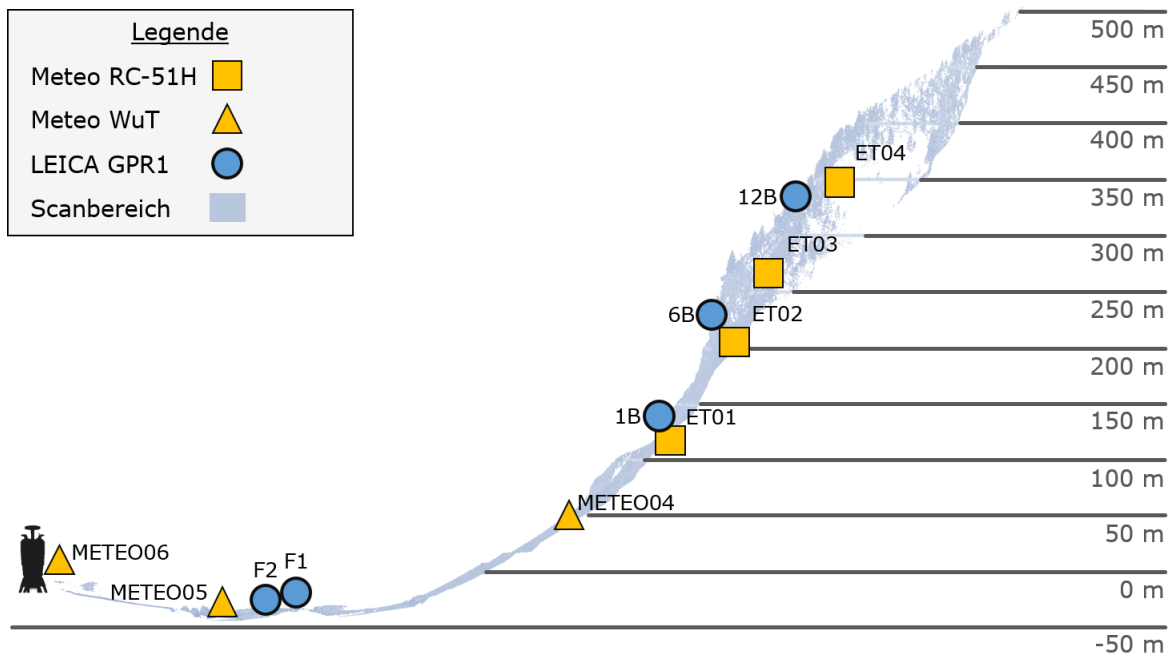
Abb. 5.12.: Skizzierung eines Vertikalschnitts entlang des Querprofils «Meteosensorik» (Abb. 5.13) mit Darstellung des Laserscanners, der ausgewählten Prismen und der verteilten meteorologischen Sensoren im Messgebiet.
