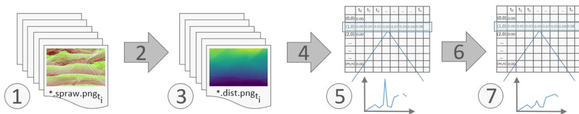
Abb. 6.5.: Workflow zur Extraktion von Zeitreihen aus 3D-Punktwolken.
