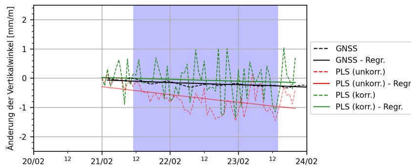
Abb. 5.6.: Vertikalwinkeländerung zwischen Container und der Horizontalen: Vergleich der Ebenenmodellierung aus unkorrigierten (unkorr.), korrigierten (korr.) PLS-Daten und den vier GNSS Antennen. Die Zeitraum von Sturm «Yulia» ist blau markiert.
