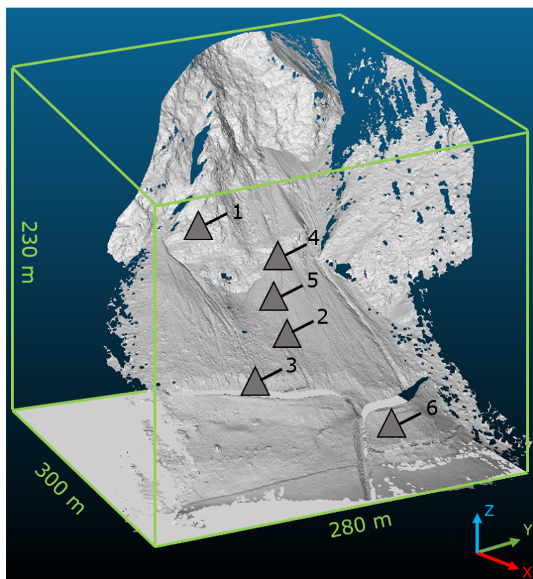
Abb. 6.31.: Übersicht zu den ausgewählten Corepoints aus der 3D-Punktwolke im limitierten Bereich.
