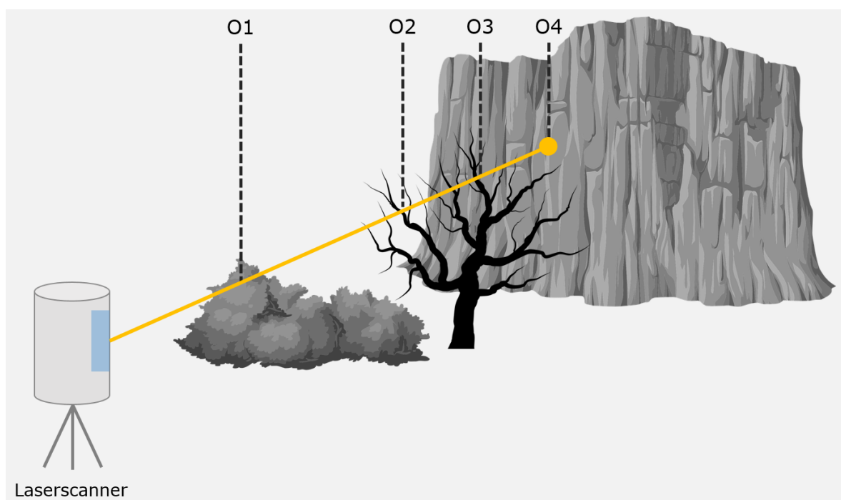
Abb. 2.7.: Grafische Darstellung der Interaktion eines ausgesendeten Messstrahls mit verschiedenen Objekten. Basierend auf Ullrich und Pfennigbauer (2011).
