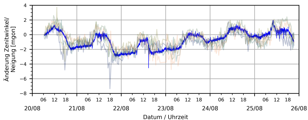
Abb. 5.17.: Vergleich der Zenitwinkeländerung an den Prismen gegenüber den Neigungsänderungen an «Neigung 2» (blau).
