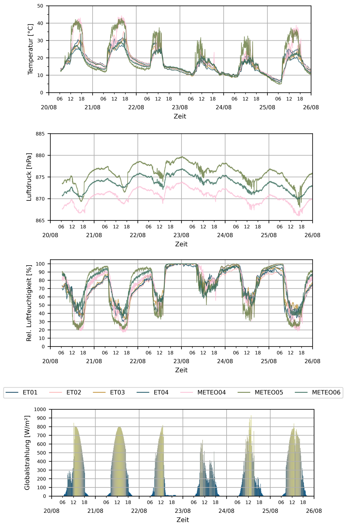
Abb. 5.20.: Meteorologische Daten (Temperatur, Luftdruck und relative Luftfeuchtigkeit) an den Stationen im Messgebiet sowie die Globalstrahlung an der Wetterstation «STEINACH» eingefärbt von dunkel (wenig Strahlung) nach hell (viel Strahlung).
