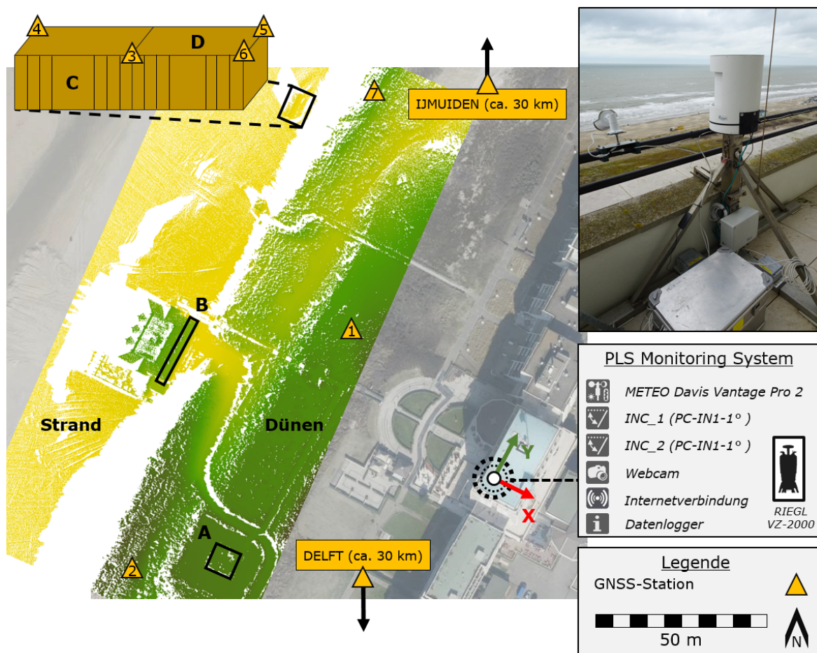
Abb. 5.2.: Räumliche Darstellung der Messkonfiguration in Noordwijk / NL. Punktwolke des Untersuchungsgebiets vom 20.02.2020, 01:00 Uhr mit den durch die Buchstaben A-D gekennzeichneten Referenzebenen (Tab 5.2) und Position der GNSS-Sensoren auf dem Containerdach und in den Dünen (1 - 7). Hintergrundbild: PDOK.nl - «Luchtfoto 2022 Ortho 8cm RGB».
