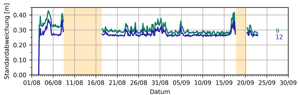
(c) Standardabweichung Klasse C.
