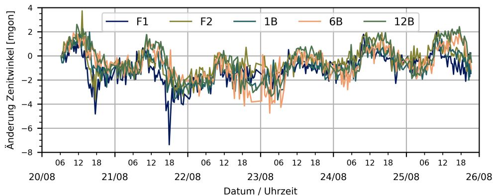
Abb. 5.14.: Zeitreihen der Zenitwinkel ( \vartheta ) der ausgewählten Prismen im unkorrigierten SOCS.
