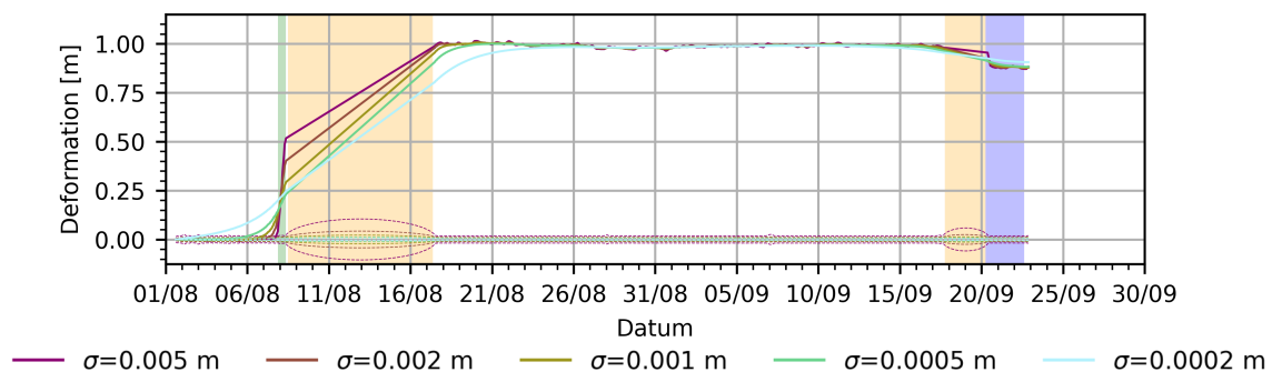
Abb. 6.34.: Ergebnisse der Kalman-Filterung an Corepoint 3.
