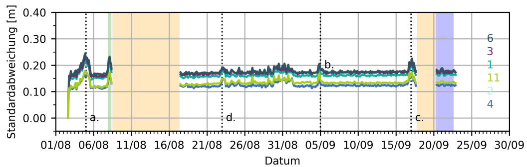
Abb. C.10.: Standardabweichung der Zeitreihen von Klasse E. für 12 Cluster.
