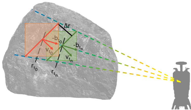
Abb. 6.4.: Darstellung des formellen Zusammenhangs bei der Bildung von Streckendifferenzen zwischen zwei Messungen.
