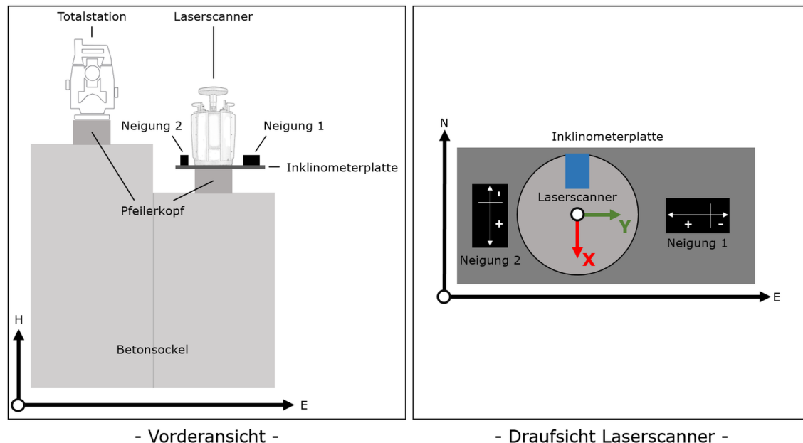
Abb. 5.15.: Skizzierung des technischen Aufbaus der Messeinrichtungen in der Schutzhütte im Valsertal. Links ist die Vorderansicht der Systemkonfiguration bestehend aus Laserscanner, Totalstation und Neigungssensorik zu sehen. Rechts die Draufsicht auf den Laserscanner mit der Anordnung der Neigungssensoren.
