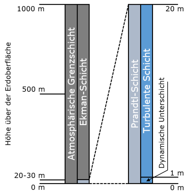
Abb. 2.11.: Aufbau der atmosphärischen Grenzschicht nach Foken (2016).
