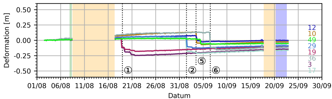
Abb. 6.13.: Median der Zeitreihen von Klasse B. für k=50 .
