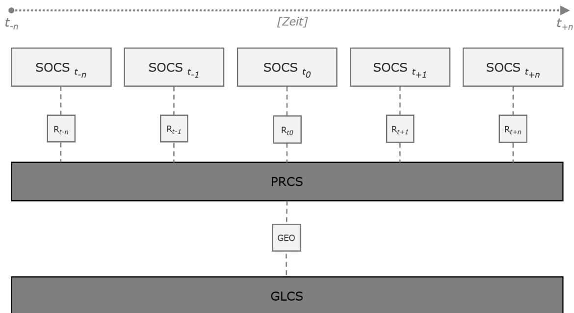
Abb. 2.9.: Schema zur Registrierung und Georeferenzierung multitemporaler Punktwolken.
