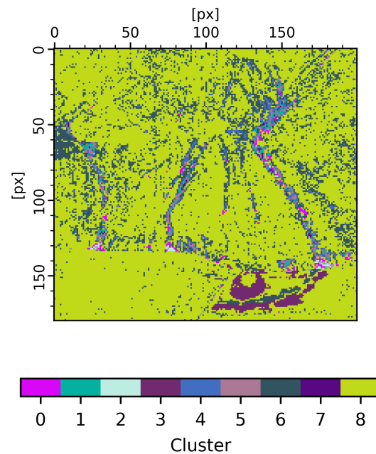
Abb. 6.16.: Räumliche Darstellung des Segmentierungsergebnis im limitierten Bereich für k=9 .
