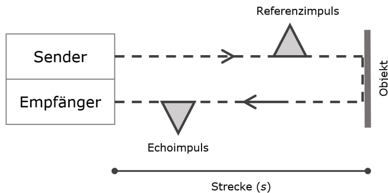
Abb. 2.6.: Grafische Darstellung des Impulslaufzeitverfahrens analog zur Gleichung 2.4.
