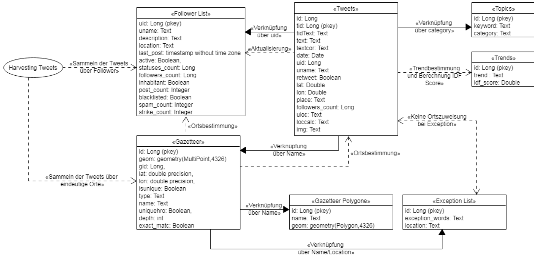
Abbildung 6-3: Datenbankstruktur.
