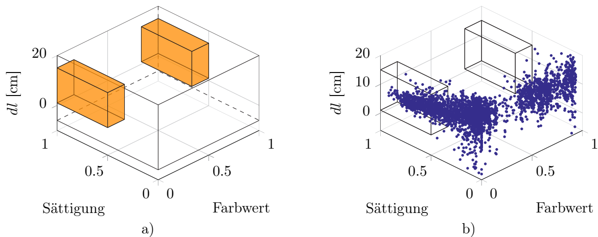
Abbildung 4.8: HSD-Merkmalsraum (Sättigung, Farbwert, Punktdistanz), a) orangener Bereich zeigt den Annahmebereich für Schalung, b) Verteilung für ein reales Schalungsteil
