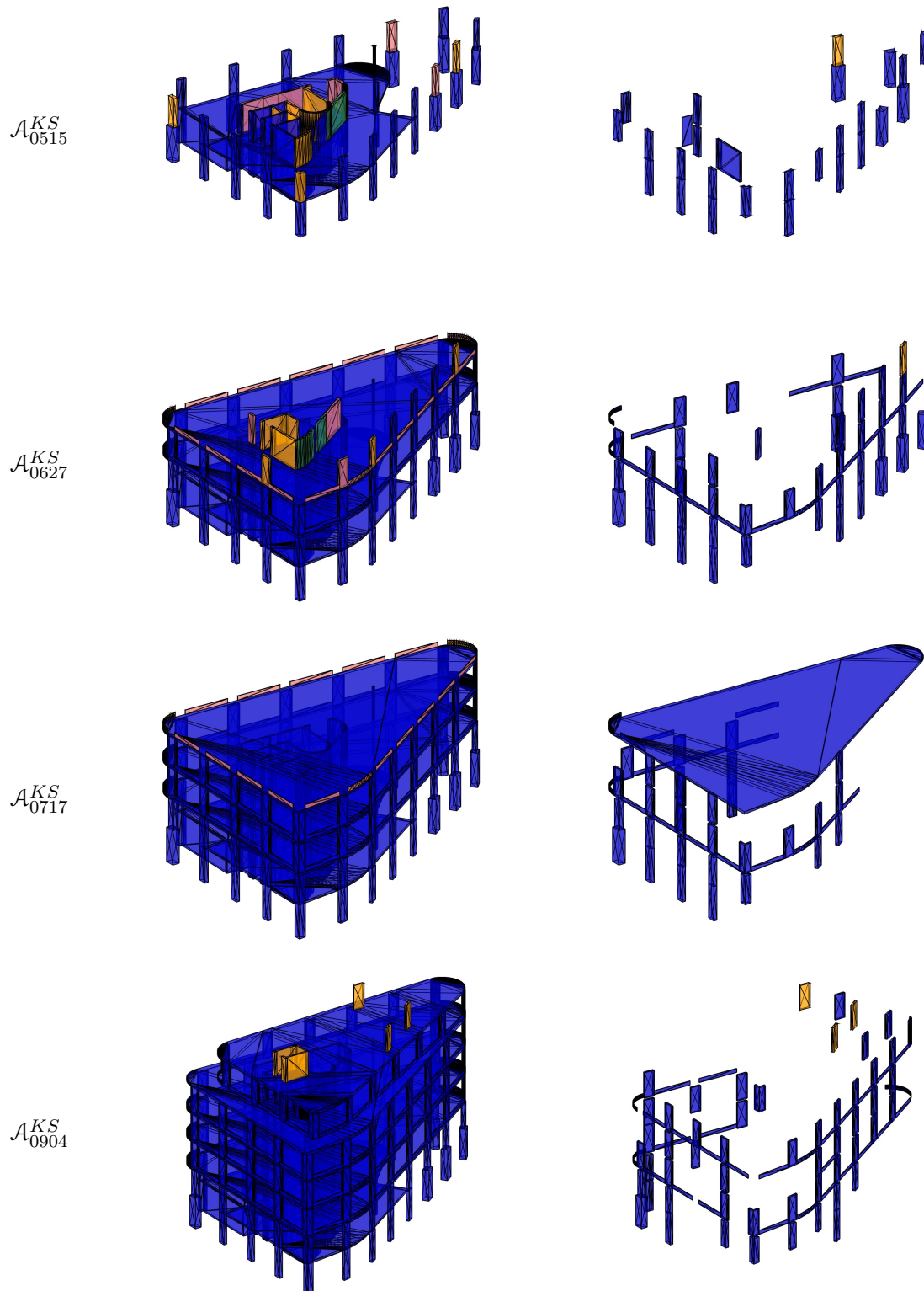
Abbildung 6.8: Ergebnis der Bauteilerkennung bei \mathcal{T}^{KS} , Auswahl von 4 Aufnahmeperspektiven, links Ground Truth \mathcal{G}_V ohne Bauteile mit dem Zustand nicht gebaut , rechts Klassifikationsergebnis ohne die Bauteile mit dem Zustand nicht gebaut , unbekannt und unsicher . Gezeigt sind die Klassen gebaut in blau, Schalung in orange, Bewehrung in korallenrot, Schalung und gebaut in magenta und Schalung und Bewehrung in grün. Die Farbgebung ist auch in Tabelle 4.1 aufgeschlüsselt.
