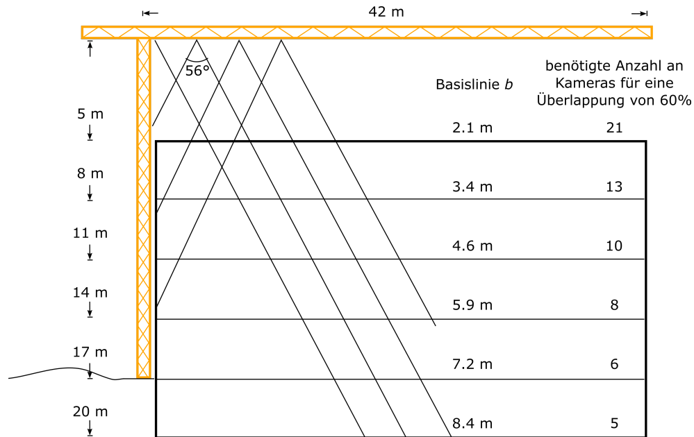
Abbildung 3.4: Seitenansicht der Aufnahmegeometrie von Krankameras: Schematische Darstellung für die Abdeckung verschiedener Gebäudehöhen durch Krankameras. Die für eine Überlappung q_Q von 60 % notwendige Anzahl an Kameras sowie der daraus resultierende Abstand entlang der Auslegerachse sind für verschiedene Gebäudehöhen in der Zeichnung angegeben.
