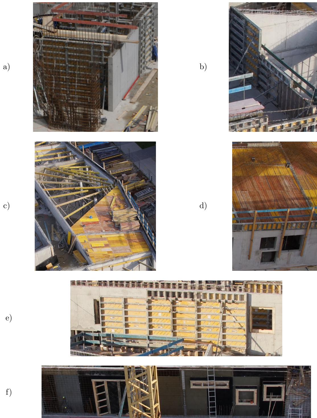
Abbildung 5.15: Beispiel für verschiedene spezielle Bauteilzustände: a) vorne Bewehrung, dahinter Schalung, rechts gebaut mit noch teilweise vorhandener Schalung, b) einseitig angebrachte Schalung, c) Deckenschalung, teilweise vorhanden, d) Deckenschalung und Bewehrung, e) gebaut mit teilweise vorhandener Schalung, f) Bewehrung und einseitig angebrachte Schalung
