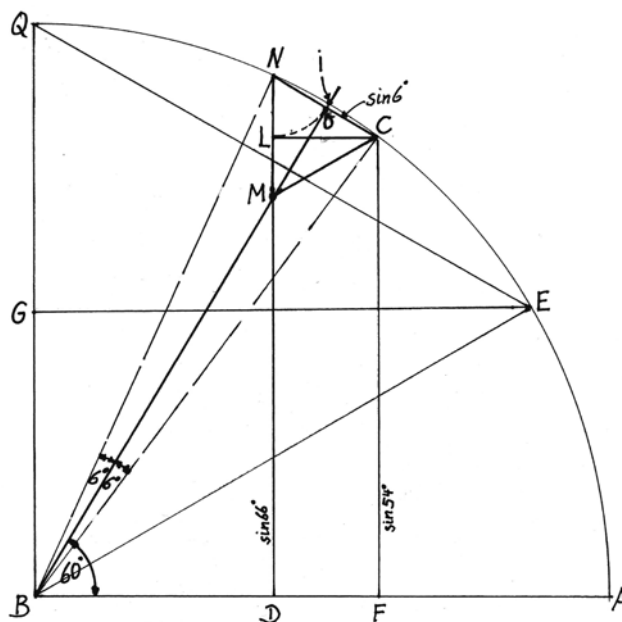
Abb. 64: Korrigierte Zeichnung zu Bürgis Blatt 42v.
