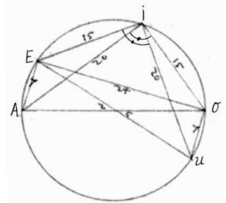
Abb. 28: Blatt 25r. Es handelt sich um dieselbe Zeichnung wie auf Blatt 24r, mit Ergänzung eines Kreisdurchmessers e u.
