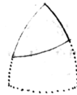
Abb. 94: Blatt 74r: Zu 1. und 2.
