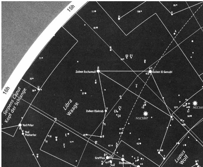
Abb. 21: Sternbild Libra-Waage, mit \beta Lib = Lanx borealis.
