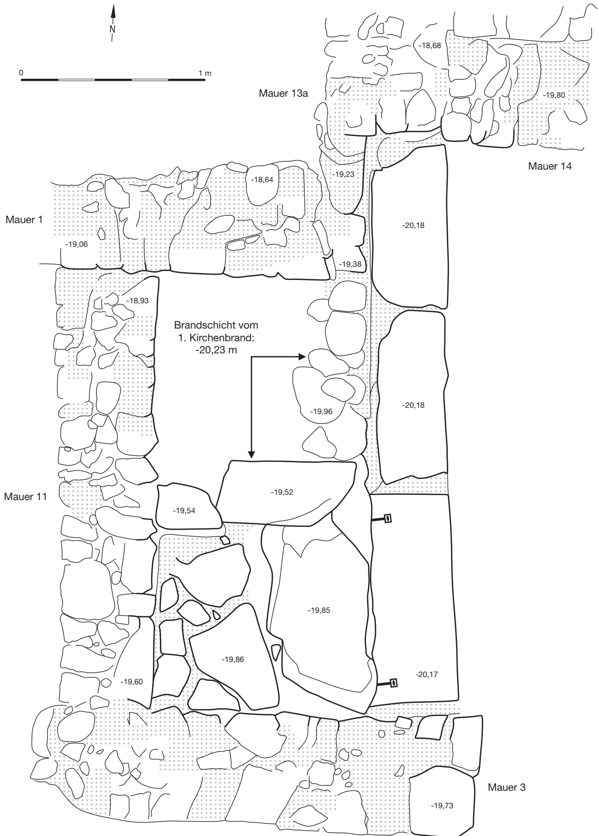
Abb. 22. Detailzeichnung der Marmorblöcke und des Treppenaufgangs (Periode 2b). Eingetragen im nördlichen Teil des nur in Resten erhaltenen Treppenaufgangs (Beil. 9) die Brandschicht vom ersten Kirchenbrand. – M. 1:20.
