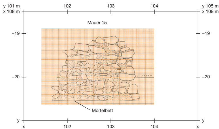
Abb. 30. Detailansicht Mauer 15 (Querannex). – M. 1:50.
