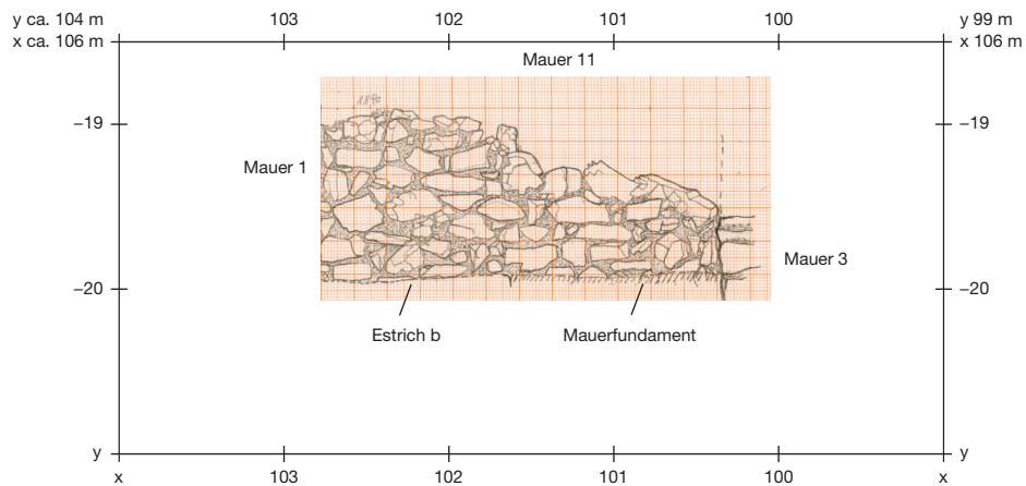
Abb. 28. Detailansicht Mauer 11, von Westen. – M. 1:50.
