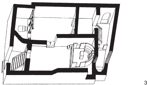
Abb. 39. Säben, Hl.-Kreuz: 1 Grabungsbefund, 2-3 rekonstruierter Grundriss und perspektivische Rekonstruktion nach F. Glaser – M. 1:400.
