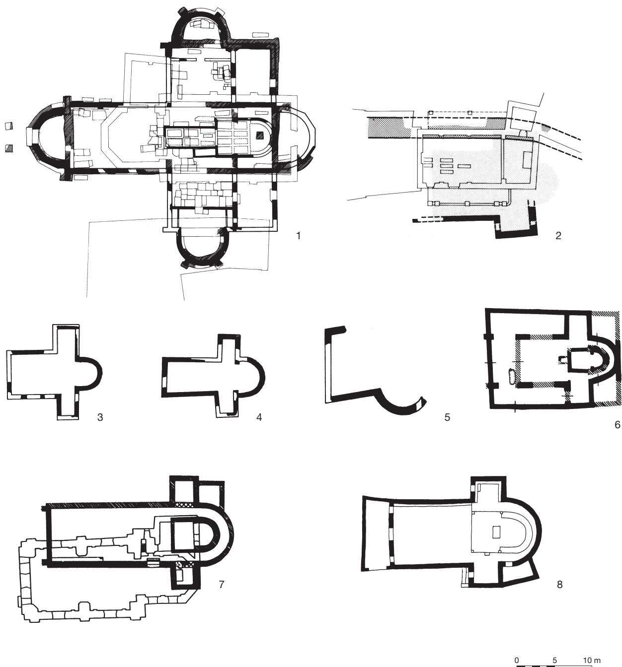
Abb. 37. 1 Aosta, S. Lorenzo; 2 Solothurn, St. Stephan; 3 Wimmis; 4 Zurzach, St. Verena I; 5 Chur, Kathedrale I; 6 Altenburg, St. Peter; 7 Lavant, St. Ulrich; 8 Teurnia , Bischofskirche I – M. 1:500.
