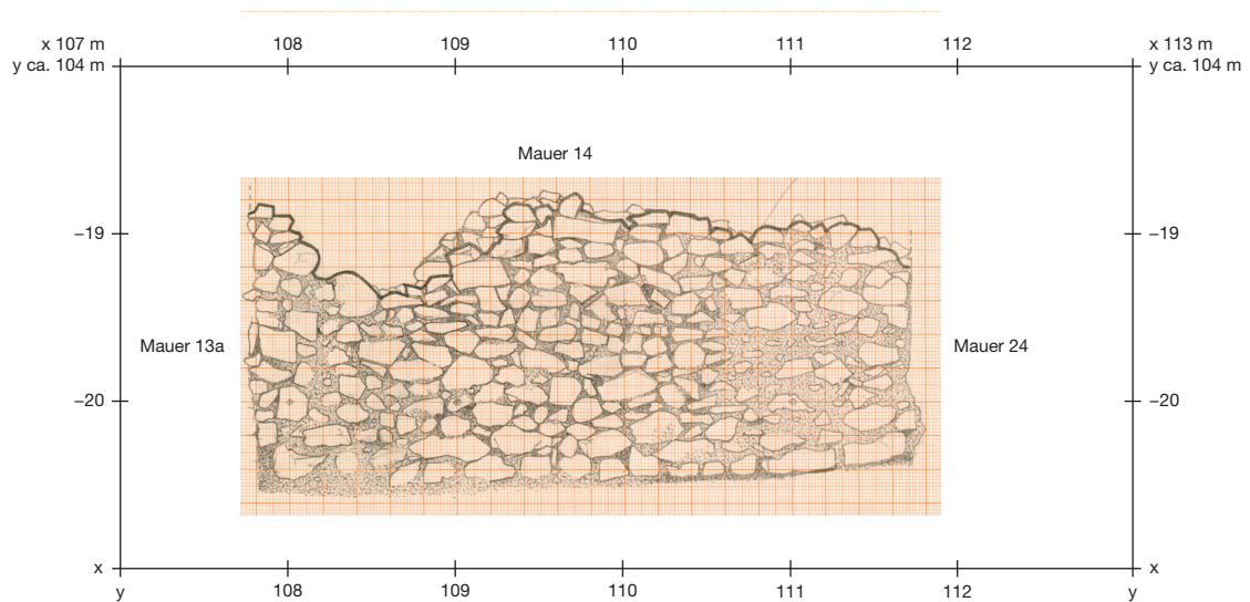
Abb. 29. Detailansicht Mauer 14, von Süden. – M. 1:50.
