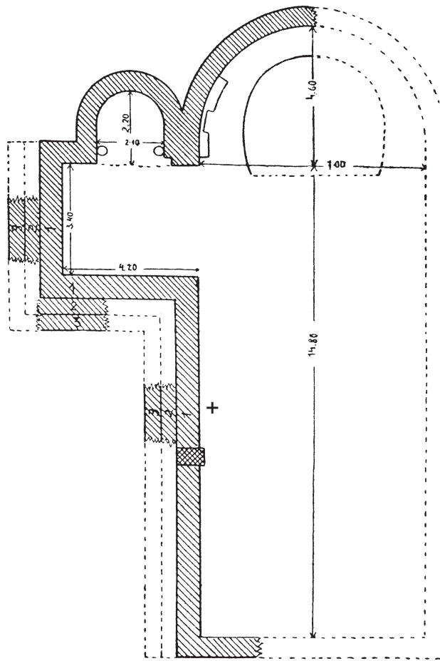
Abb. 9. Kirche am Hang: Ausgrabung A. Egger. – M. 1:150.
