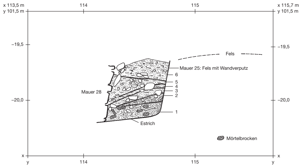
Abb. 19. Profil 18 (Grabungsprofil 328). – M. 1:20.
