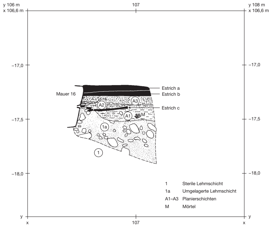
Abb. 23. Profil 14 (Grabungsprofil 303). – M. 1:20.
