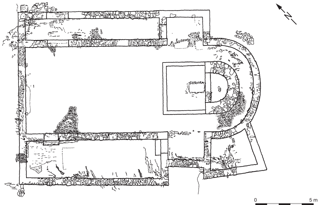
Abb. 45. Kirche vom Ducl. – M. 1:200.
