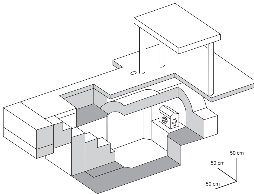
Abb. 21. Rekonstruktionszeichnung der Reliquienkammer von Säben (nach Glaser 1997d).
