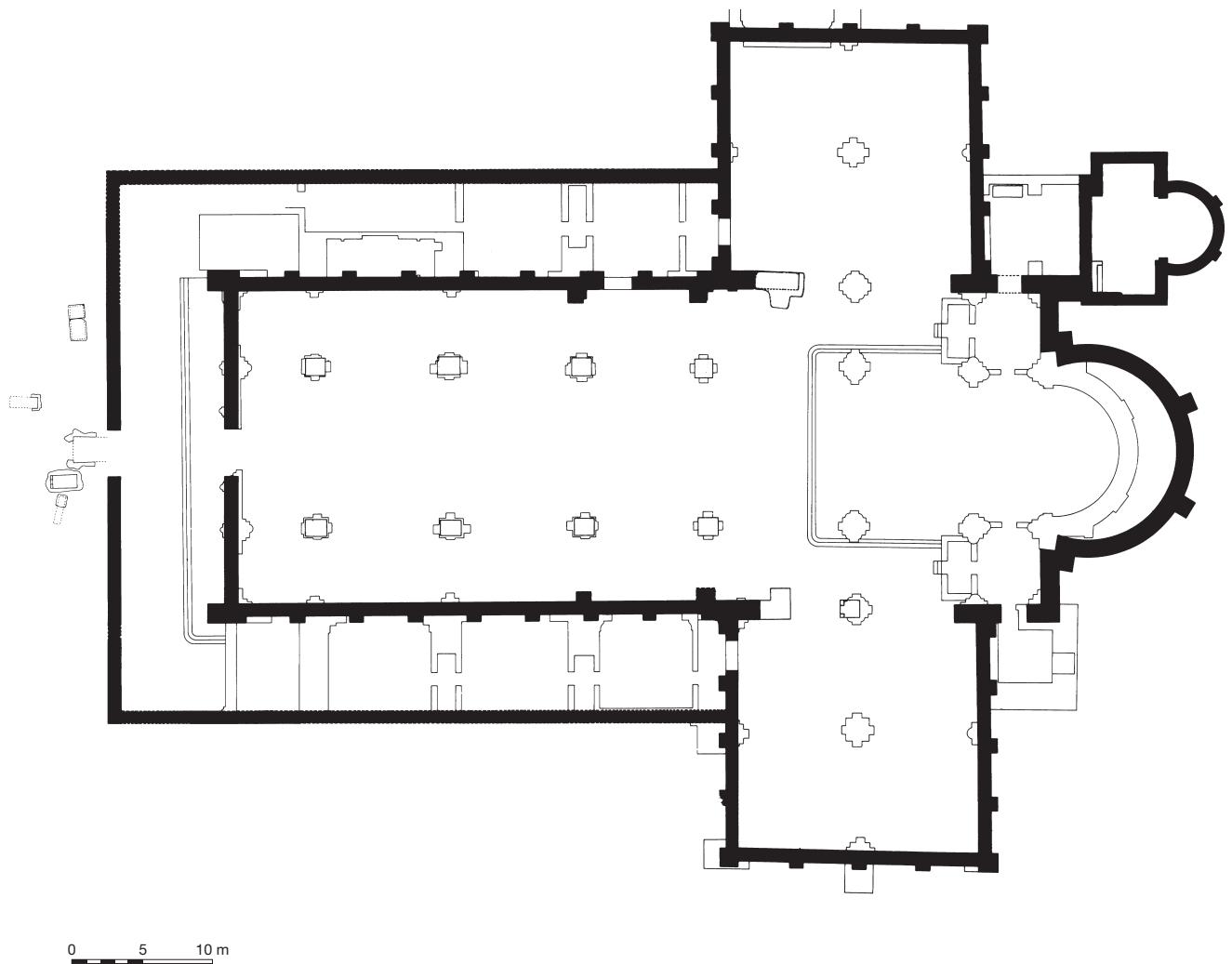
Abb. 34. Mailand, S. Simpliciano – M. 1:500.
