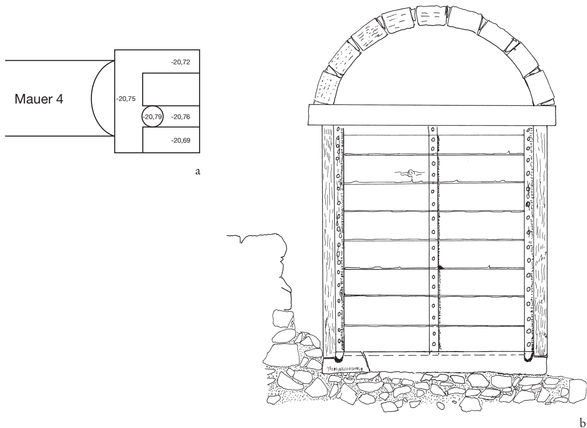
Abb. 17. a Türangelstein von der Tür in das Kirchenschiff: Idealisierte Umzeichnung (Skizze) nach Grabungstagebuch (Journal) IX 47; b Rekonstruktion der Tür in das Kirchenschiff (Zeichnung: H. Nothdurfter).
