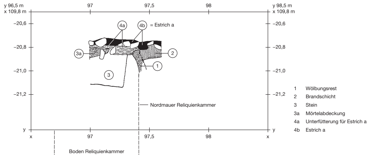
Abb. 20. Profil 17 (Grabungsprofil 404). – M. 1:20.
