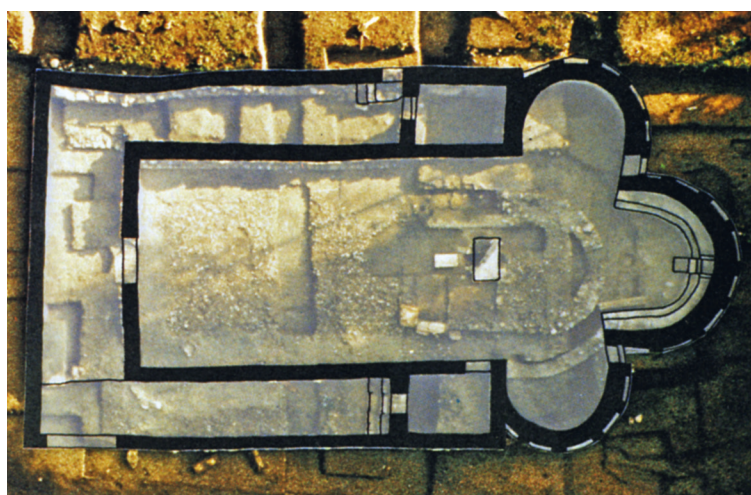
Abb. 44. 1 Invillino, Colle di Zuca, spätantike Kirchenanlage; Teurnia , Bischofskirche: 2 ältere Periode, 3 jüngere Periode. – M. 1:300.
