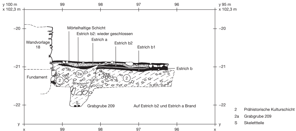
Abb. 18. Profil 8 (Grabungsprofil 555). – M. 1:50.
