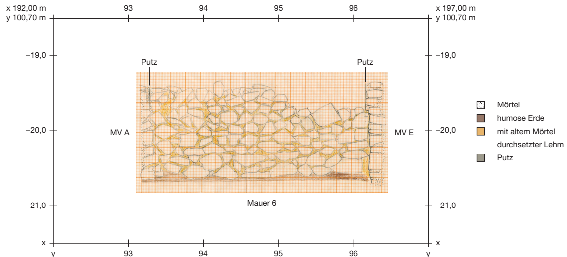
Abb. 31. Detailansicht Mauer 6. – M. 1:50.
