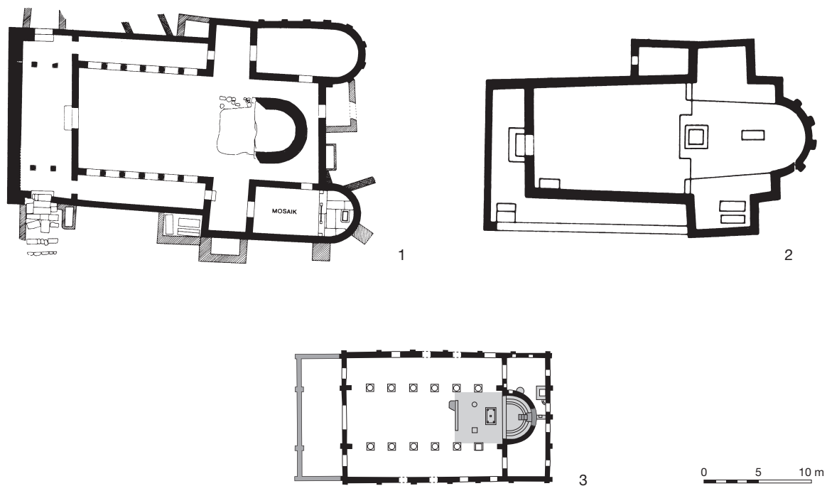
Abb. 38. 1 Teurnia , extra muros; 2 Hemmaberg, Kirche O; 3 Grado, S. Maria – M. 1:500.
