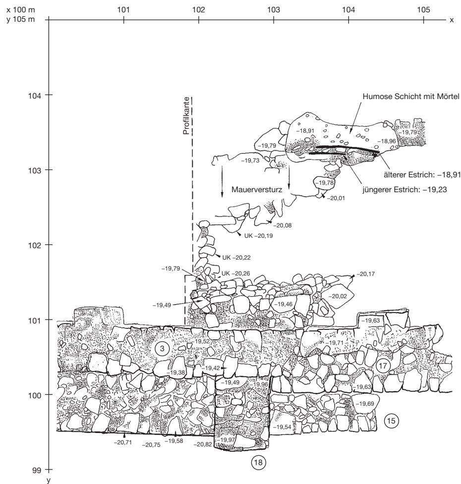
Abb. 24. Detailzeichnung der verstürzten Mauerteile und der Estriche von Mauer 16 im Längsannex. M. 1:50.
