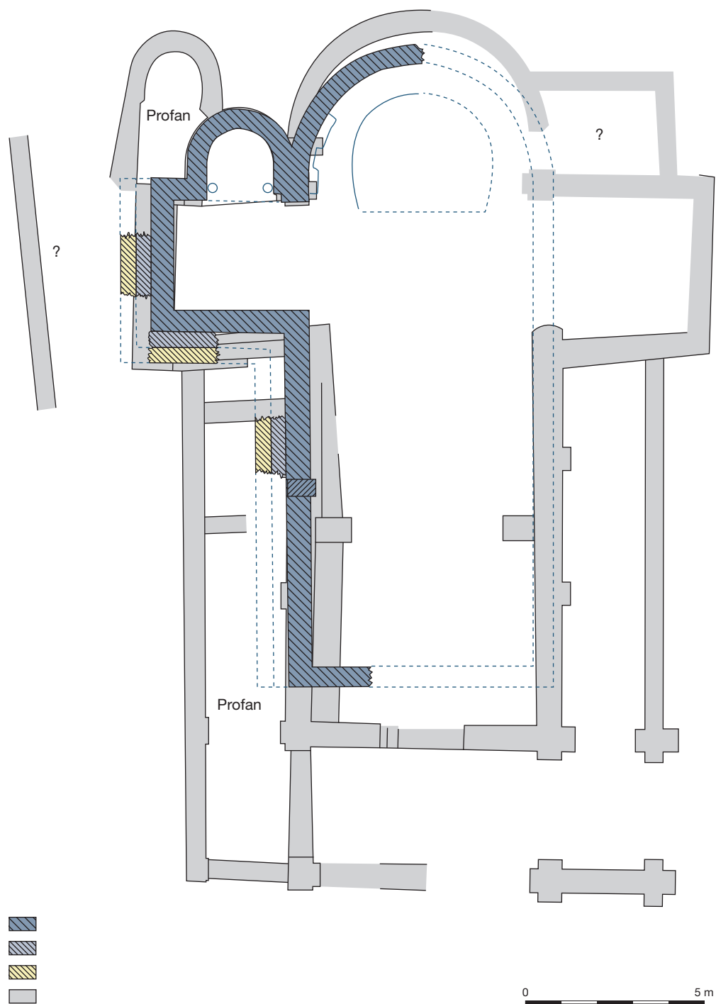
Abb. 11. Kirche am Hang; vergleichende Zusammenzeichnung der Grabungsbefunde von A. Egger (dunkelblau, hellblau, gelb; vgl. Abb. 9) mit den Grabungsergebnissen von 1978 bis 1982 (grau; ohne Periodentrennung). M. 1:150.
