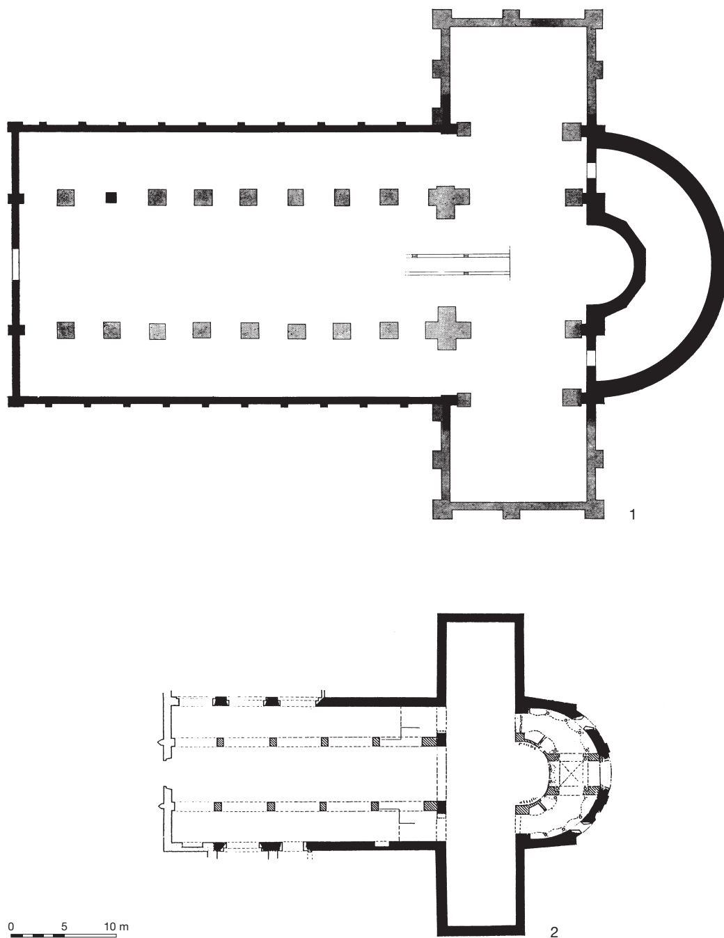
Abb. 36. 1 Aquileia, Basilica del fondo Tullio; 2 Verona, S. Stefano – M. 1:500.
