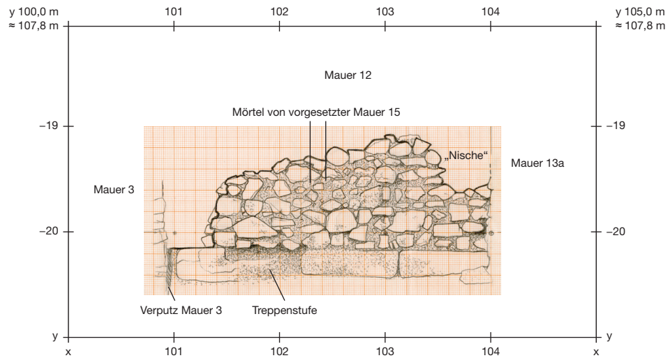
Abb. 27. Detailansicht Mauer 12, von Westen. – M. 1:50.
