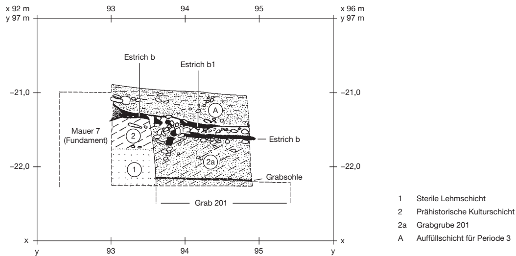
Abb. 15. Profil 20 (Grabungsprofil 510). – M. 1:50.
