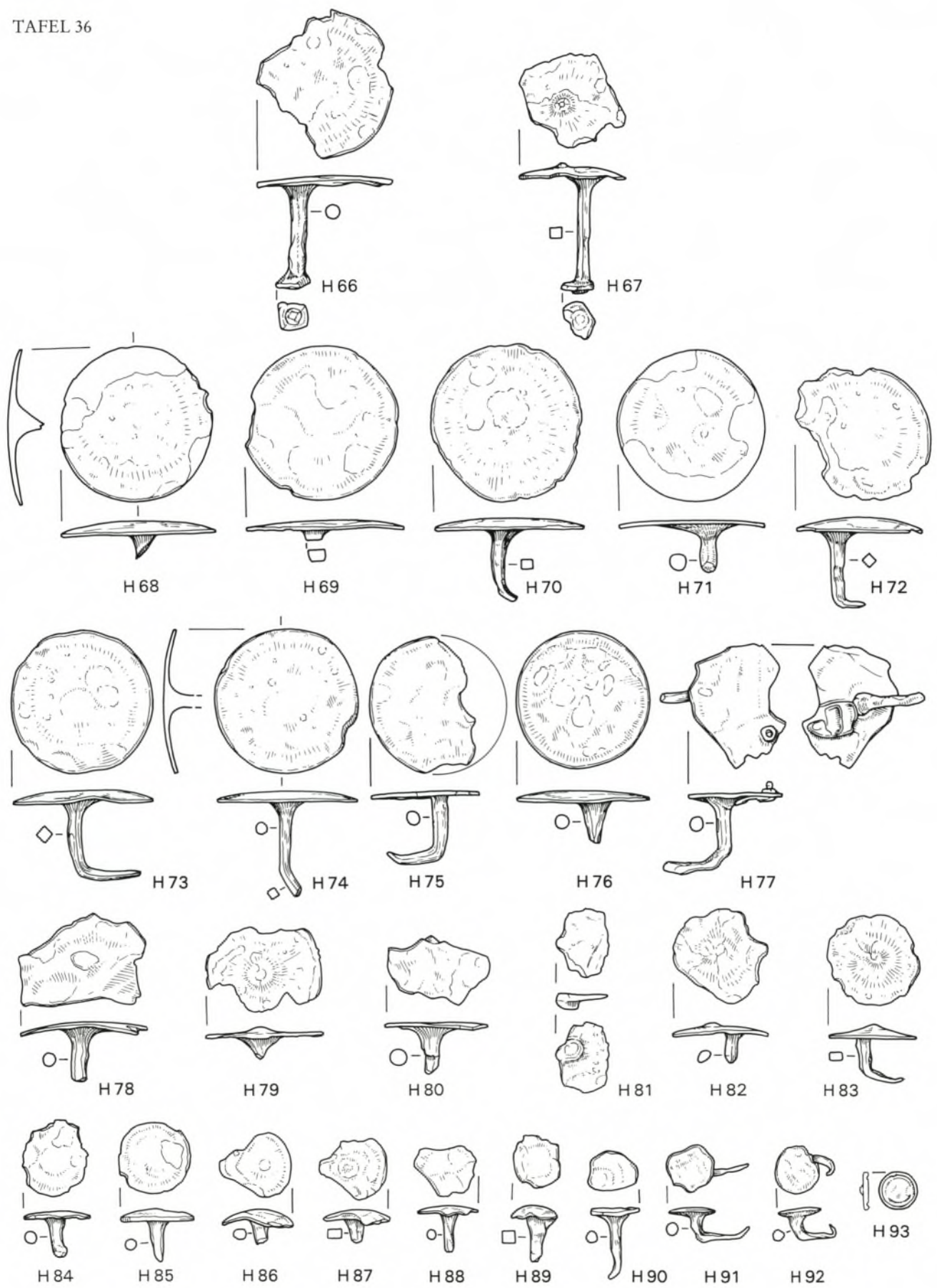
Brandopferplatz Forggensee. – H66–93 Nägel. – Eisen. – M. 1:2.
