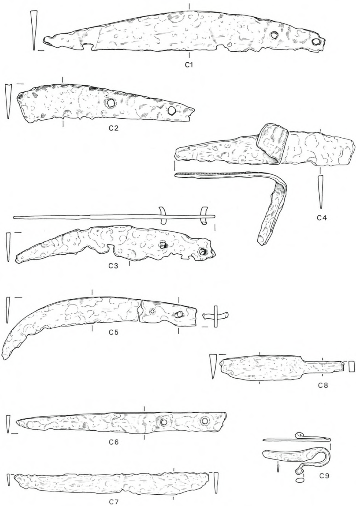
Brandopferplatz Forggensee. – C1–9 Messer. – Eisen. – M. 1:2.
