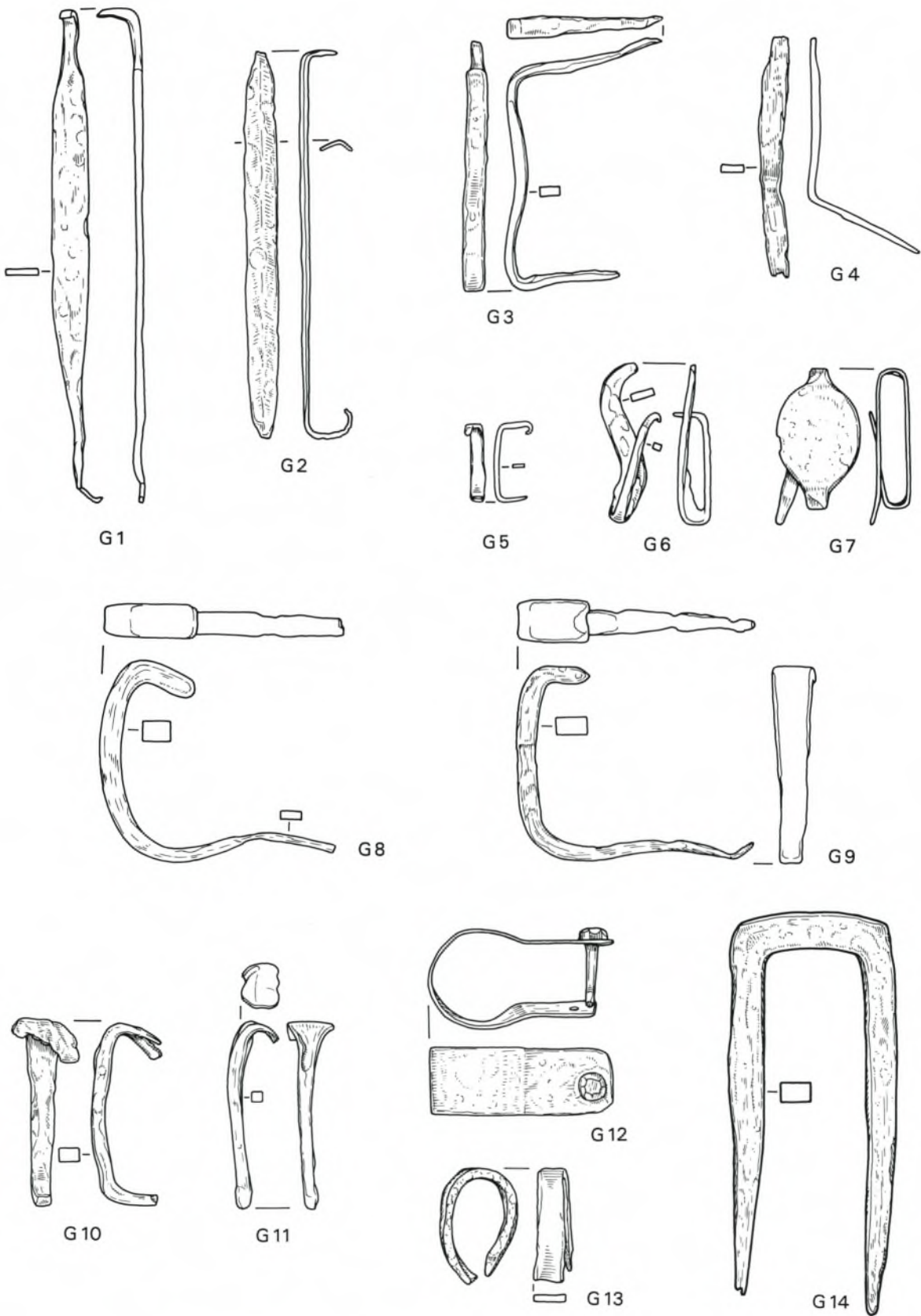
Brandopferplatz Forggensee. – G1–14 Bau- und Verbindungselemente. – Eisen. – M. 1:2.
