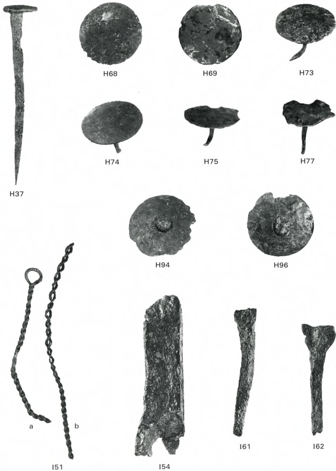
Brandopferplatz Forggensee. – H37–96 Nägel; I51–62 Sonstiges. – Eisen. – M. 1:2.
