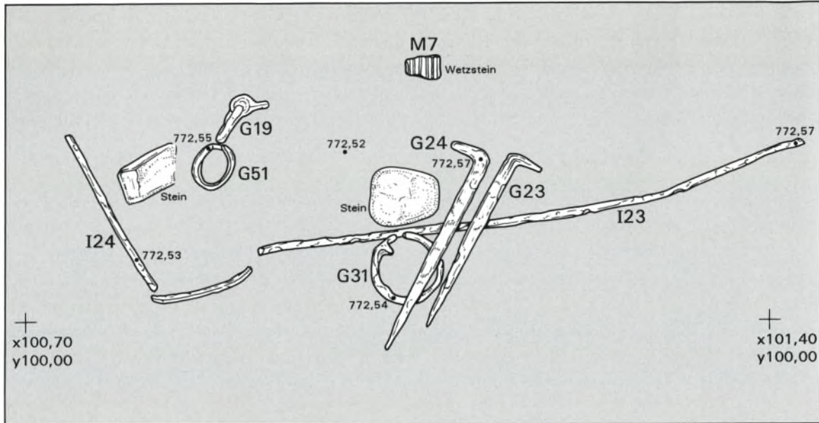
Abb. 7. Brandopferplatz im Forggensee. Eisendepot westlich der Opferstelle 1; Lage der in situ geborgenen Gegenstände mit Angabe der Katalognummern. – M. 1:5.
