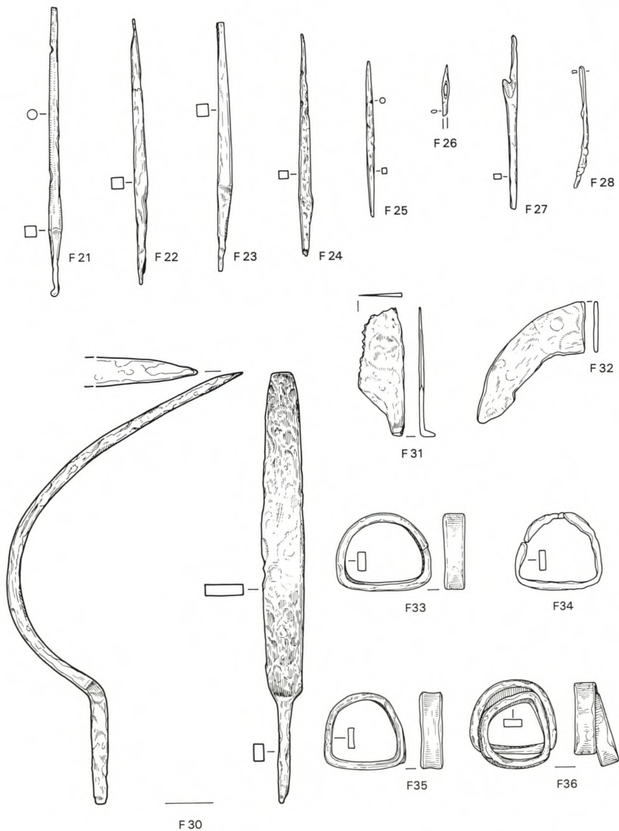
Brandopferplatz Forggensee. – F21–36 Werkzeuge und Geräte. – Eisen. – M: 1:2.
