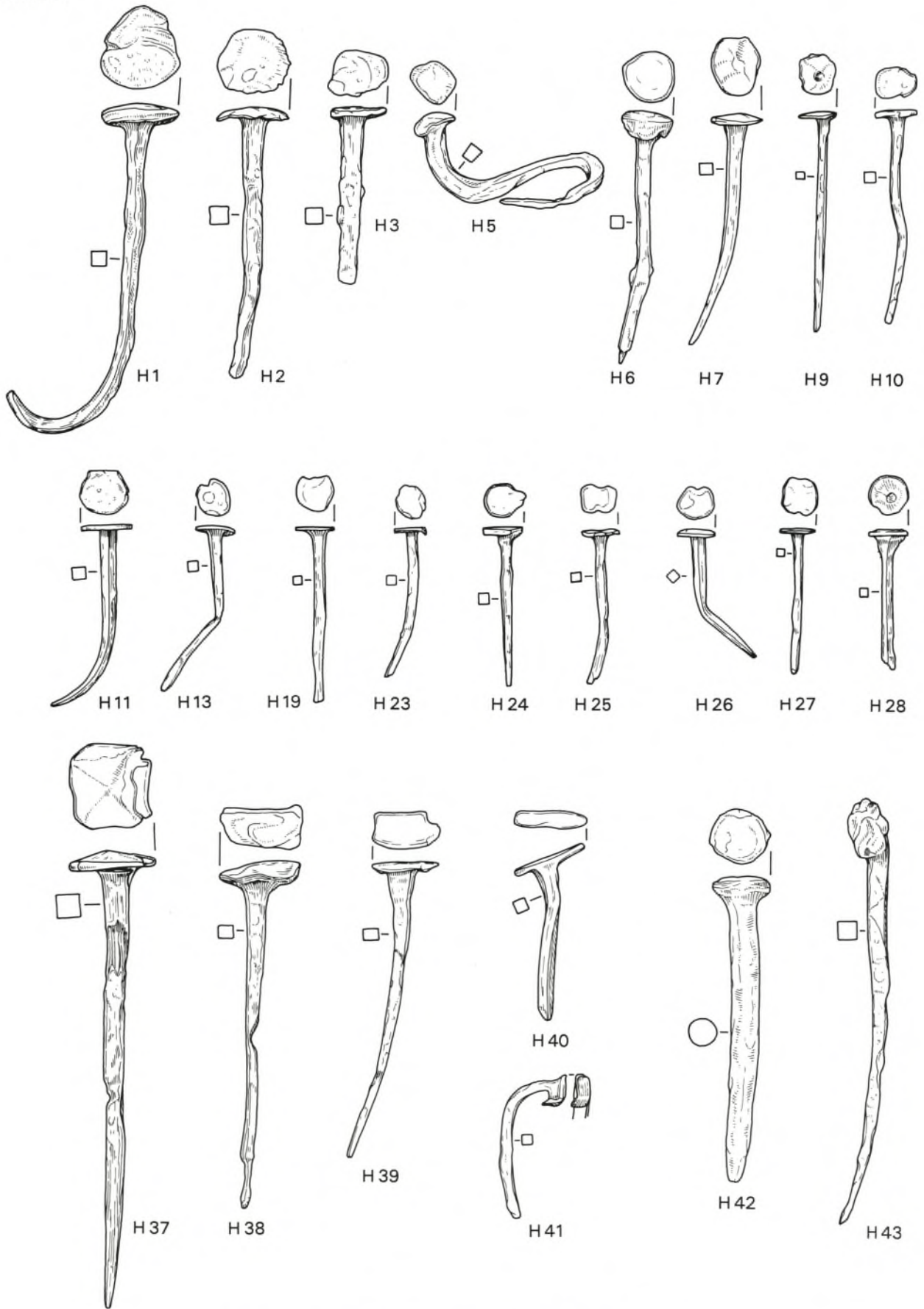
Brandopferplatz Forggensee. – H1–43 Nägel. – Eisen. – M. 1:2.
