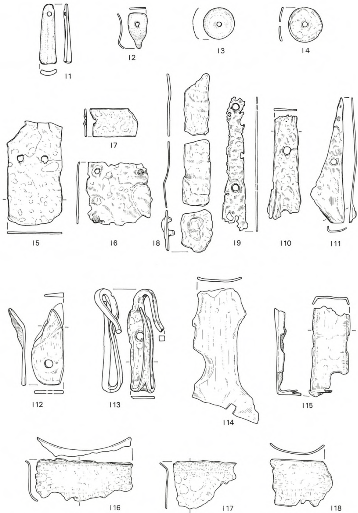
Brandopferplatz Forggensee. – I1–18 Sonstiges. – I1–3 Bronze; I4–18 Eisen. – M. 1:2.
