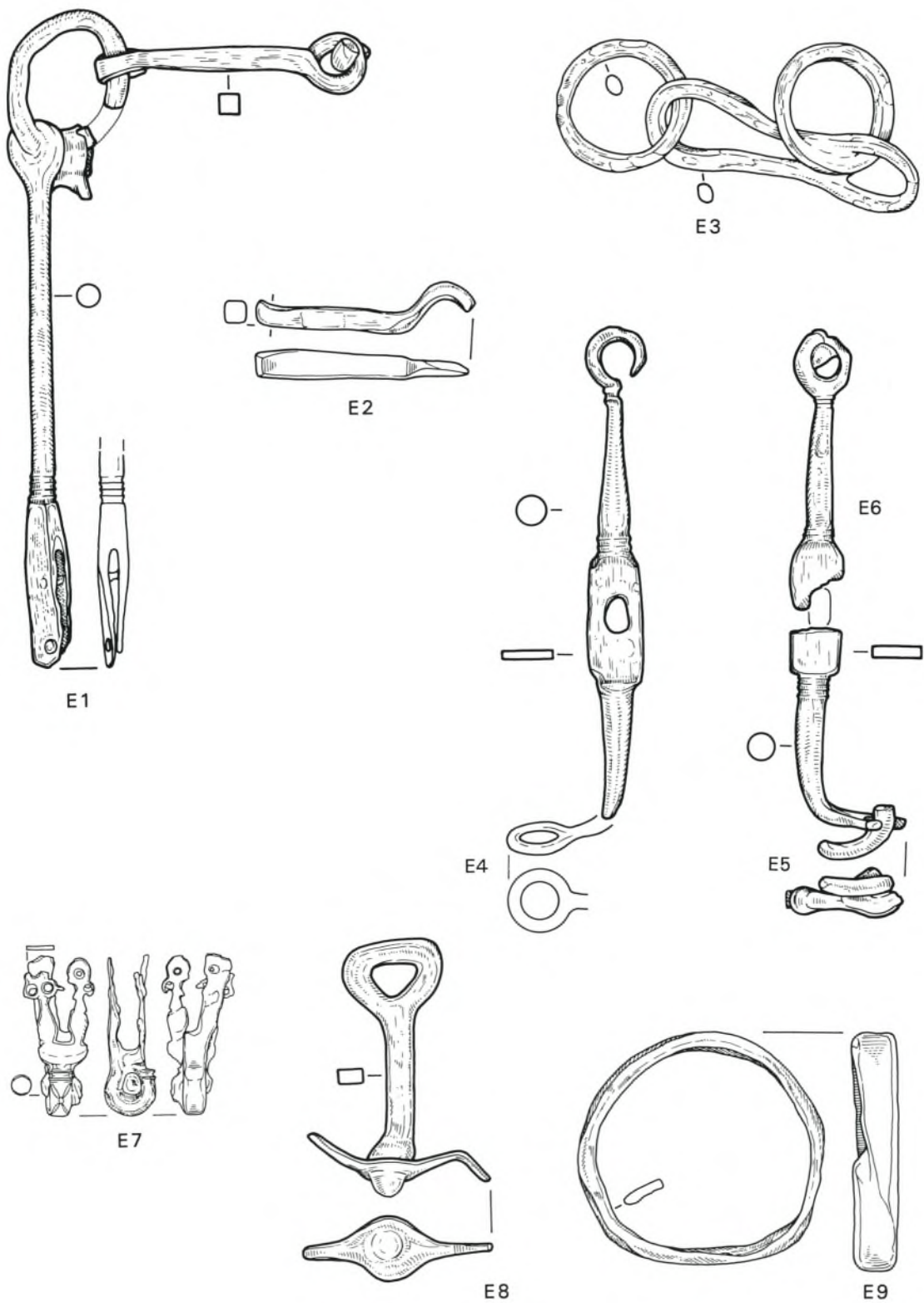
Brandopferplatz Forggensee. – E1–9 Pferdegeschirr- und Wagenteile. – Eisen; E8 Eisen und Bronze. – M. 1:2.
