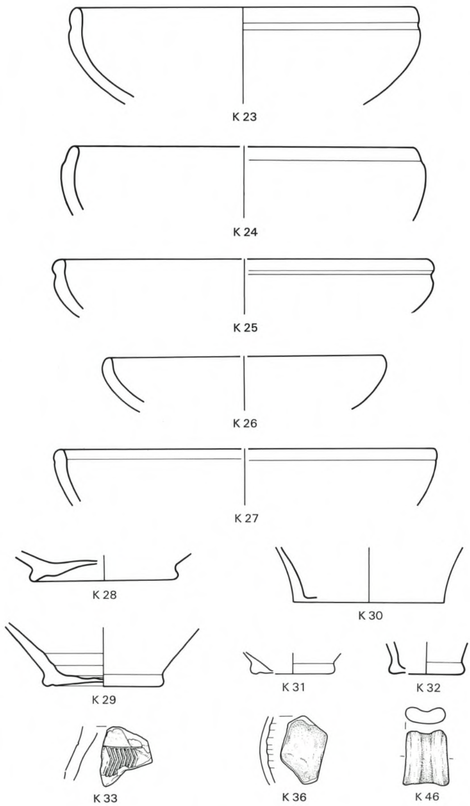
Brandopferplatz Forggensee. – K23–46 Keramik. – M: 1:2.
