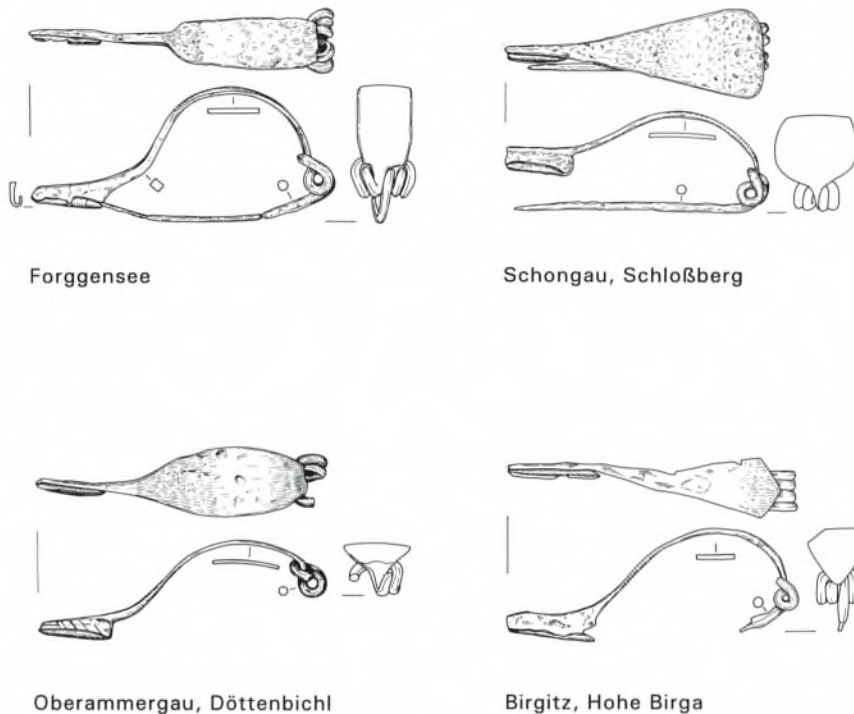
Abb. 11. Große spätlatènezeitliche Eisenfibeln vom Forggensee (Katalog B7), vom Schloßberg bei Schongau (vgl. Anm. 83), von der Hohen Birga bei Birgitz im Inntal (Gleirscher, Hohe Birga 343 Abb. 59, 12) und vom Döttenbichl bei Oberammergau. – M. 1:3.
