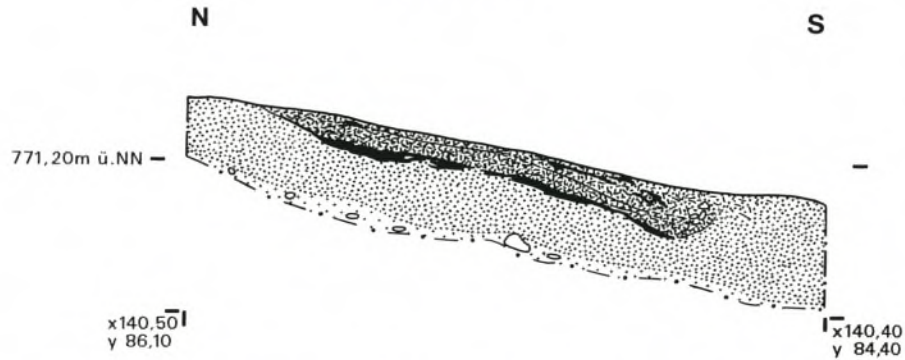
Abb. 9. Brandopferplatz im Forggensee. Ostprofil des Längsschnittes durch die Feuerstelle (14). – M. 1:20.
