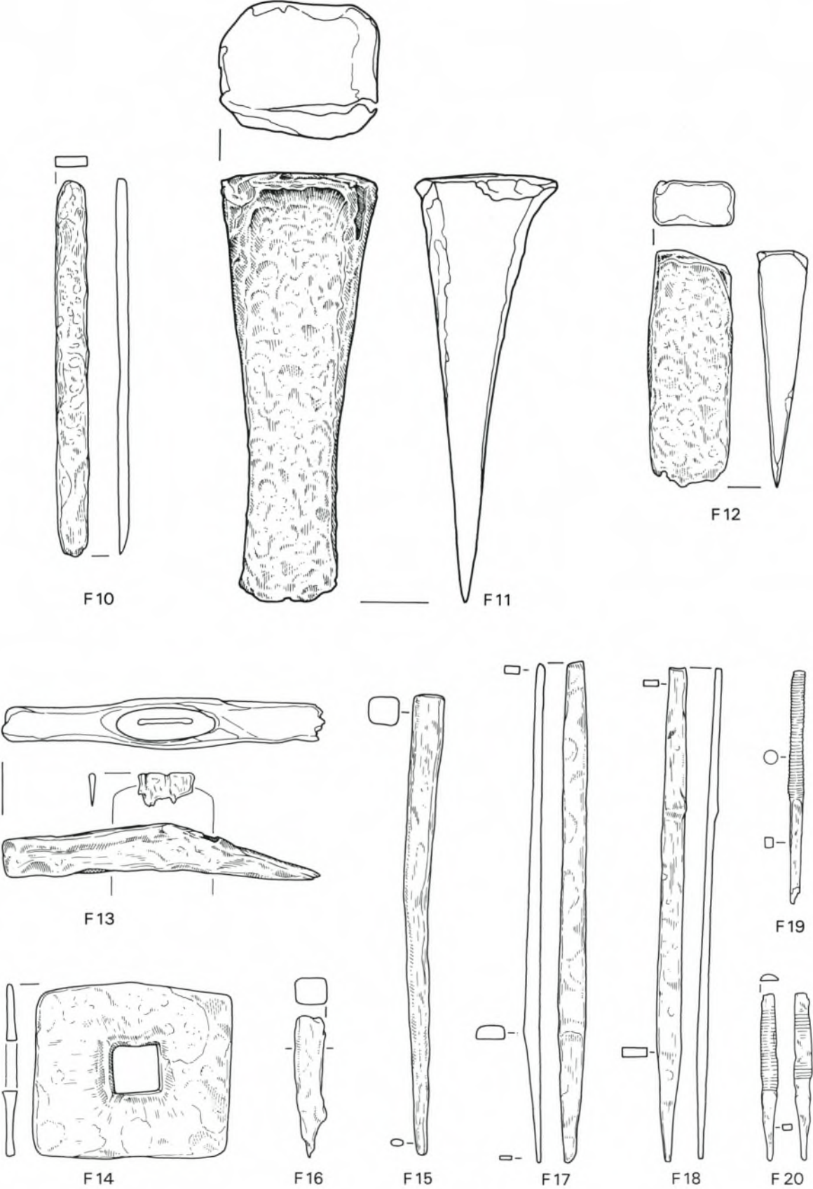
Brandopferplatz Forggensee. – F10–20 Werkzeuge und Geräte. – Eisen. – M. 1:2.
