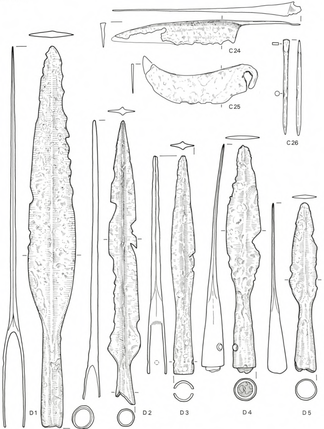
Brandopferplatz Forggensee. – C24.25 Toilettgerät; C26 Stilus; D1–5 Lanzenspitzen. – Eisen. – M. 1:2.
