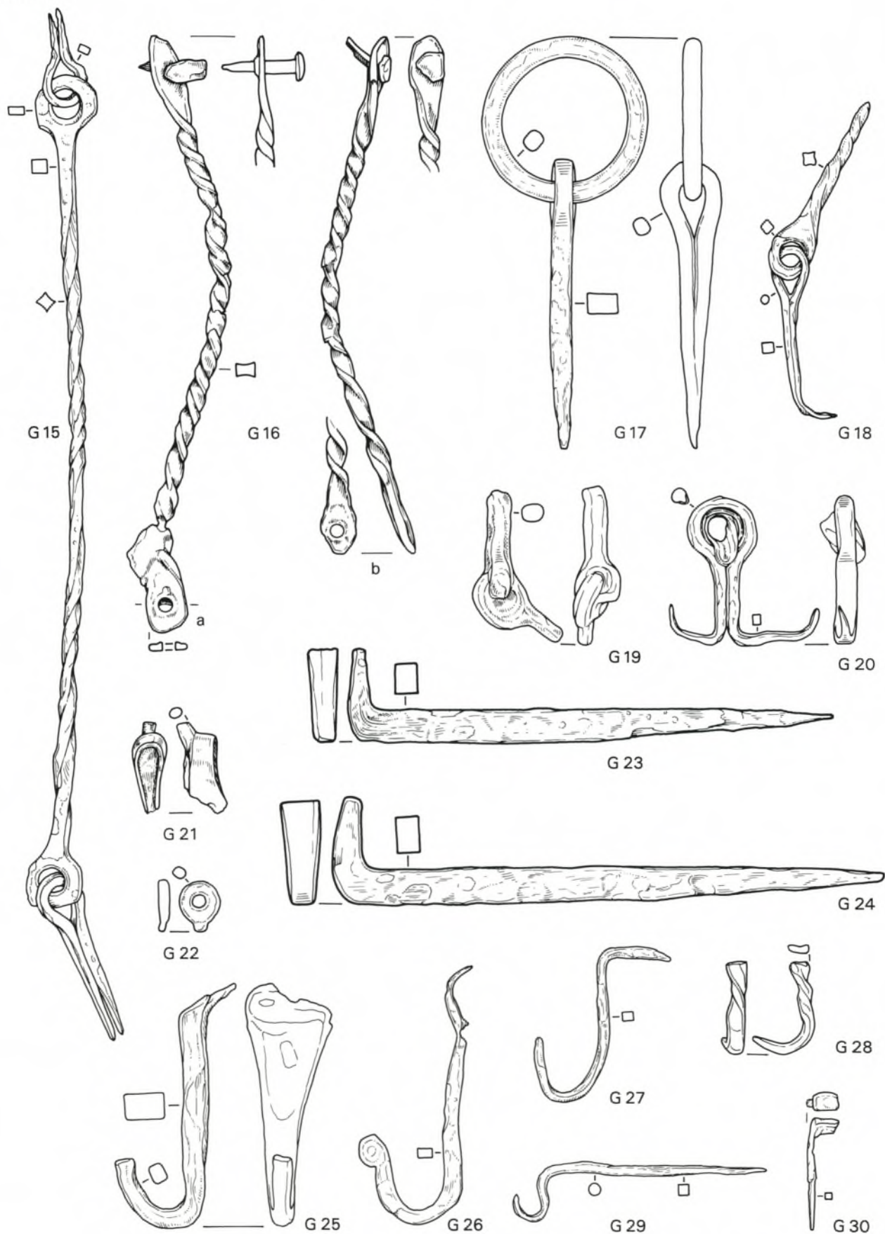
Brandopferplatz Forggensee. – G15–30 Bau- und Verbindungselemente. – Eisen. – M. 1:2.
