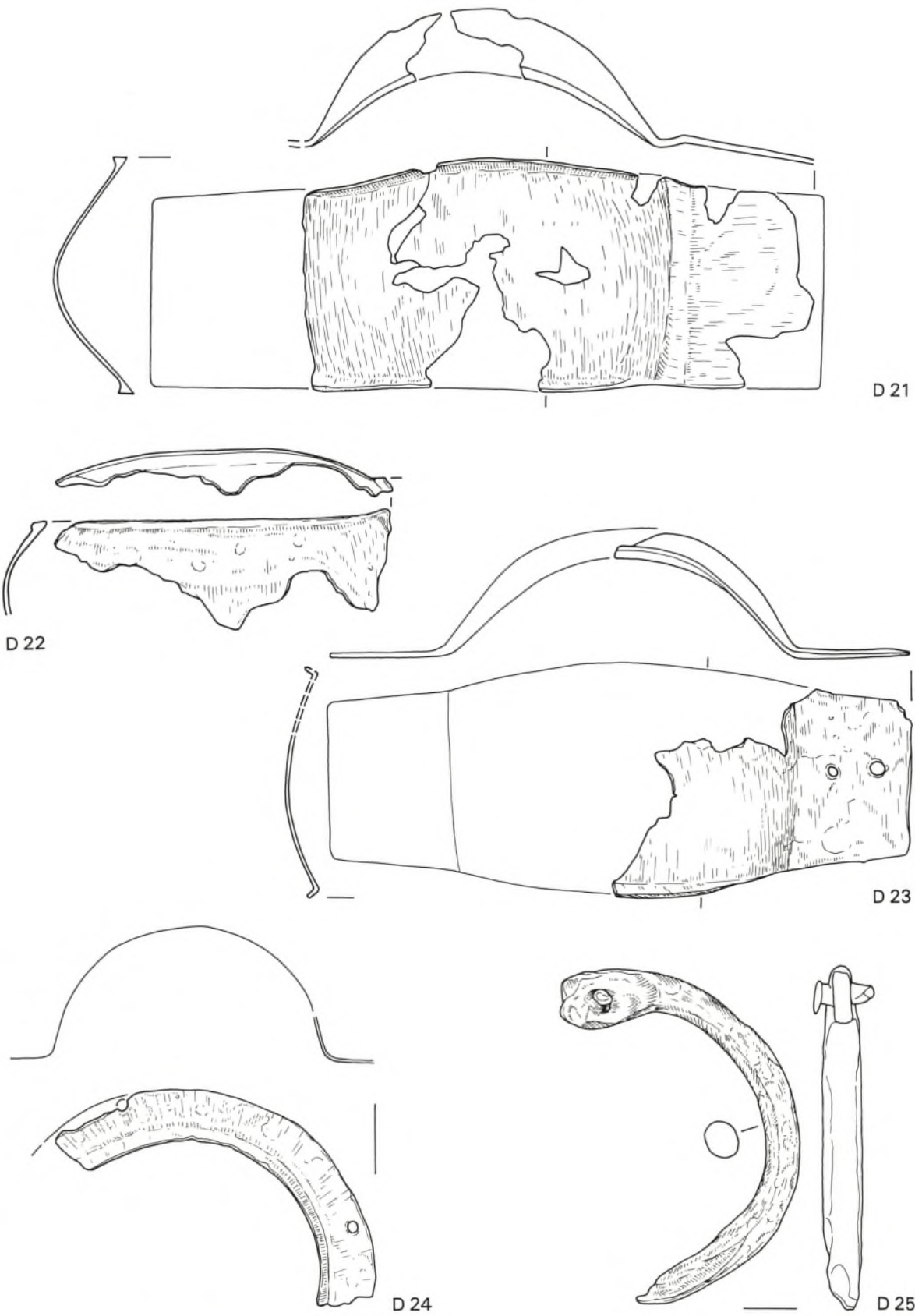
Brandopferplatz Forggensee. – D21–24 Schildbuckel; D25 Fessel (?). – Eisen. – M. 1:2.
