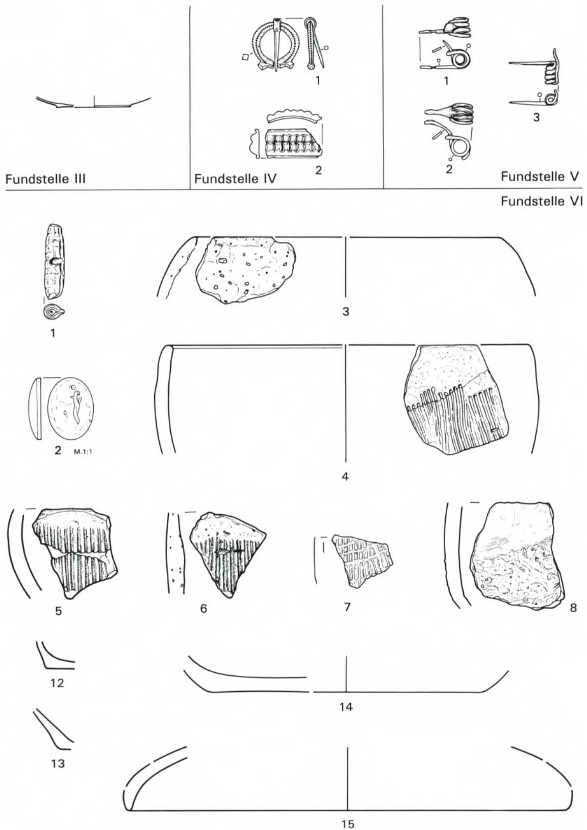
Abb. 31. Funde aus den Fundstellen III–VI nördlich des Brandopferplatzes im Forggensee. – M. 1:2.
