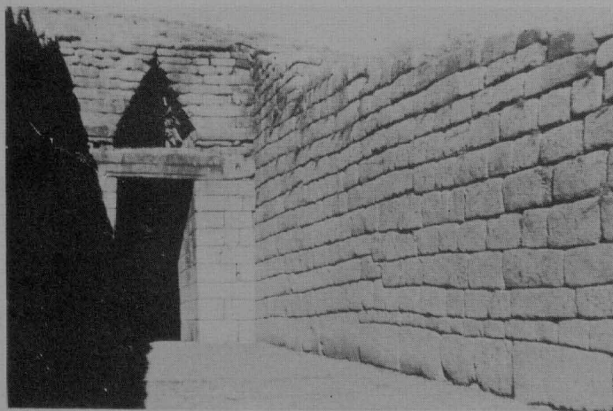
2. Abschluß des Gewölbes in der Firstlinie einer Steinhütte bei La Roque-sur-Perthes (Vaucluse), phot. Rohlf
