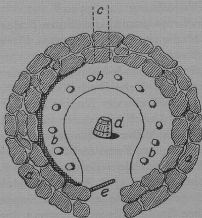
Fig. 1. Grundriß einer Hirtenhütte im Tal von Poschiavo, s. Anm. 27
