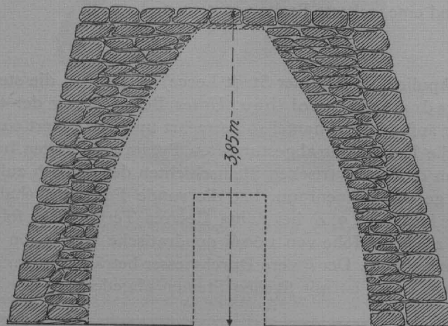
Fig. 4. Senkrechter Schnitt der gleichen Steinhütte aus der Umgegend von Santa Cesarea (Prov. Lecce)
