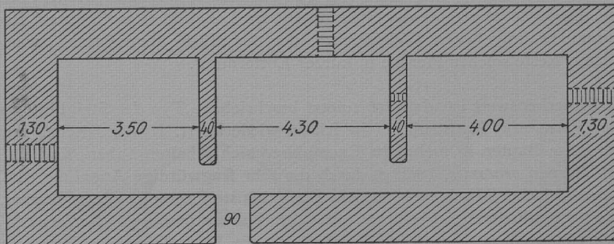
Fig. 14. Grundriß eines Monumentalbaues (s. Tafel 19, 1) bei La Roque-sur-Pernes (Vaucluse)
