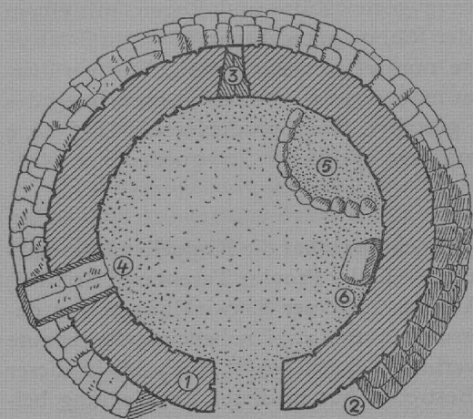
Fig. 6. Grundriß einer Rundhütte bei Dignano (Istrien), s. Anm. 53
