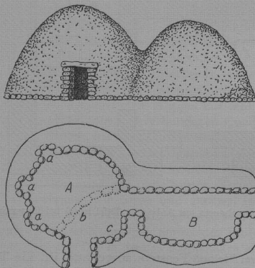
Fig. 10. Doppelhütte ( beehive house ) auf der Insel Lewis (Hebriden), s. Anm. 57
