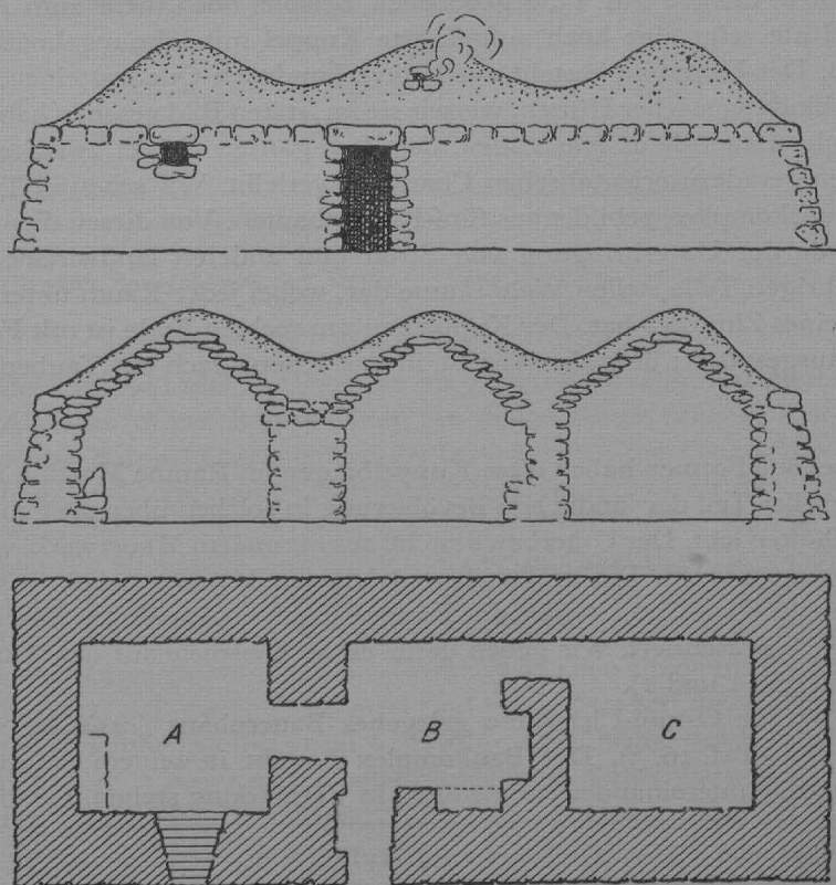
Fig. 8. Vorderansicht, Querschnitt und Grundriß eines Bauernhauses der Provinz Tarragona, s. Anm. 54
