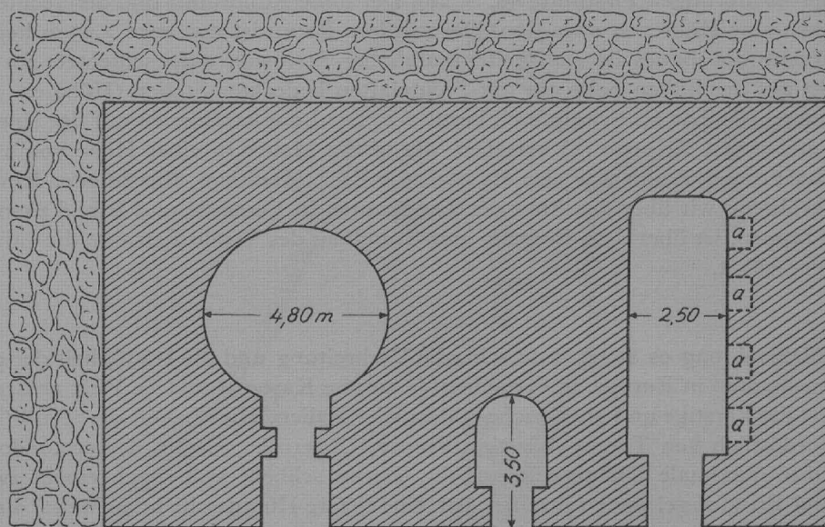
Fig. 15. Grundriß eines Gewölbekomplexes (s. Tafel 20, 4) bei Ruffano (Prov. Lecce)
