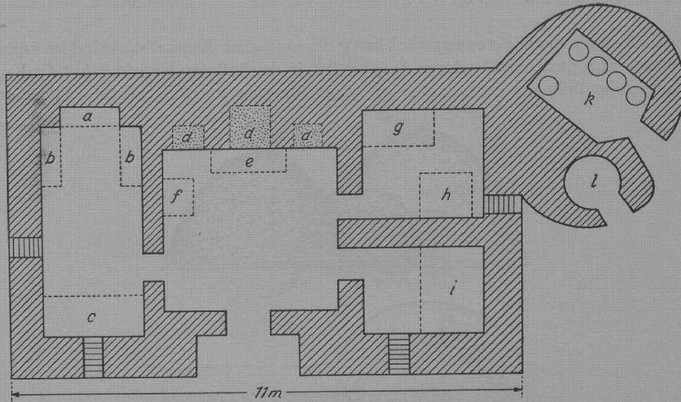
Fig. 9. Grundriß eines Bauernhauses mit Anbau (s. Tafel 16, 3) bei Cisternino in der Provinz Brindisi
