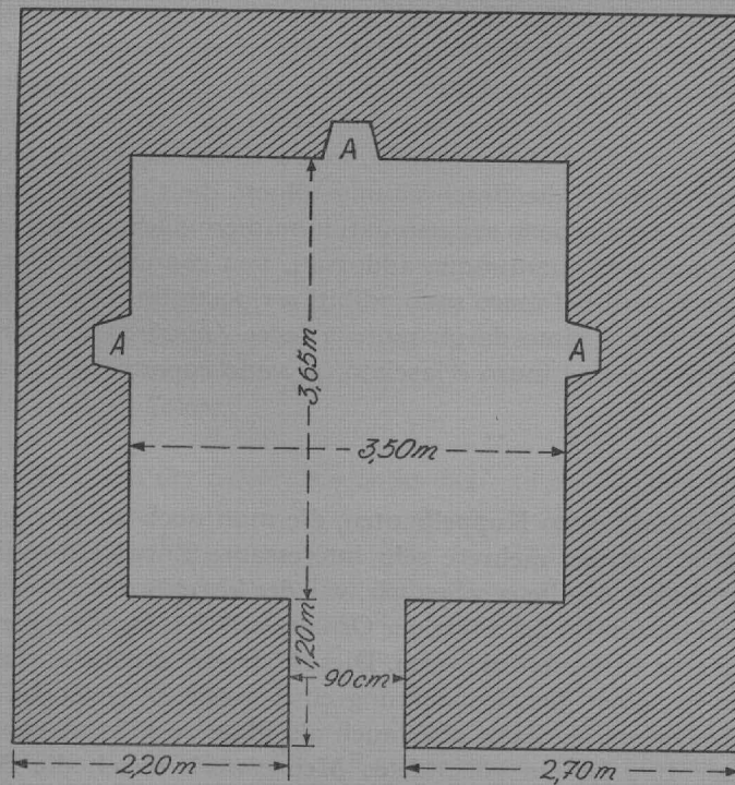
Fig. 3. Grundriß einer quadratischen Steinhütte aus der Umgegend von Santa Cesarea Terme (Prov. Lecce)
