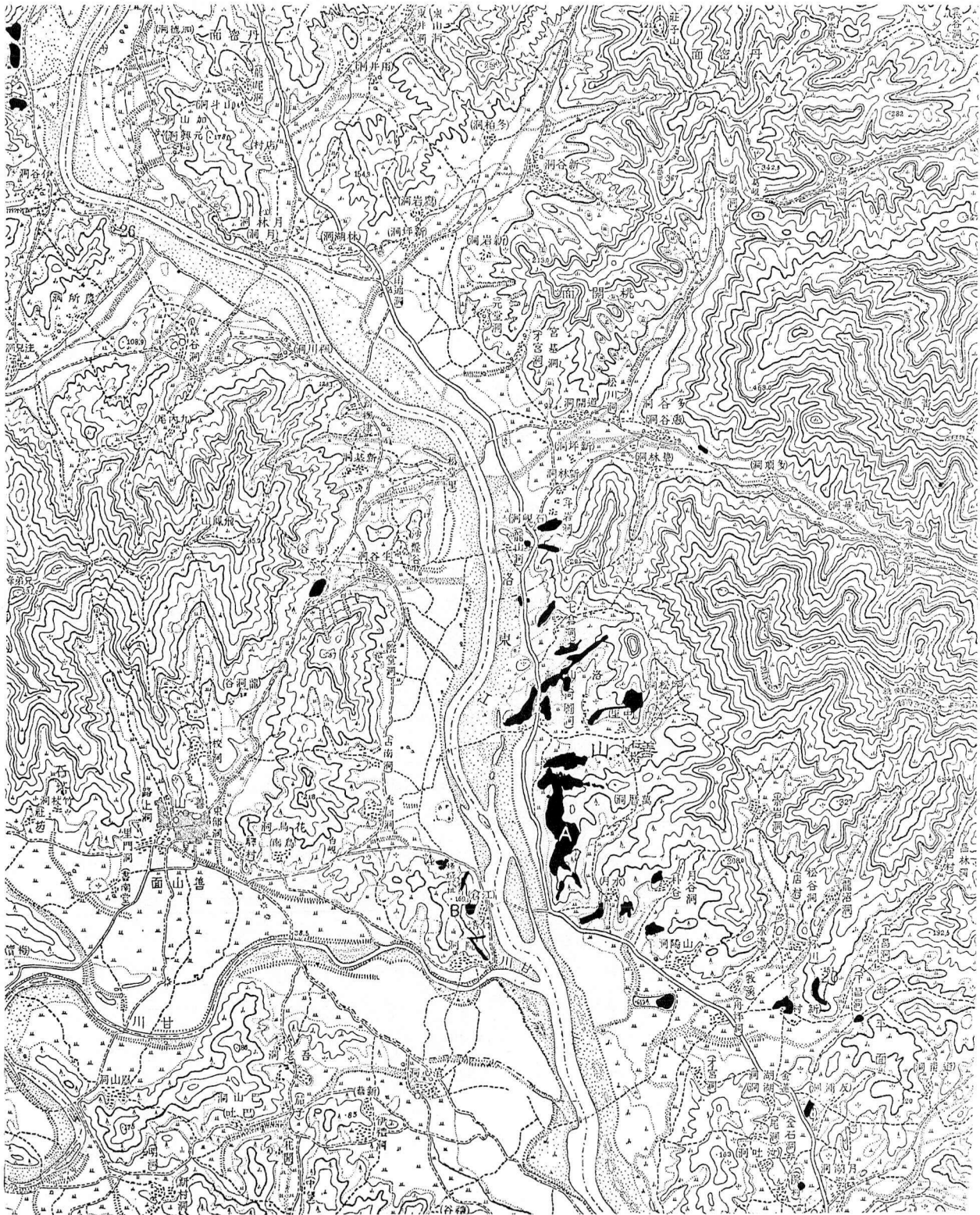
Abb. 9. Die Lage der Grabgruppen der Nekropole von Sounsansan. M. 1 : 75000.
