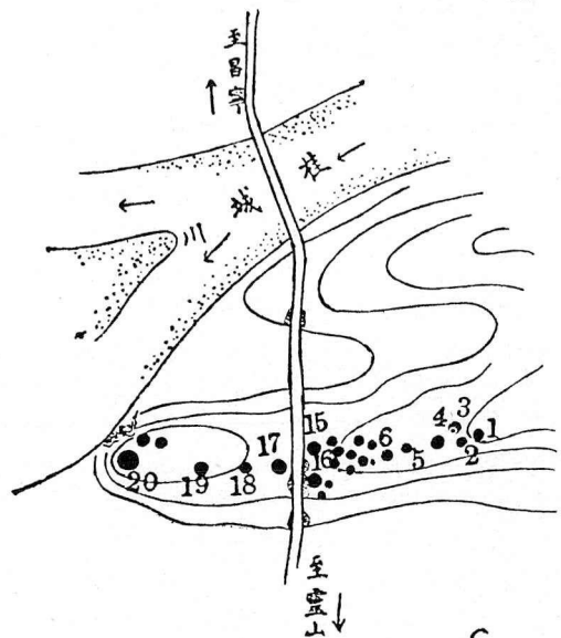
Abb. 20. a) Die Lage der Gräberfelder von Youngsan (1) und Gesuong (2) sowie der Höhenbefestigung (3). M. 1 : 50000. b) Plan des Gräberfeldes von Youngsan (schematische Skizze, Maßstab unbekannt). c) Plan des Gräberfeldes von Gesuong (schematische Skizze, Maßstab unbekannt).
