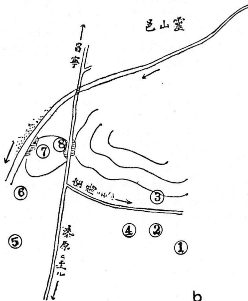
Abb. 20. a) Die Lage der Gräberfelder von Youngsan (1) und Gesuong (2) sowie der Höhenbefestigung (3). M. 1 : 50000. b) Plan des Gräberfeldes von Youngsan (schematische Skizze, Maßstab unbekannt). c) Plan des Gräberfeldes von Gesuong (schematische Skizze, Maßstab unbekannt).
