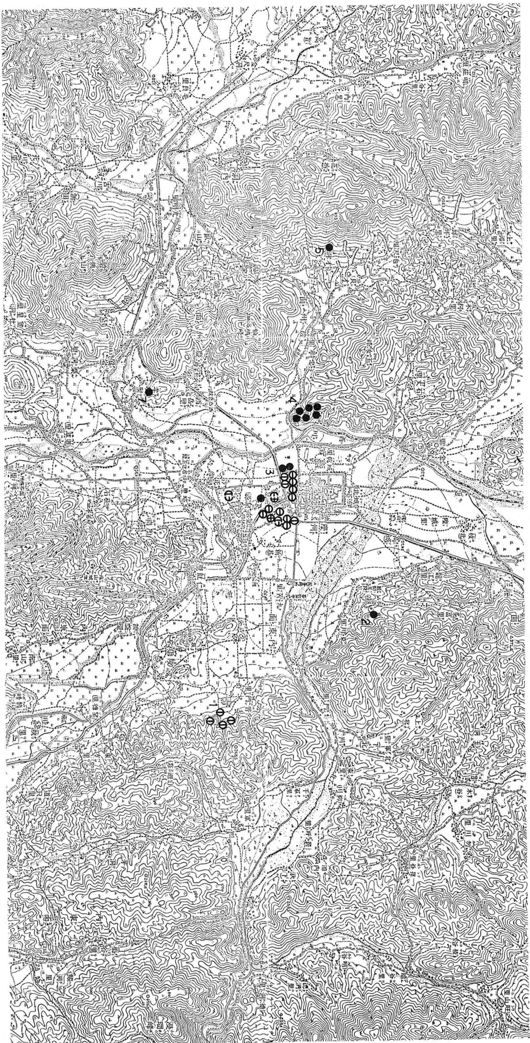
Abb. 117. Gräberfelder des Kyongju-Gebietes. Die Bezifferung bezieht sich auf das Fundstellenverzeichnis. M. 1 : 75000. ● Stufe A, ⊙ Stufe B, ⊕ Stufe C, ○ Stufe D.
