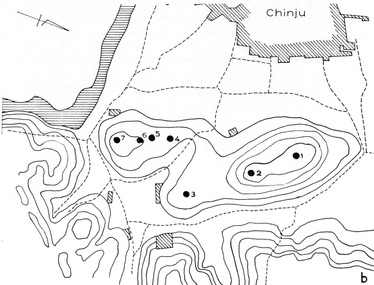
Abb. 23. a) Die Lage des Gräberfeldes von Okbongdong. M. 1 : 50000. b) Plan des Gräberfeldes von Okbongdong. M. 1 : 1200.
