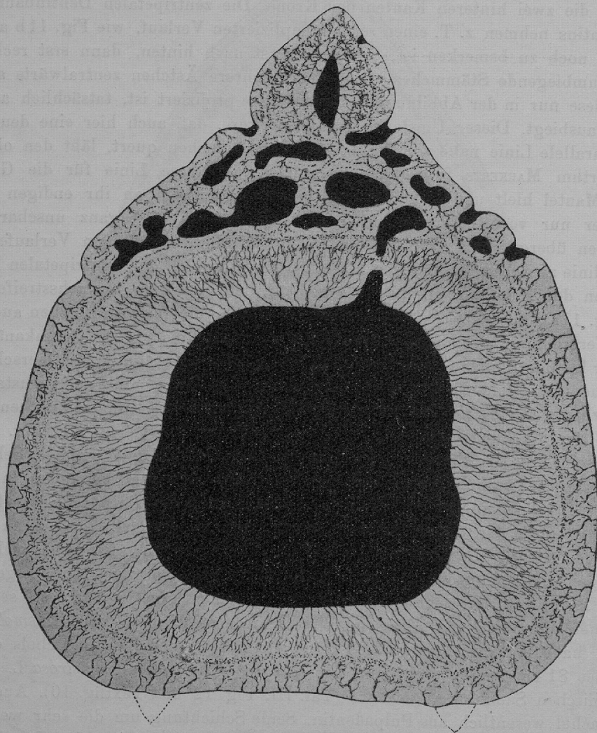
Textfig. 10. Querschnitt über der Mitte der Höhe des Flossenstachels von Chimera monstrosa stark vergrößert, nach einem etwas höheren Querschnitte ergänzt und ein wenig schematisiert.
