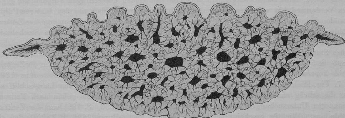
Textfig. 14. Querschnitt durch die Mitte eines Schwanzstachels eines Myliobatiden und Trygoniden , stark vergrößert und etwas schematisiert nach BENDA 1882 und RITTER 1900 und nach einem Querschliff durch ein Stachelstück aus dem Mittelmiozän Oberbayerns.
