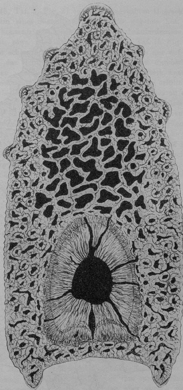
Textfig. 12. Querschnitt über der Mitte eines Flossenstachels von Nemacanthus monilifer aus der obersten Trias, stark vergrößert und etwas schematisiert, ergänzt und kombiniert nach mehreren Querschliffen durch Flossenstachelstückchen aus rhätischen Bonebeds Württembergs.
