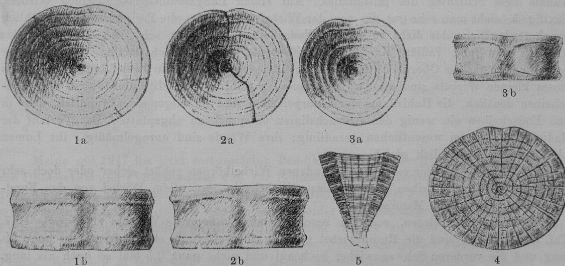
Textfig. 1—5. Wirbelkörper (Nr. 1912 VIII 52) zusammen 500 m westlich des Gebel Maghrafte gefunden, zu Onchoprists numidus (HAUG) gehörig. Fig. 1a, b großer Rumpfwirbel von vorn und oben; Fig. 2a, b kleinerer Rumpfwirbel von vorn und oben; Fig. 3a, b vorderer Schwanzwirbel von vorn und oben; Fig. 4 mittlerer Querschliff durch einen großen Rumpfwirbel, etwas schematisiert; Fig. 5 mittlerer Längsschliff durch die Hälfte eines vorderen Schwanzwirbels in doppelter Größe.
