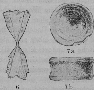
Textfig. 6. Medianer Längsschnitt durch einen halben Lendenwirbel von Platyspondylus Fourcaui HAUG (Nr. 1911 XII 17b) vom Fundorte A des Gebel Mandische. Textfig. 7. Vorderer Schwanzwirbel (Nr. 1911 XII 16) aus einer roten Schicht 1,5 m unter dem Basalt nahe dem Südosteck des Gebel Mandische, zu Platyspondylus Fourcaui HAUG gehörig, Fig. 7a von vorn, 7b von oben.
