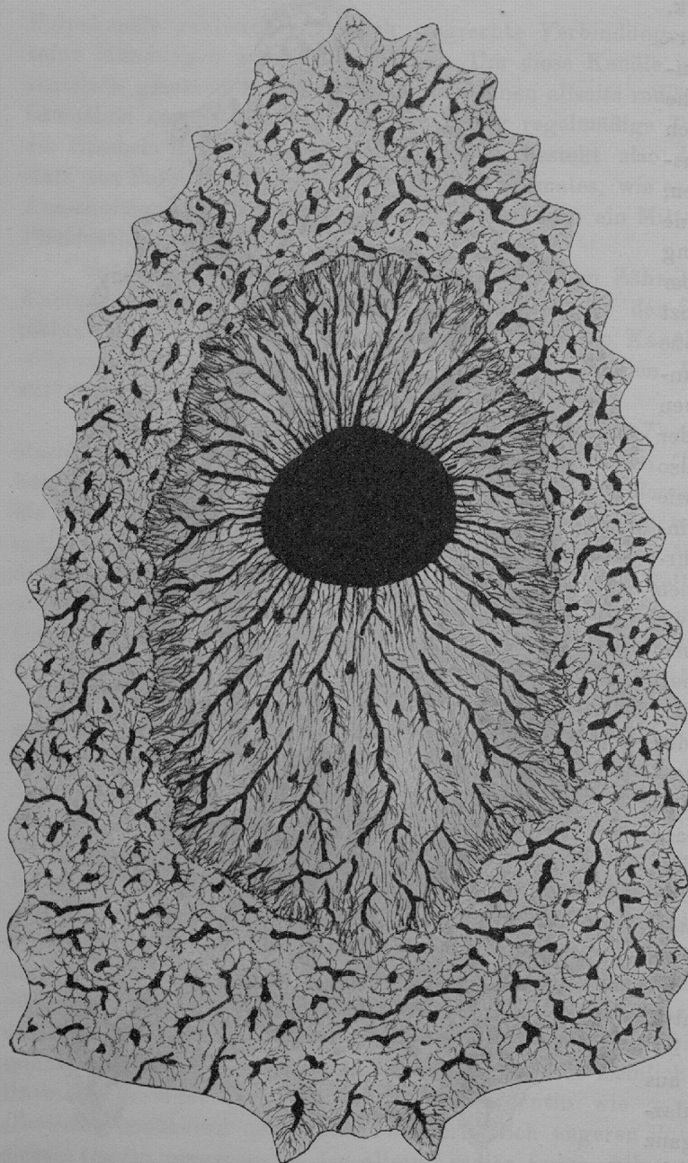
Textfig. 13. Querschnitt über der Mitte eines Flossenstachels von Hybodus Aschersoni aus der mittleren Kreide, nach Fig. 9a auf Taf. III ergänzt und etwas schematisiert.
