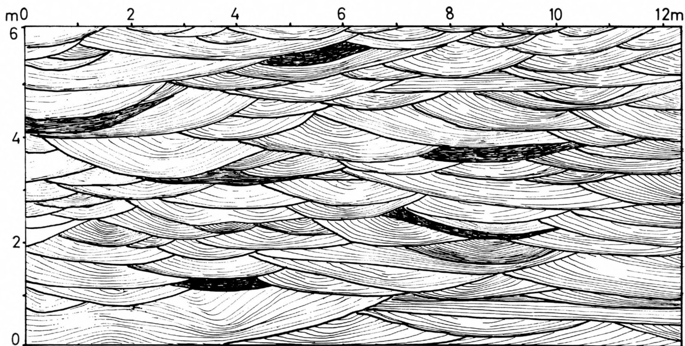
Abb. 2. Sandgrube Goppertshofen b. Dachau/Obb. (Erläuterungen s. Text S. 21/22 und Abb. 1). Detail aus der Aufschlußwand.
