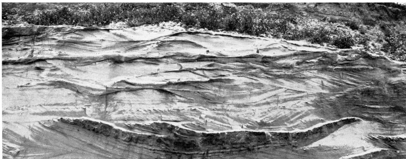
Abb. 1. Sandgrube Goppertshofen b. Dachau/Obb. (Erläuterungen s. Text S. 21/22). Aufschlußwand (Streichen ca. 10^\circ ) etwa senkrecht zur Transportrichtung a des Sedimentes. Der bc-Schnitt durch die Sedimentationskörper zeigt Bogensichtungung mit erhaltenen Mulden und gekappten Sätteln.
