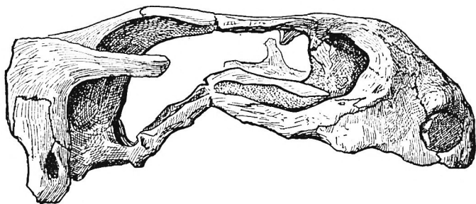
Fig. 1. Synostocephalus van hoepeni nov. gen. nov. spec. Münchn. Samml. Nr. 1934 VIII 24. Karrooformation, unt. Beaufort-Schichten, Endothiodon-Zone (ob. Perm). Farm Lombardskraal bei Beaufort West, Kap-Provinz, Südafrika. — Seitenansicht des Schädels. — Nat. Gr.
