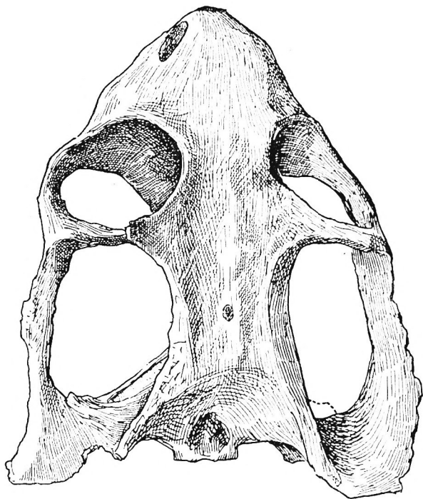
Fig. 20. Brachyuraniscus reuningi nov. gen. nov. spec. Exemplar und Fundort wie Fig. 19. — Oberseite des Schädels. — Nat. Gr.
