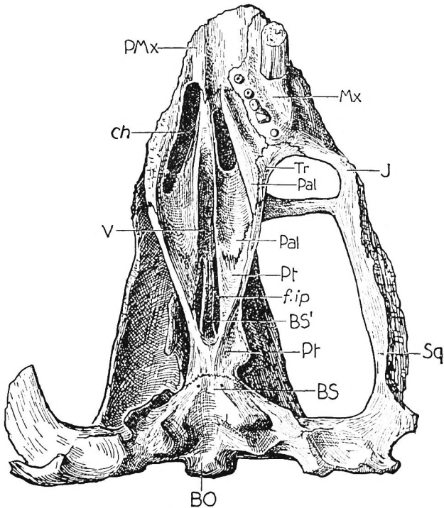
Fig. 14. ? Cryptocynodon spec. Exemplar und Fundort wie Fig. 10. — Unterseite des Schädels. — Nat. Gr.
