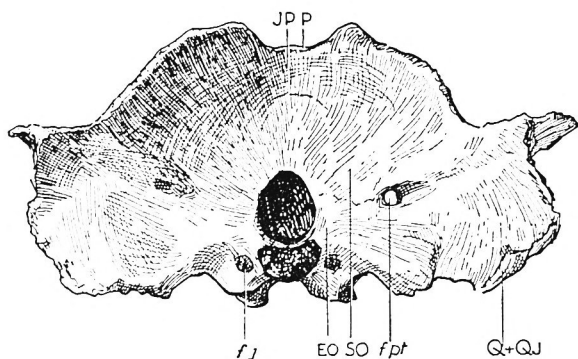
Fig. 13. ? Cryptocynodon spec. Exemplar und Fundort wie Fig. 10. — Hinteransicht des Schädels. — Nat. Gr.
