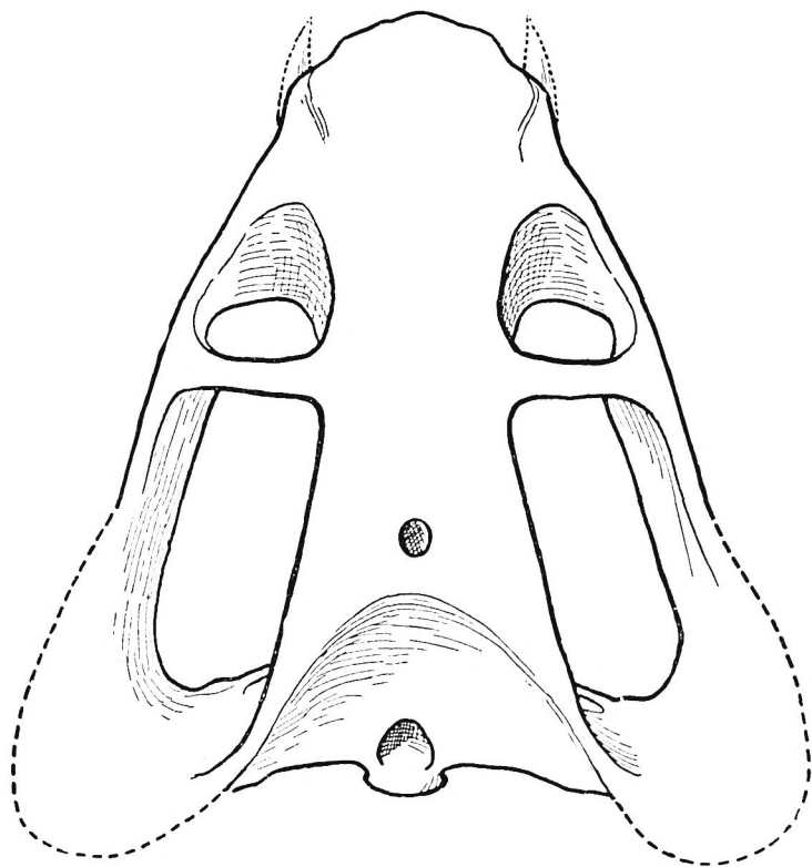
Fig. 12. ? Cryptocynodon spec. Exemplar und Fundort wie Fig. 10. — Rekonstruktion des Schädels. Oberseite. — Nat. Gr.
