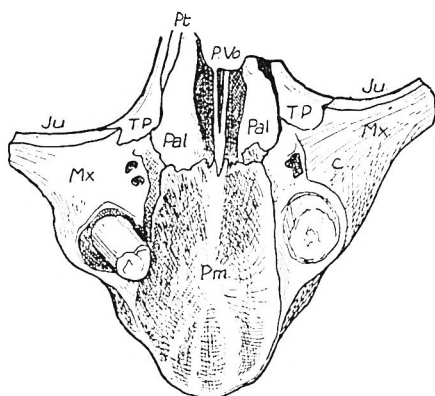
Fig. 9. Tropidostoma microtrema (Seeley). Vordere Gaumenregion. \frac{1}{2} nat. Gr. — Nach Broom (1915).
