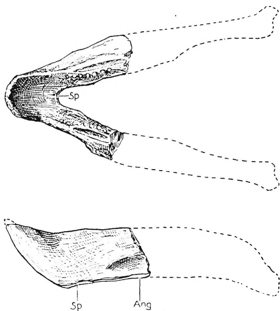
Fig. 8. Synostocephalus van hoeperi nov. gen. nov. spec. Exemplar und Fundort wie Fig. 1. — Unterkiefer von oben und von links. — Nat. Gr. Ang Angulare. Sp Spleniale.
