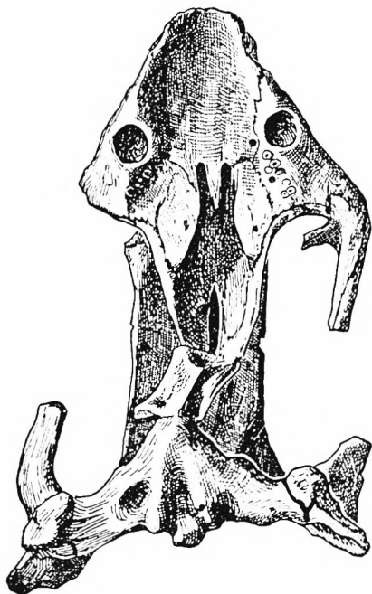
Fig. 4. Synostocephalus van hoeperi nov. gen. nov. spec. Exemplar und Fundort wie Fig. 1. — Unterseite des Schädels. — Nat. Gr.
