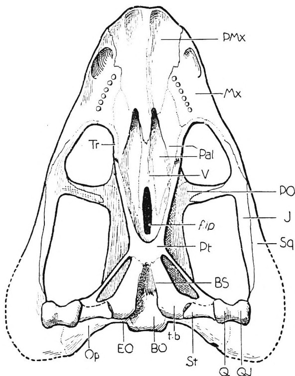
Fig. 30. Eurychororhinus boonstrai nov. gen. nov. spec. Exemplar und Fundort wie Fig. 23. — Rekonstruktion des Schädels. Unterseite. — Nat. Gr. BO Basioccipitale. BS Basisphenoid. EO Exoccipitale laterale. f. ip. Interpterygoid-Lücke. J Jugale. Mx Maxillare. Op Opisthoticum. Pal Palatin. PMx Praemaxillare. PO Postorbitale. Pt Pterygoid. Q Quadratum QJ Quadratojugale. Sq Squamosum. St Stapes. t. b. Tuber basisphenoidale. Tr. Ectopterygoid (Transversum). V „Vomer“.
