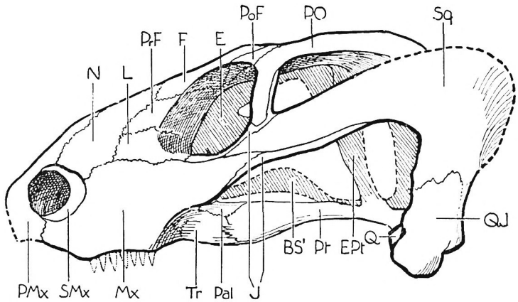
Fig. 27. Eurychororhinus boonstrai nov. gen. nov. spec. Exemplar und Fundort wie Fig. 23. — Rekonstruktion des Schädels. Seitenansicht. — Nat. Gr. BS' Rostrum des Basisphenoids. E Ethmoid. Ept Epipterygoid. F Frontale. J Jugale. L Lacrimale. Mx Maxillare. N Nasale. Pal Palatin. PMx Praemaxillare. PO Postorbitale. PoF Postfrontale. PrF Praefrontale. Pt Pterygoid. Q Quadratum. QJ Quadratojugale. SMx Septomaxillare. Sq Squamosum. Tr Ectopterygoid (Transversum).
