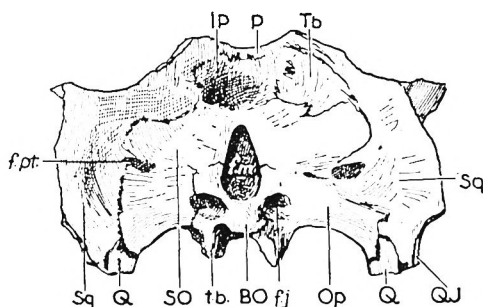
Fig. 3. Synostocephalus van hoeepeni nov. gen. nov. spec. Exemplar und Fundort wie Fig. 1. — Hinteransicht des Schädels. — Nat. Gr.
