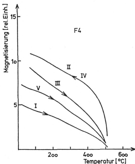
Abb. 5. Natürliche remanente Magnetisierung NRM (Kurve V), z -Komponente der NRM (Kurve I, Erhitzung, Erdfeld kompensiert), thermoremanente + induzierte Magnetisierung während der Abkühlung in einem Feld von 0,57 Oe (Kurve II, IV) und künstliche Thermoremanenz (Kurve III, erneute Erwärmung, Erdfeld kompensiert) als Funktion der Temperatur. Kurve III liegt unter Kurve II, da bei Messung der Kurve III das äußere Magnetfeld Null und damit die induzierte Magnetisierung Null war. Der Vergleich der Kurven III und V wird zur Bestimmung der Paläointensitäten verwendet (siehe Text). Die Probe F 4 stammt aus dem Lavastrom von 1950/51 bei Fornazzo
