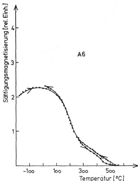
Abb. 7. Temperatur-Abhängigkeit der Sättigungs-Magnetisierung der Probe A 6, gemessen in einem Magnetfeld von 5000 Oe. Dominierende Phase mit einem Curiepunkt bei 250 °C
