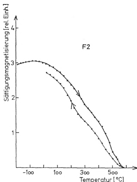
Abb. 9. Temperatur-Abhängigkeit der Sättigungs-Magnetisierung der Probe F 2, gemessen in einem Magnetfeld von 5000 Oe. Verschiedene magnetische Phasen mit unterschiedlichen Curie-Temperaturen sind erkennbar
