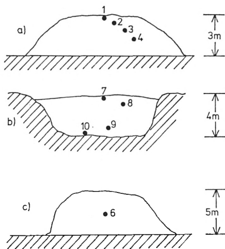
Abb. 2a. Die Lage der Proben im Lavastrom von 1910. Erster Aufschluß an der Straße von Nicolosi kommend gelegen (etwa 5 km nördlich von Nicolosi) b. Eine Kehre höher, etwa 50 m rechts der Straße ein kleiner Steinbruch c. Zwei Kehren höher, an der rechten Straßenseite
