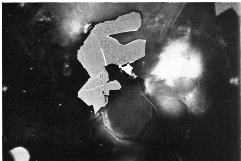
Abb. 13. Erzkorn in der Probe F 2 (Lava von 1950 bei Fornazzo). Titanomagnetit (grau) mit schwachen Zeichen einer beginnenden Umwandlung (Granulation in den mittleren Teilen des Kornes). Vergr. 1400 \times , Ölimmersion
