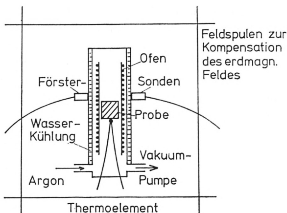
Abb. 4. Schematische Darstellung der Apparatur, die zur Bestimmung der Paläointensitäten verwendet wurde
