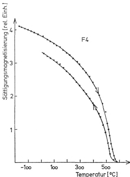
Abb. 8. Temperatur-Abhängigkeit der Sättigungs-Magnetisierung der Probe F 4 , gemessen in einem Magnetfeld von 5000 Oe
