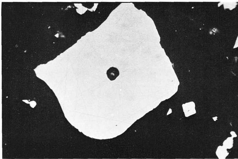
Abb. 11. Homogenes Titanomagnetit-Korn (grau) in der Probe A 6. Keine Anzeichen von beginnender Entmischung bzw. Oxydation erkennbar. Vergr. 800×, Ölimmersion
