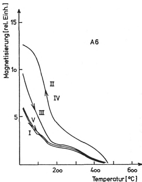
Abb. 6. Wie in Abb. 5. Die Probe A 6 stammt aus dem Lavastrom von 1910, etwa 5 km nördlich von Nicolosi
