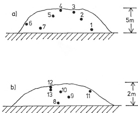
Abb. 3 a. Die Lage der Proben im Lavastrom von 1950/51 bei Fornazzo. Westliche Seite des Steinbruchs
