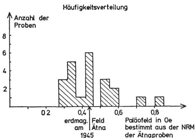
Abb. 14. Häufigkeitsverteilung der Werte der gemessenen Paläointensitäten
