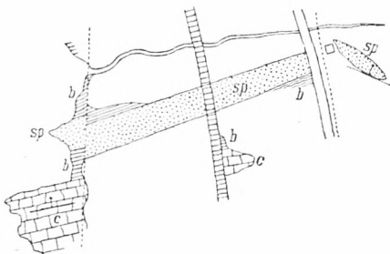
Fig. 4. Links das Seeufer, rechts die Fahrstrasse Moelven-Ring, in der Mitte die Eisenbahnlinie, im Norden der Smedstad-elven. sp Sparagmit, c Quarzsandstein, b Birikalk. Die zwei N-S gerichteten punktierten Linien Querverwerfungen.
