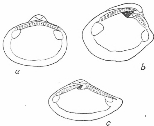
Abb. 1. Nuculidenschloß. a) Ctenodonta , b) Nucula , c) Leda .
