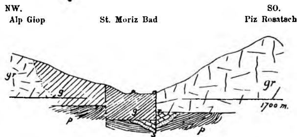
Fig. 2. Schnitt quer über das Innthal (1:75000) mit den muthmasslichen tektonischen Verhältnissen unterhalb des 1700 Meter-Niveaus.
