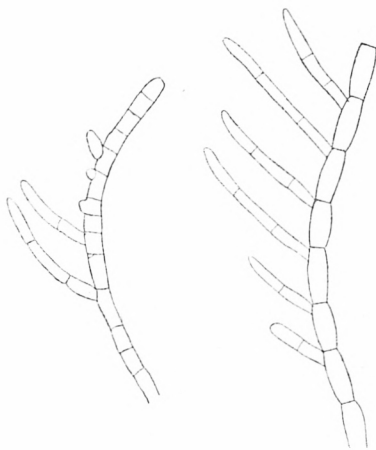
Fig. IV und V. Einzelne Fäden aus dem in Fig. III abgebildeten Protonemapolster.
