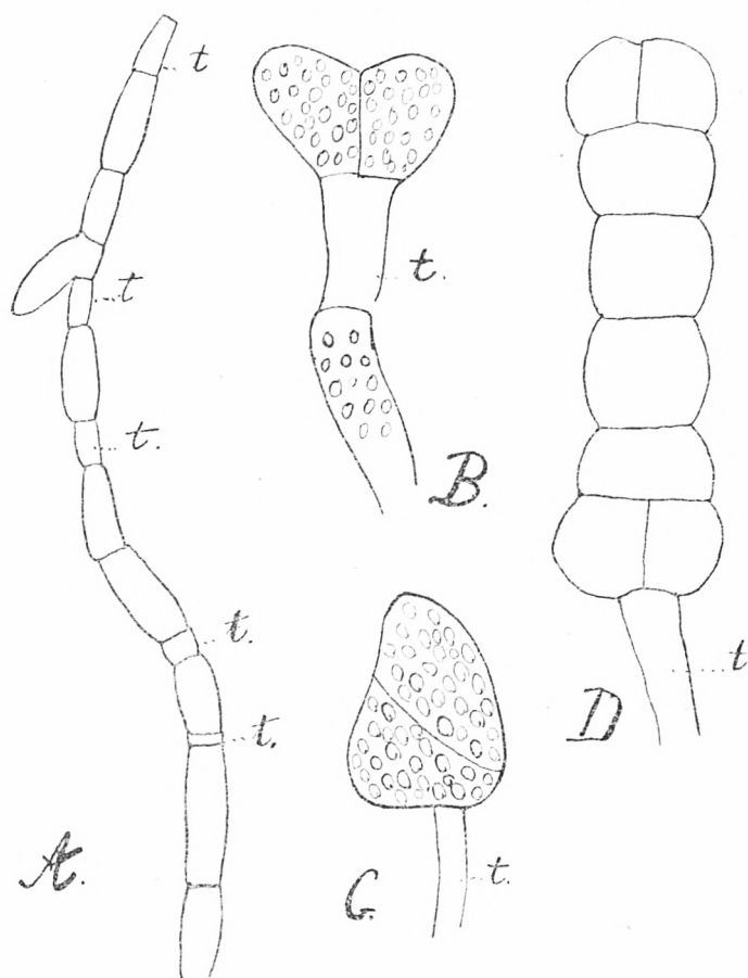
Fig. VI. Gemmenbildung des Protonema's von Funaria hygrometrica (die Figuren sind bei verschiedener Vergrösserung gezeichnet). t die leeren Zellen. In manchen Fällen treten in den Fäden Längswände auf.
