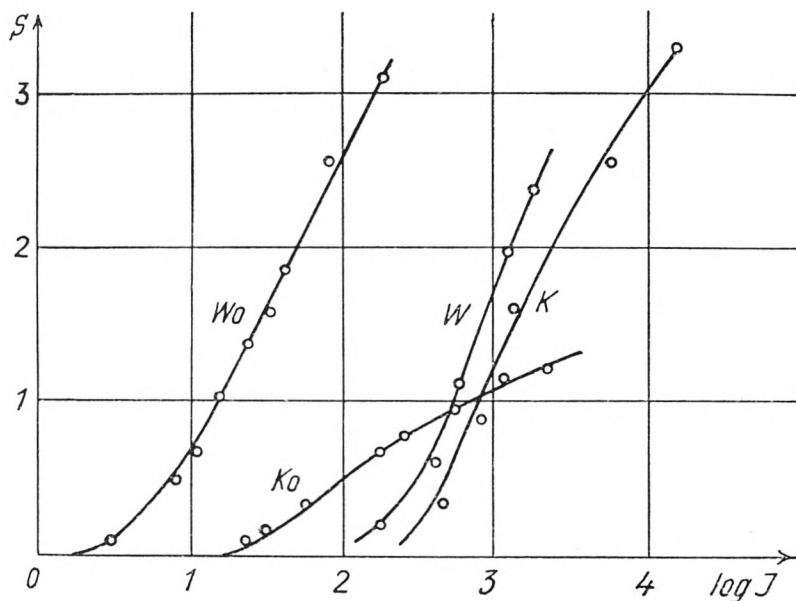
Fig. 2. Schwärzungskurven bei Pinakryptolgelb
