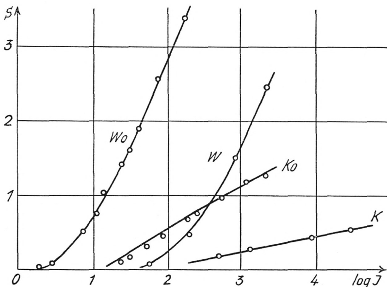
Fig. 1. Schwärzungskurven bei Phenosafranin
