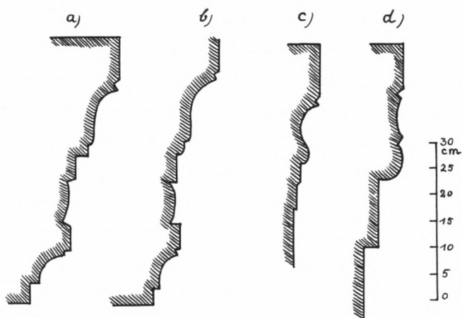
Abb. 6. Gebäude A, Profile. 1911. Aufnahme und Zeichnung S. Guyer.
