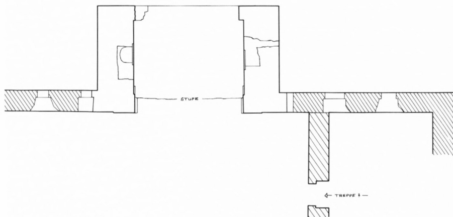
Abb. 11. Festung. Obergeschoß des Ostraktes. Aufnahme und Zeichnung U. Peschlow.
