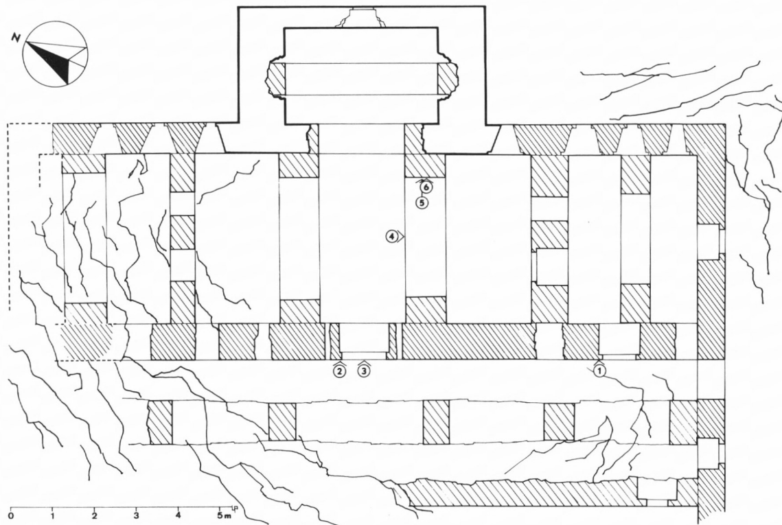
Abb. 10. Festung. Untergeschoß des Ostraktes. Aufnahme und Zeichnung U. Peschlow.
