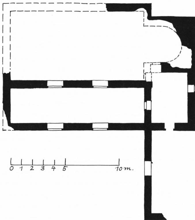
Abb. 5. Gebäude A, Grundriß. Zustand von 1911. Aufnahme und Zeichnung S. Guyer.
