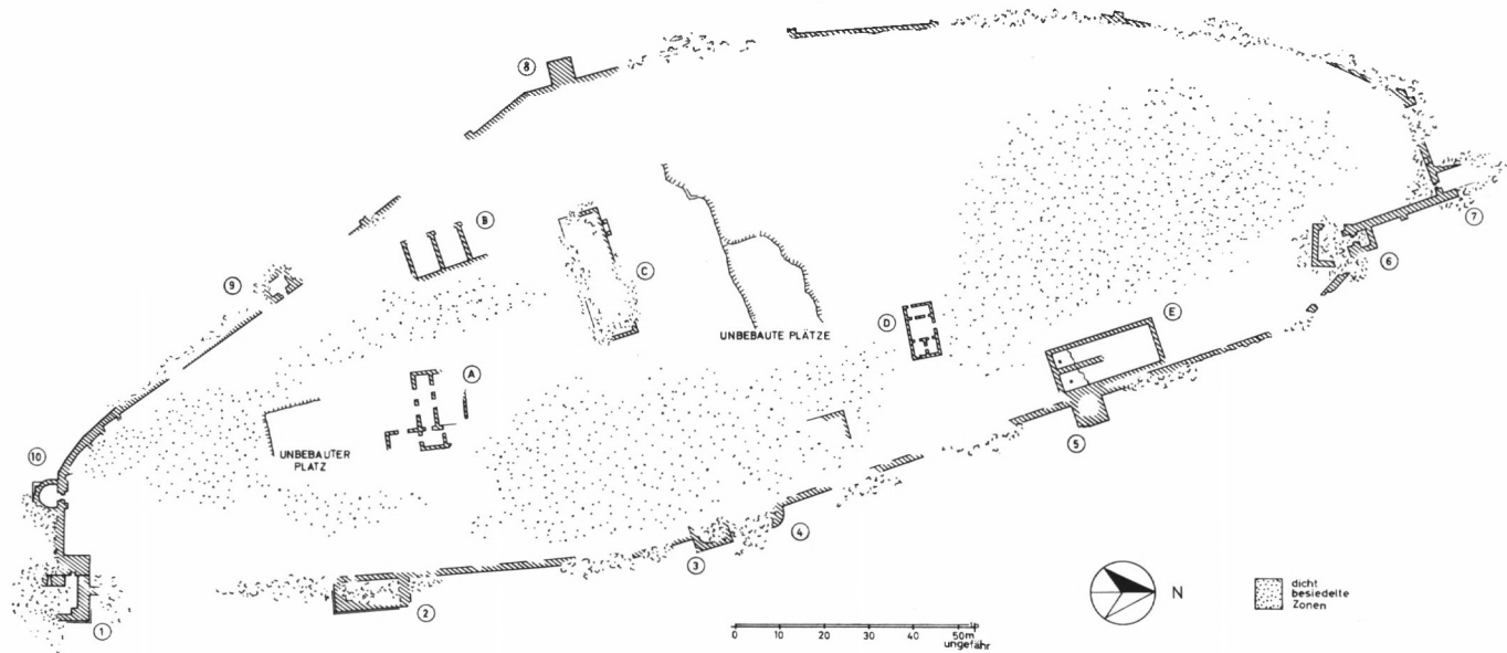
Abb. 1. Gesamtplan von Kale'i Zerzevan. Aufnahme und Zeichnung U. Peschlow.
