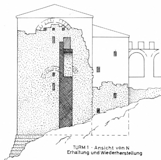
Abb. 2. Turm 1, Ansicht von Norden. Aufnahme und Zeichnung U. Peschlow.
