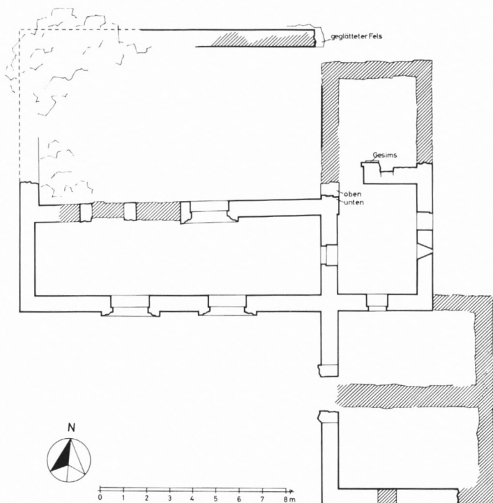
Abb. 4. Gebäude A, Grundriß. Heutiger Zustand. Aufnahme und Zeichnung U. Peschlow.
