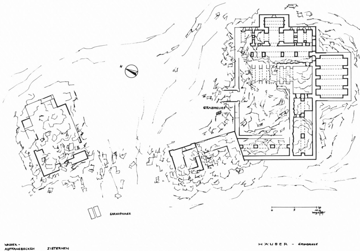
Abb. 9. Gesamtplan von Deyr Yakup. Aufnahme und Zeichnung U. Peschlow.
