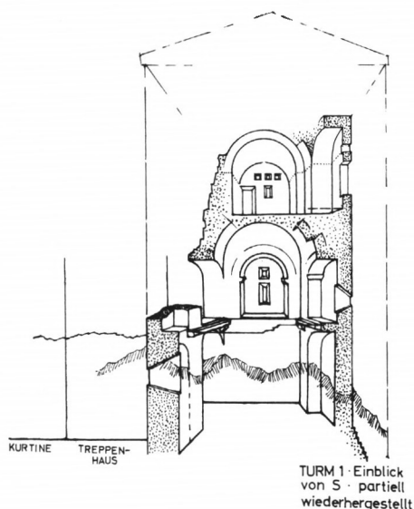
Abb. 3. Turm 1, Schnitt. Aufnahme und Zeichnung U. Peschlow.
