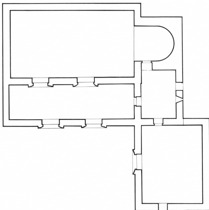
Abb. 7. Gebäude A (Kirche), rekonstruierter Grundriß. Zeichnung U. Peschlow.
