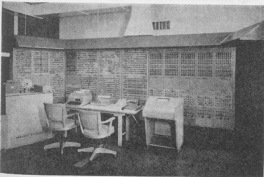
Bild 1: PERM im Zustand von 1961 nach Kernspeichererweiterung.
