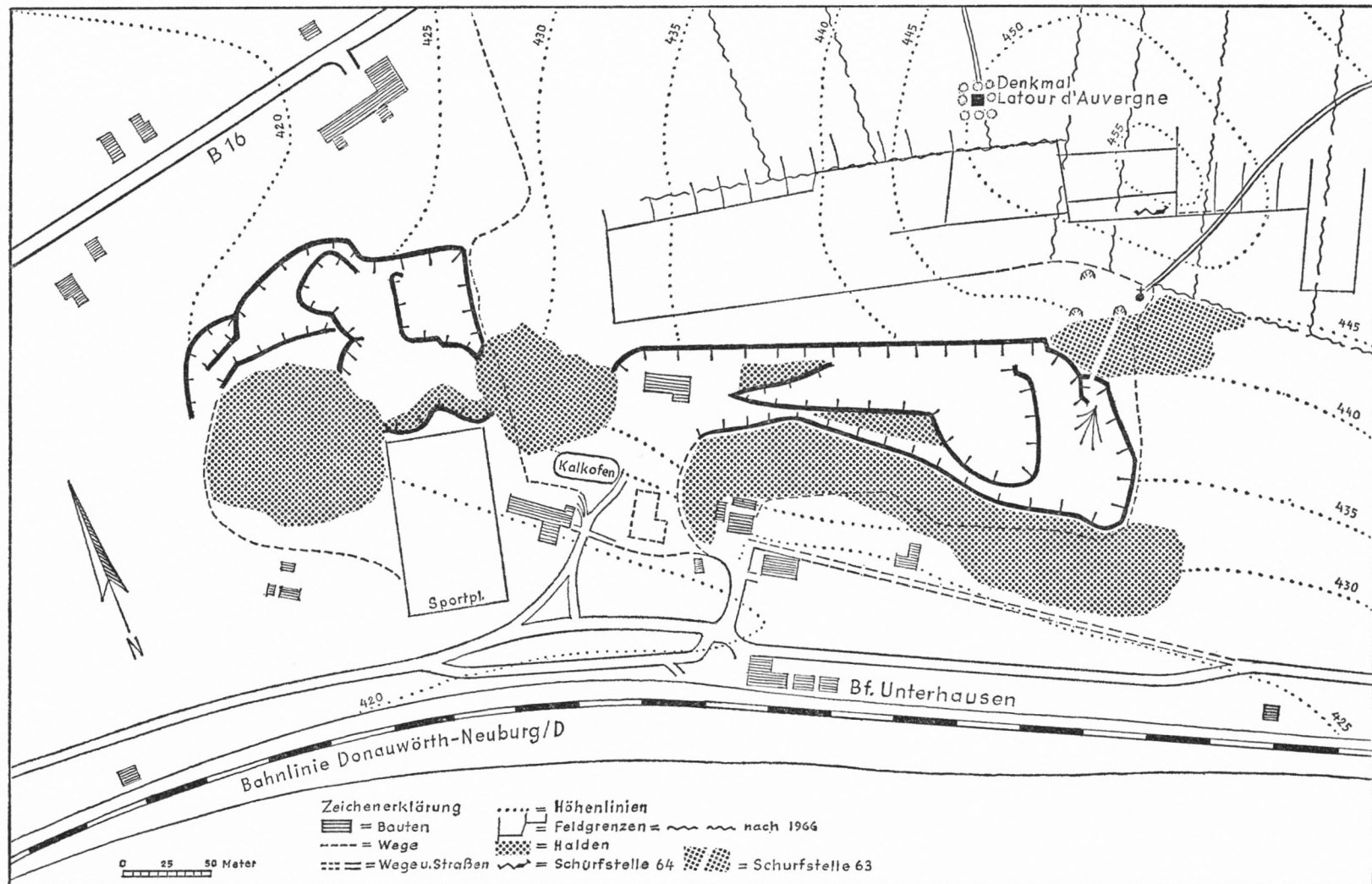
Abb. 2. Lage-Plan der Steinbrüche am Bahnhof Unterhausen und der Gemarkung Oberhausen im Bereich des Latour d'Auvergne-Denkmal (Nach einem Luftbild).
