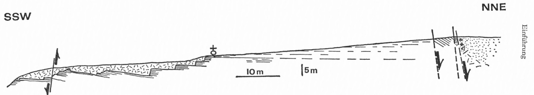
Abb. 5. Profil-Schnitt von der NE Ecke des großen Bruchs am Bahnhof Unterhausen zu den Schürfen am Latour-Denkmal (rechts). Oberkreide-Sande punktiert, Schicht-Signatur und punktierte Blöcke: oberster Jura. Im Schurf-Graben (links) SchuttSignatur.
