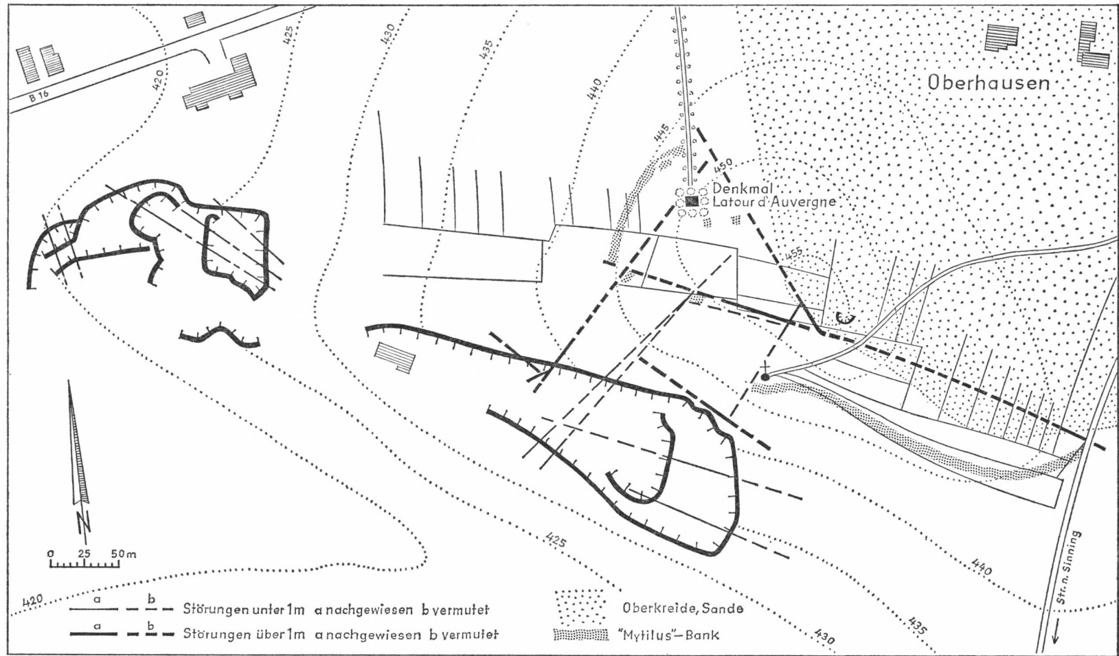
Abb. 3. Verlauf der Störungen im Obersten Jura zwischen Oberhausen und Unterhausen (nach einem Luftbild mit Erlaubnis der Rhein-Main-Donau A.G.).
