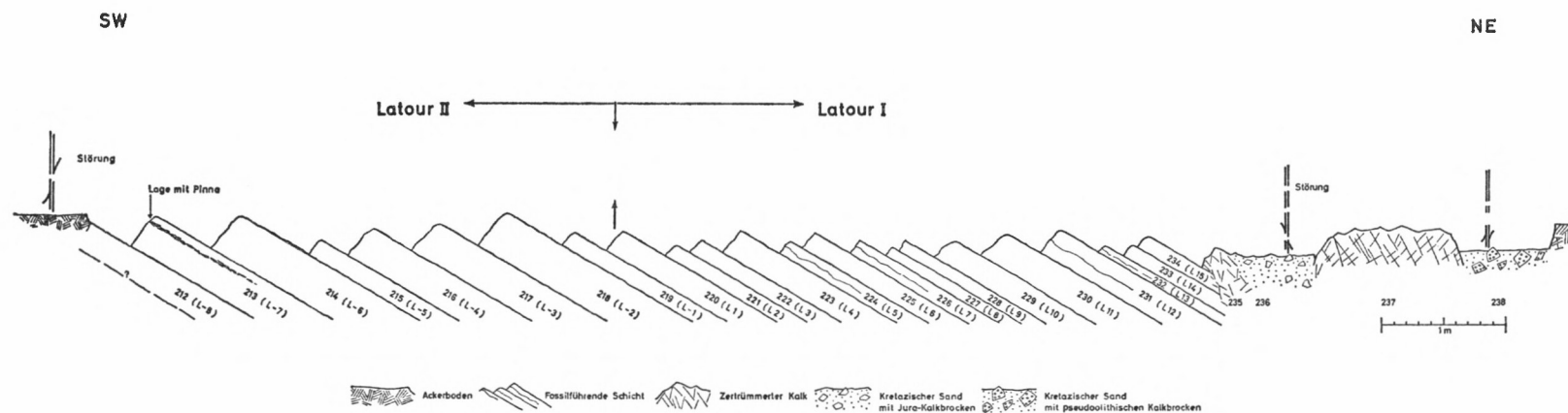
Abb. 7. Detaillierter Plan der Latour-Schürfe (oben) und zusammengefaßtes Profil (unten), das in den nicht-gebankten Seiten-Teilen verkürzt gezeichnet ist.
