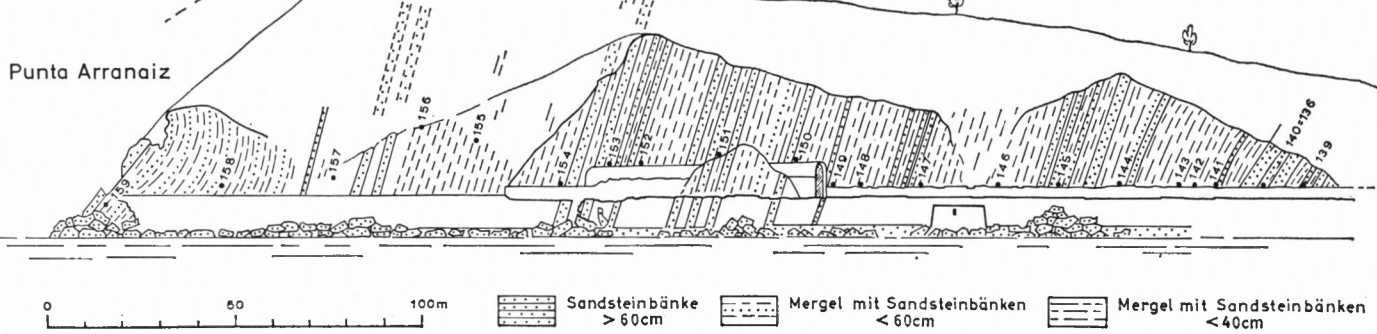
Profil 3. Straße Zumaya – Guetaria zwischen km 34 und 35
