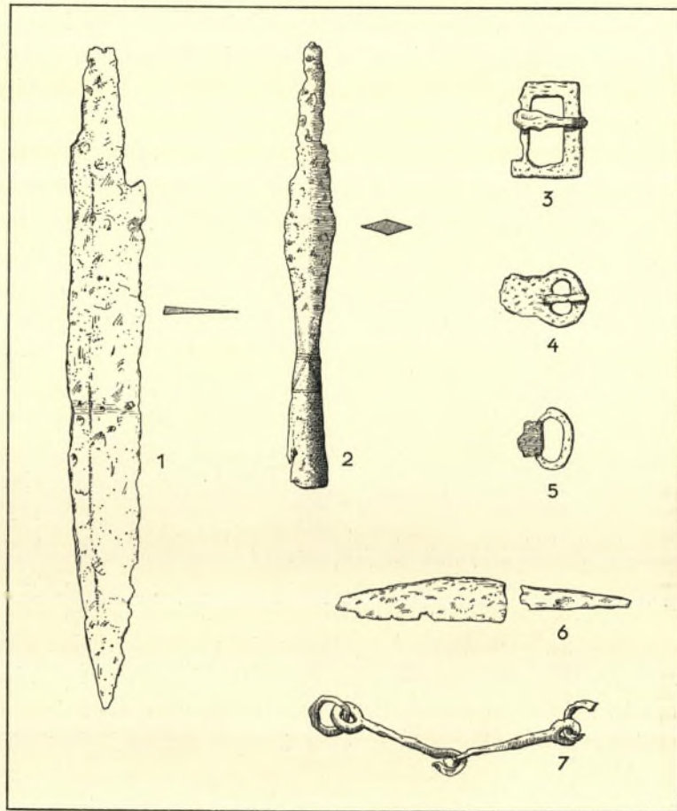
Abb. 4. Eiserne Waffen und Pferdezaumzeug aus dem Männergrab am „Hefeskreuz“ (III). M. 1: 4
