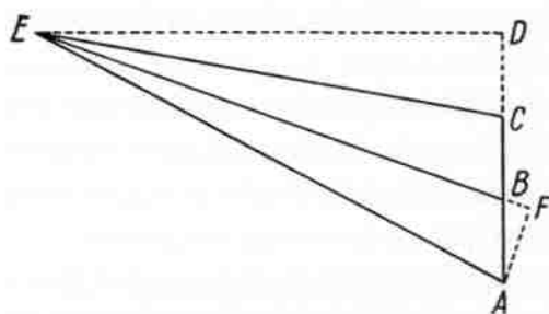
A Sol, B Centrum Eccentricij, C Centrum aequantis, E Planeta, ED Perpendicularis in AC continuatam, AF Perpendicularis in EB continuatam, si opus est.
