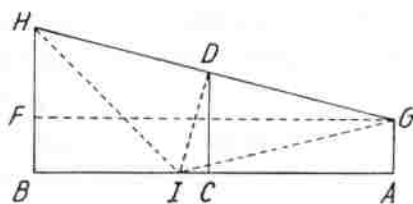
I Centrum \odot . G. D. H. centrum \gg invisibile in principio medio et fine, ut IG. IH utrumque aequalis sit summae semidiametrorum.
