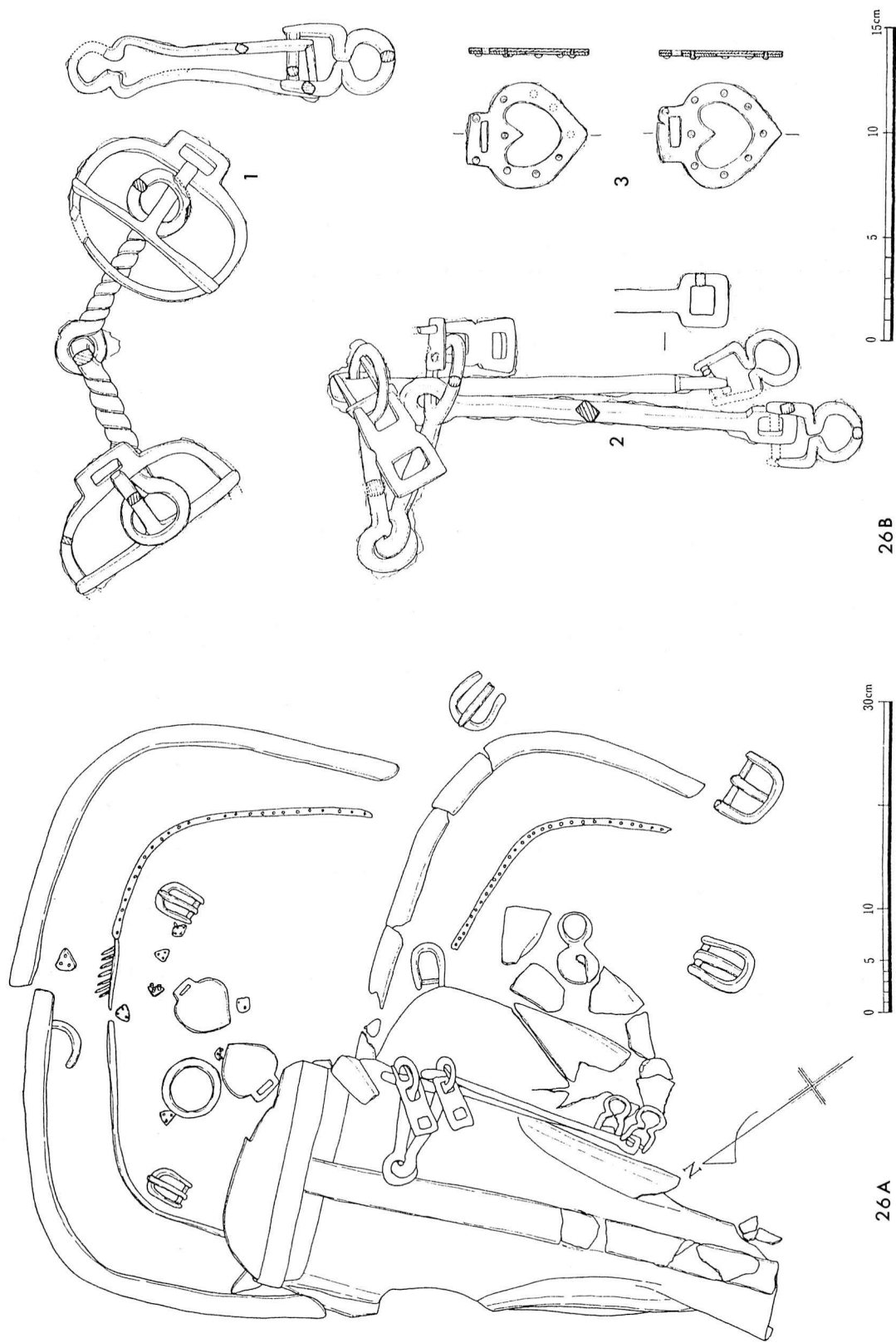
Abb. 26. Bokchondong Beigabenkammer 10. A: Eiserner Pferdekopfschutz und eiserne Sattelleinfassungen. M. 1:6. B: Eiserner Trensen. M. 1:3. Nach Kul-cheol Shin 1982 (Anm. 52) 20 Abb. 7 (A) und 55 Abb. 10 (B).
