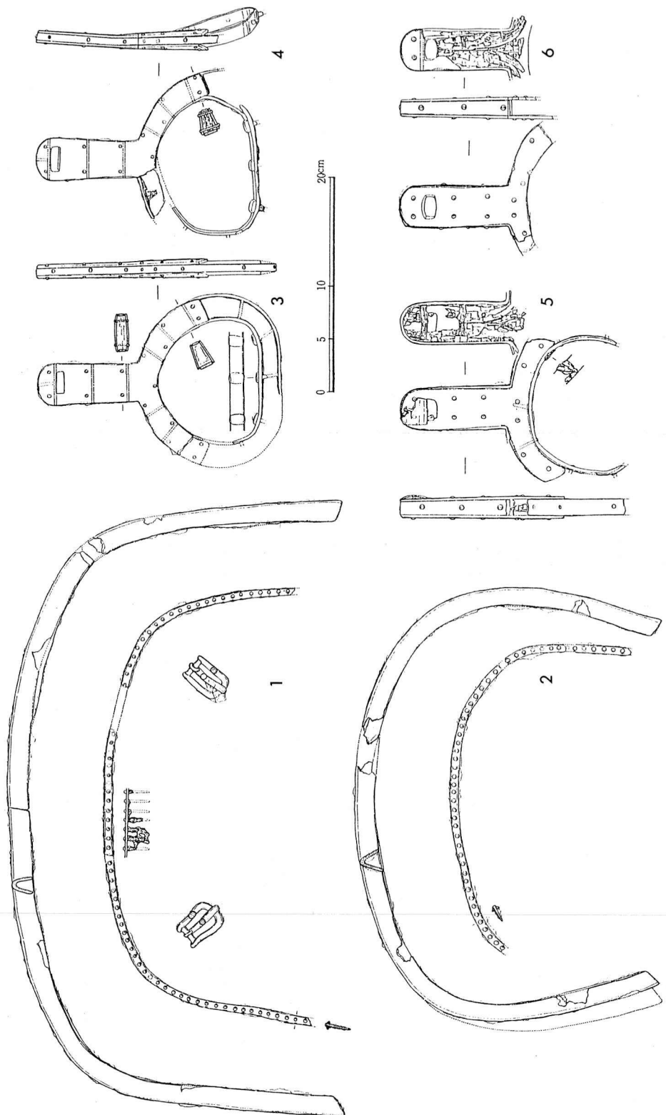
Abb. 27. Bokchondong Beigabenkammer 10. Zwei eiserne Sattelleinfassungen und zwei Paare eiserner Steigbügel. M. 1:5. Nach Kul-cheol Shin 1982 (Anm. 52) 53 Abb. 36.
