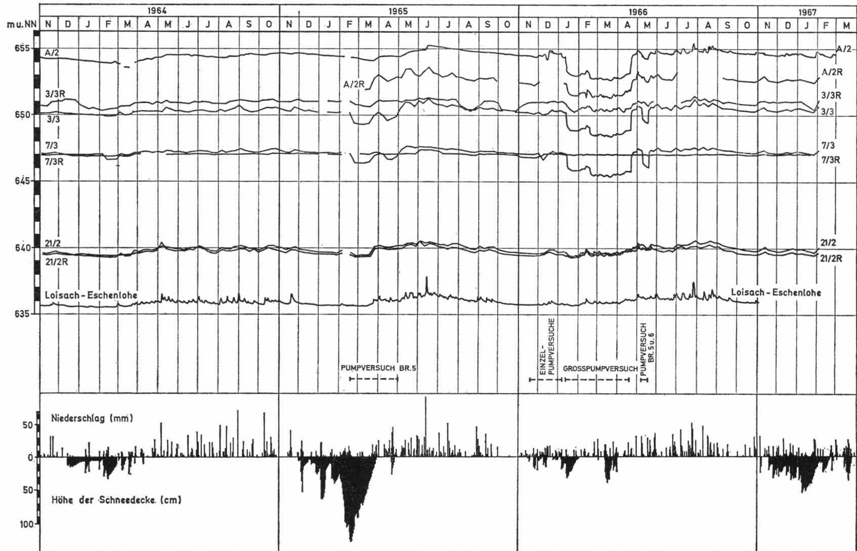
Abb. 26: Ganglinien von Grundwassermeßstellen zwischen Oberau und Eschenlohe und der Loisach am Pegel Eschenlohe mit den dazugehörigen Werten des Niederschlags und der Höhe der Schneedecke für die Niederschlagsmeßstelle Oberau.
