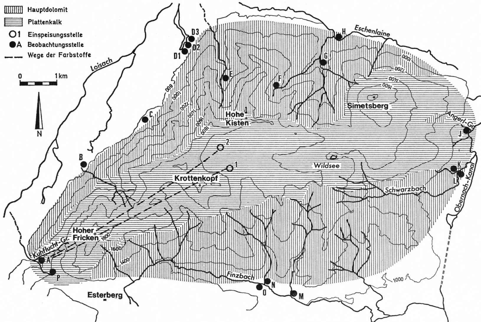
Abb. 9: Lageplan zum Färbeversuch am Krottenkopf.
