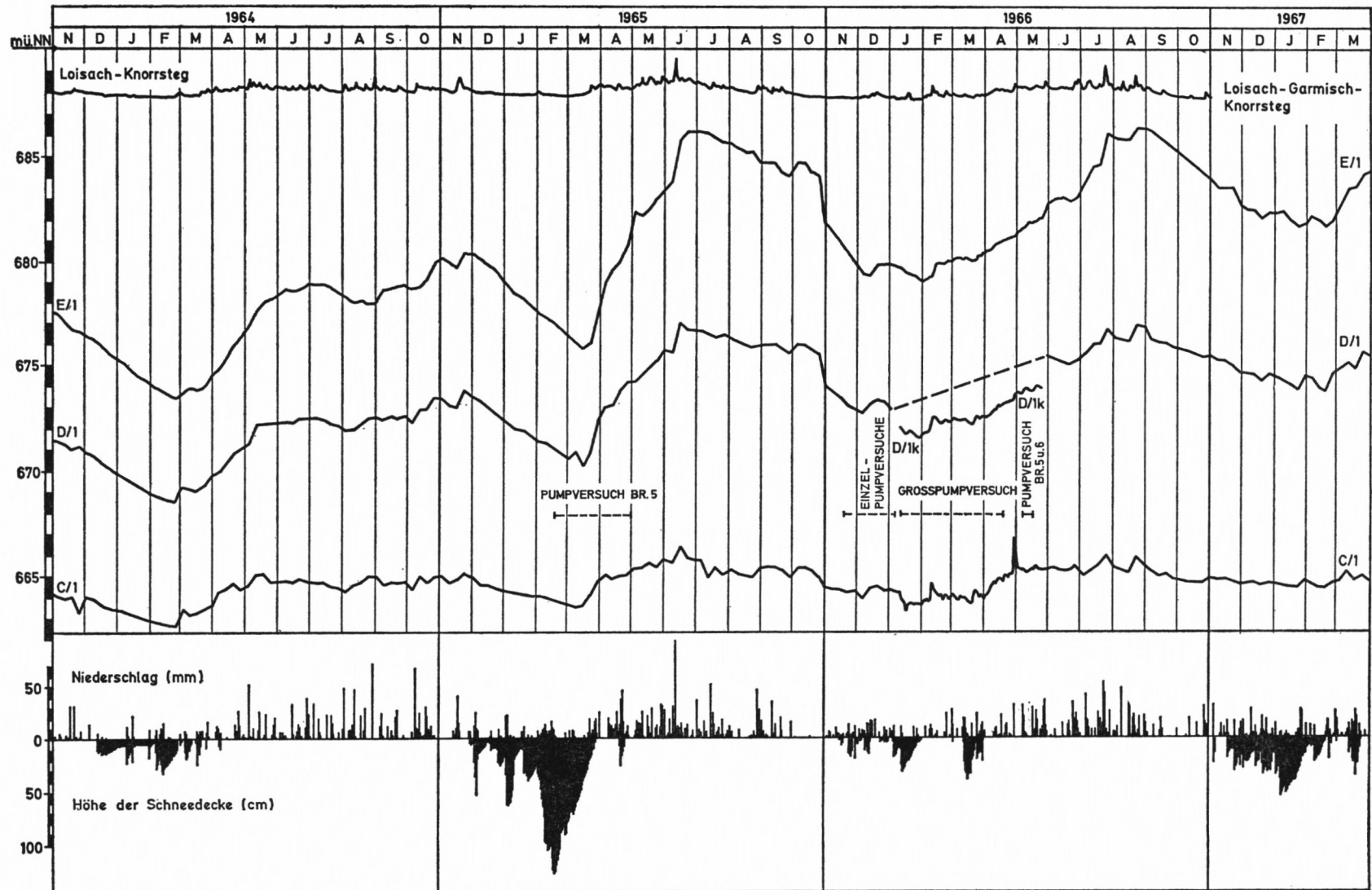
Abb. 25: Ganglinien der Grundwassermeßstellen E/1, D/1 (D/1k), C/1 und der Loisach am Pegel Garmisch-Knorrsteg mit den dazugehörigen Werten des Niederschlags und der Höhe der Schneedecke für die Niederschlagsmeßstelle Oberau.
