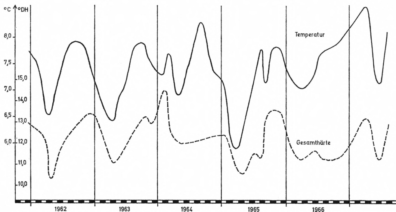
Abb. 31: Abhängigkeit der Temperatur und der Gesamthärte der Lauterbachquelle (Quell-Nr. 38) von der Jahreszeit (nach Kalenderjahr).
