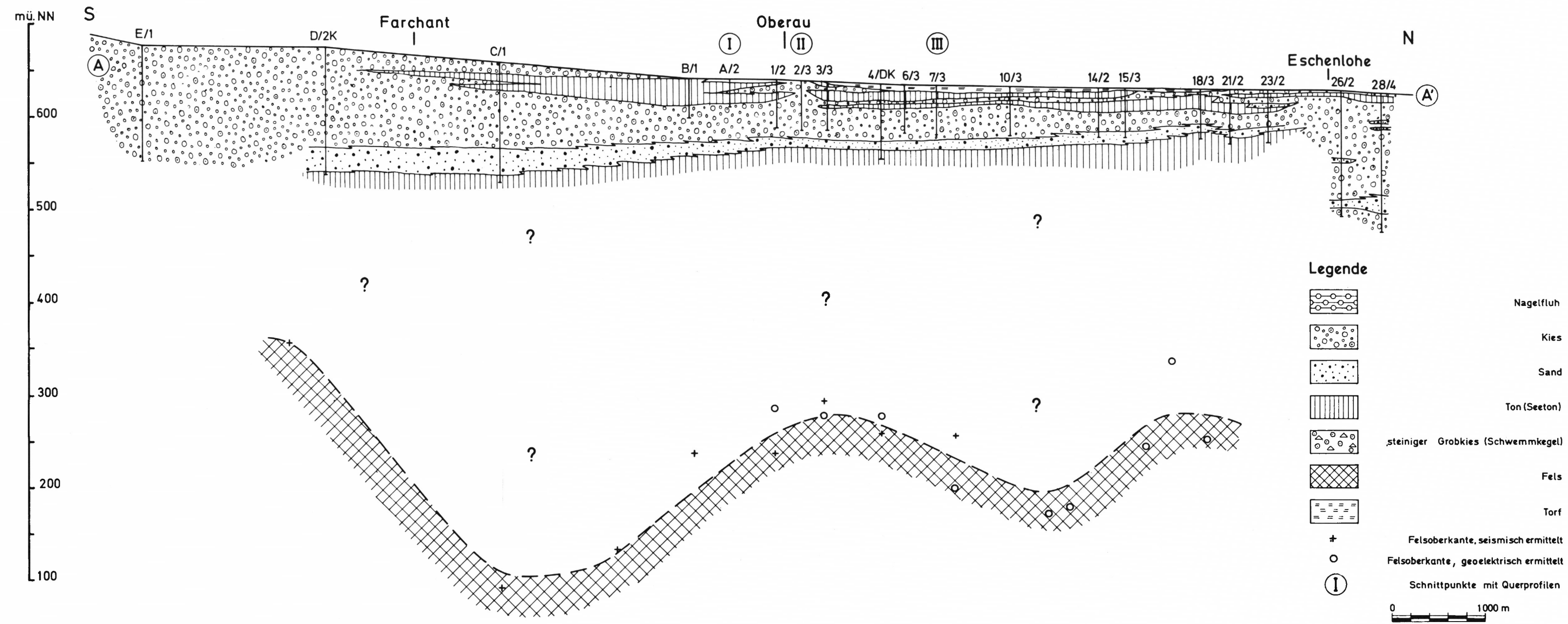
Abb. 13: GEOLOGISCHES NORD-SÜD-PROFIL DURCH DAS LOISACHTAL
