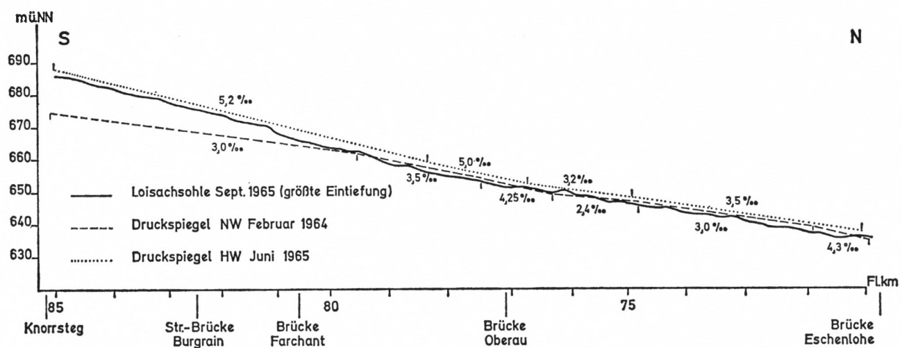
Abb. 24: NW- und HW-Druckspiegel (2. Stockwerk) und Loisachsohle.
