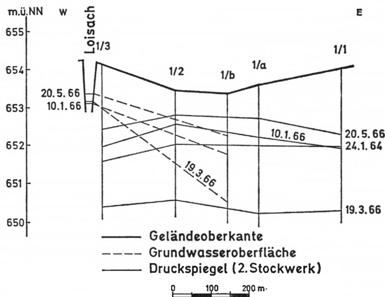
Abb. 36: Grundwasseroberfläche und Druckspiegel im Profil 1
