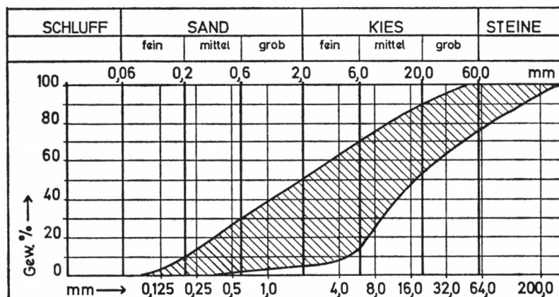
Abb. 3: Kornverteilungsband der Kiese im 2. Grundwasserstockwerk.
