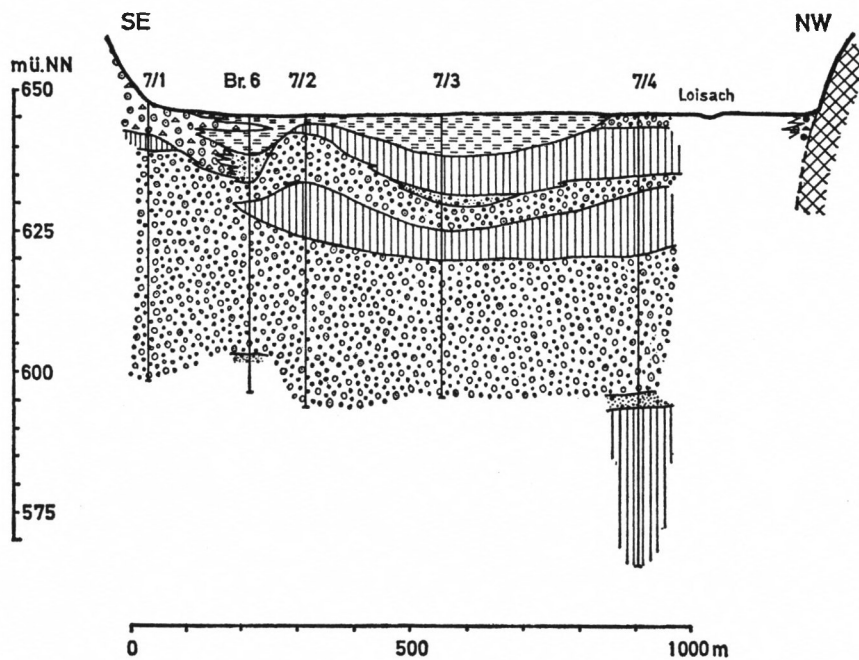
Abb. 16: Geologisches Querprofil III durch das Loisachtal (Legende s. Abb. 13).
