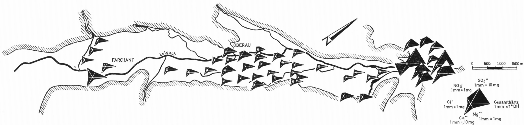
Abb. 28: Der Chemiesmus im 2. Grundwasserstockwerk.
