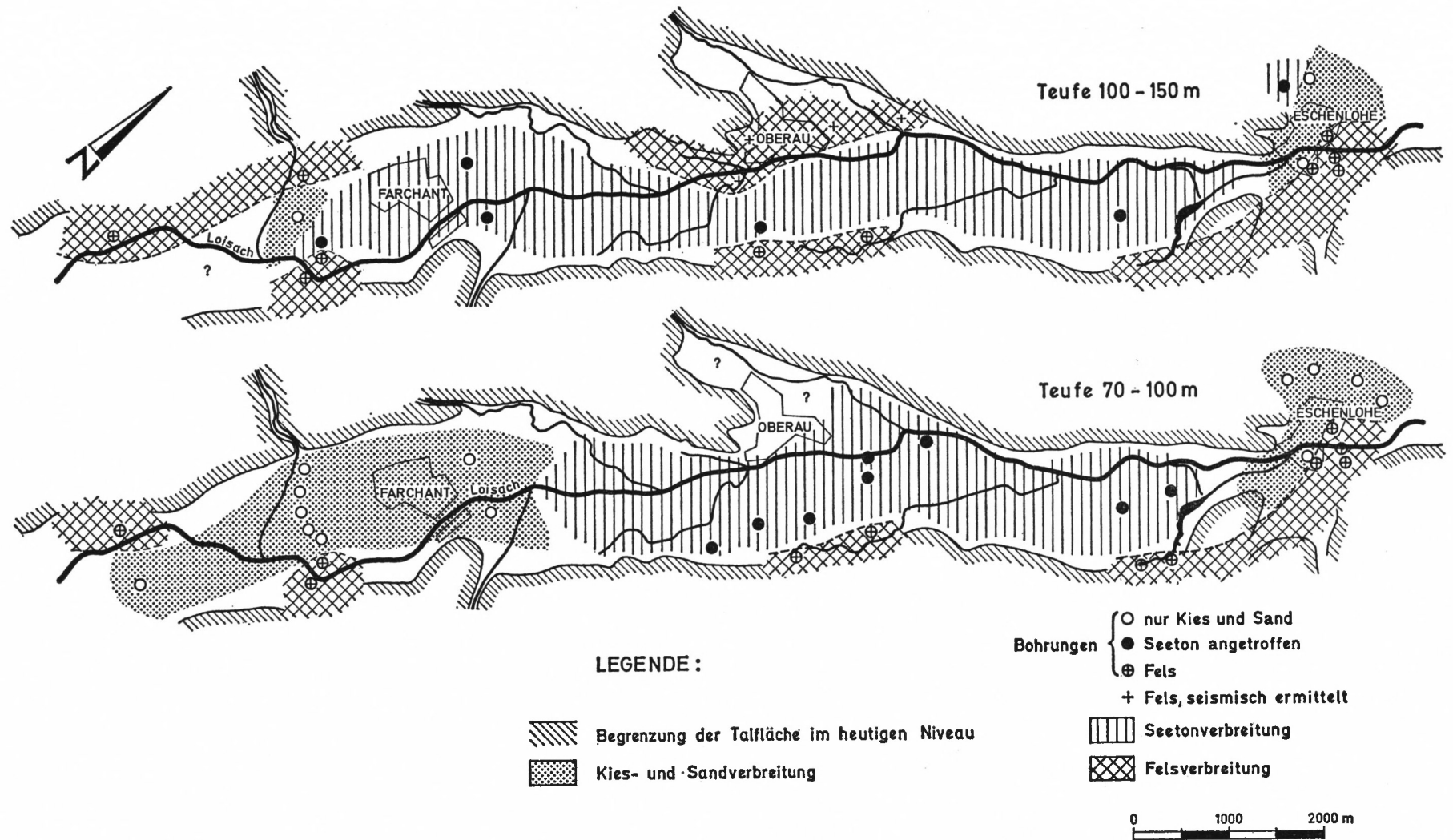
Abb. 17: Darstellung der Talauffüllung in Schichtpaketen; Teufen: 100-150 m und 70-100 m
