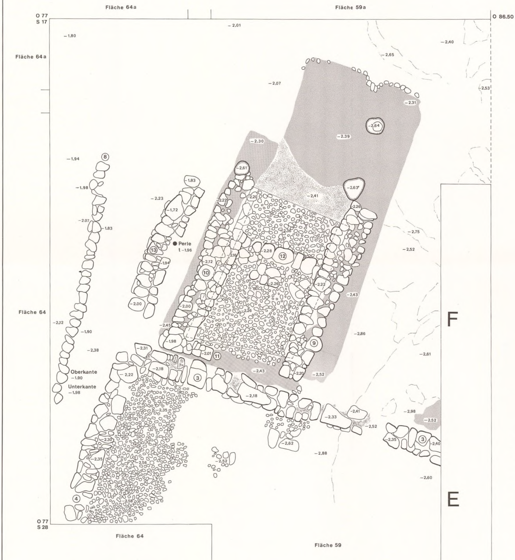
3 Nordwestteil von Holzhaus E und Gebäude F (Periode III). M. 1:50.
