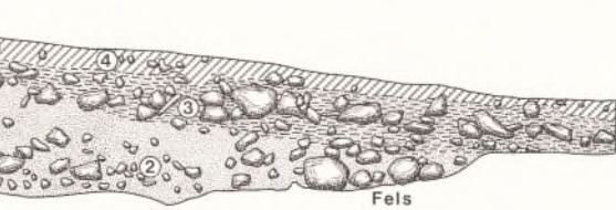
8 Fläche 72: Nordprofil.
