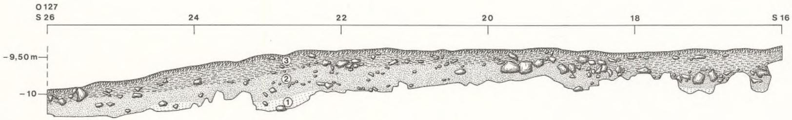
3 Fläche 71: Westprofil.
