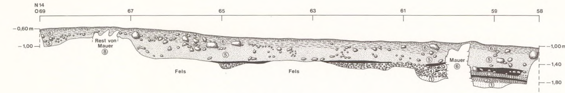
4 Fläche 28: Südprofil.
