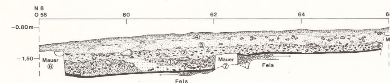
7 Fläche 20: Nordprofil.
