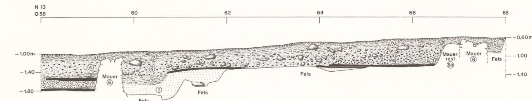
5 Fläche 23: Nordprofil.
