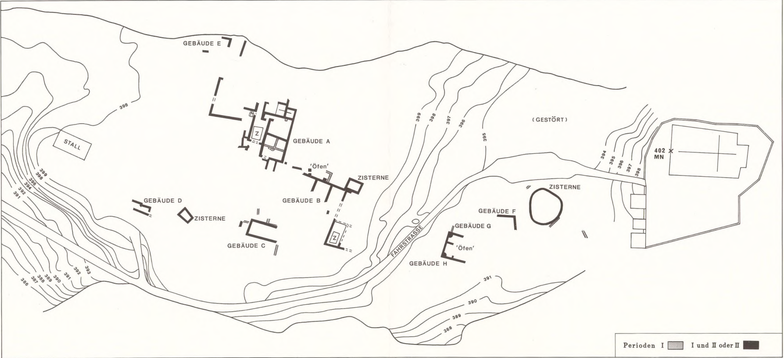
1 Bebauungsplan der Perioden I-II.
