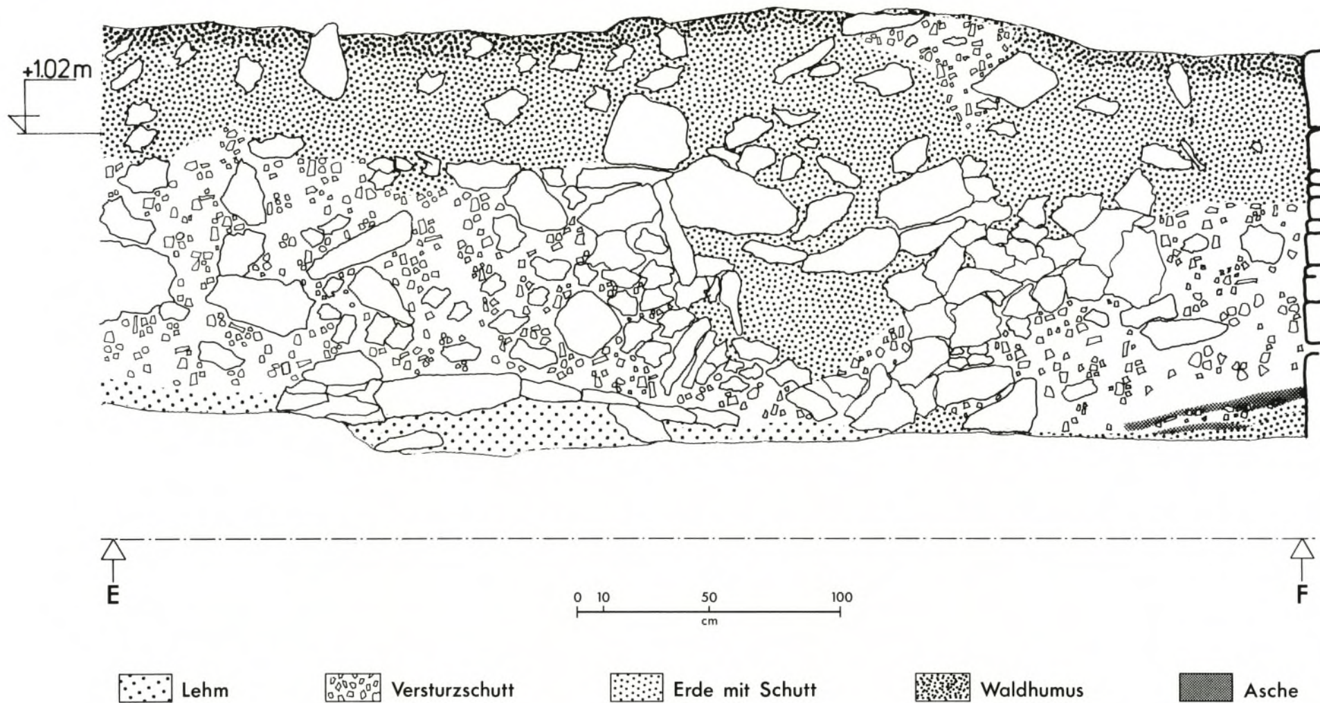
Abb. 17. Hrušica- Ad pirum . Straßen-Limestor, Innenprofil (Lage s. Beilage 4 B).
