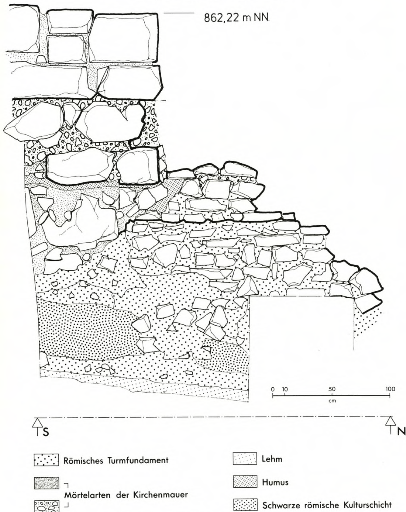
Abb. 15. Hrušica- Ad pirum . Schnitt X, Hangschnitt, S-N-Profil. Fundamentierungen für römischen Torturm und mittelalterliche Kirchenmauer. (Lage s. Abb. 13).
