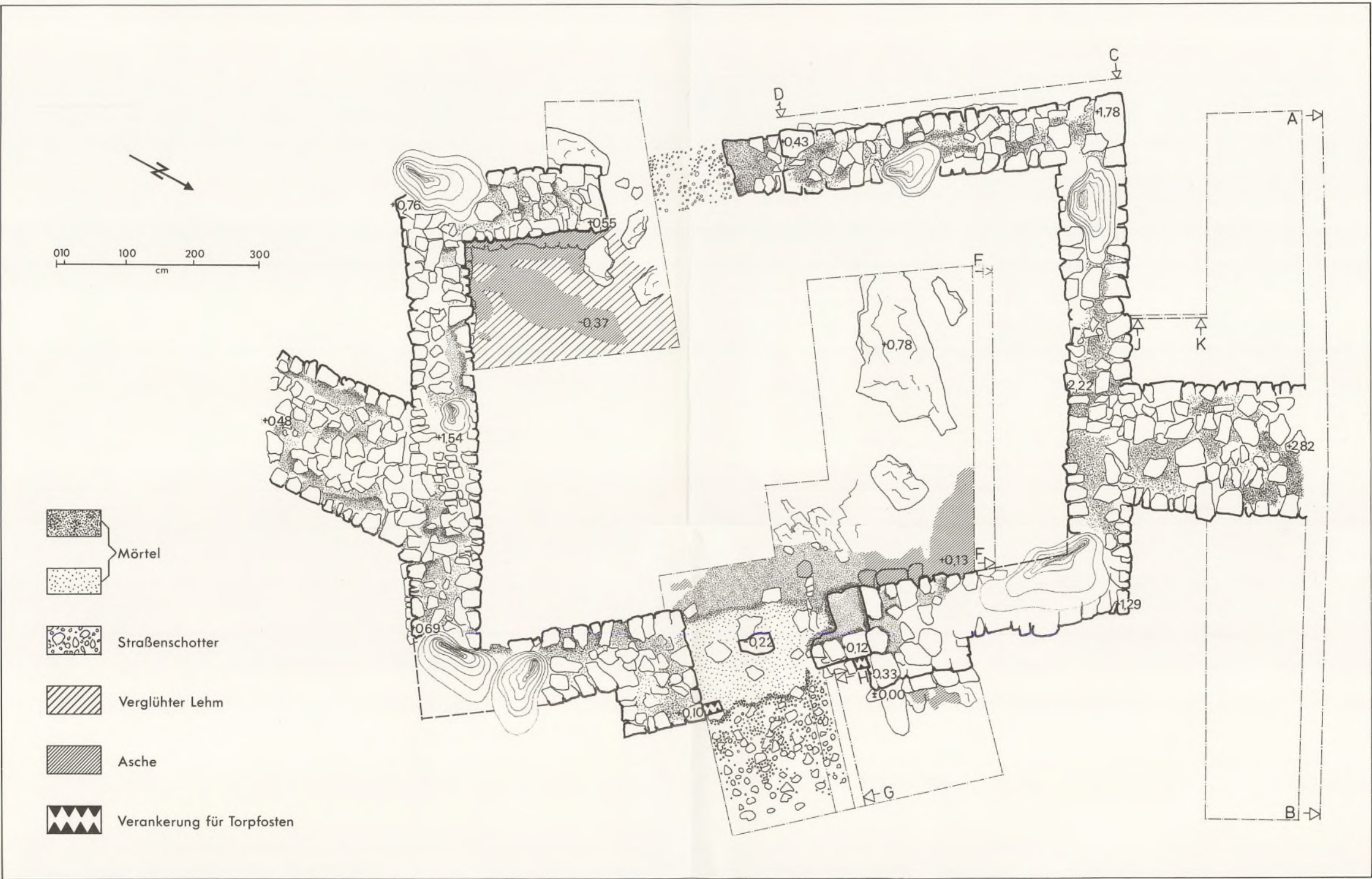
B. Hrušica-Ad pirum. Straßen-Limestor, Steinplan mit Lage der Profilschnitte.
