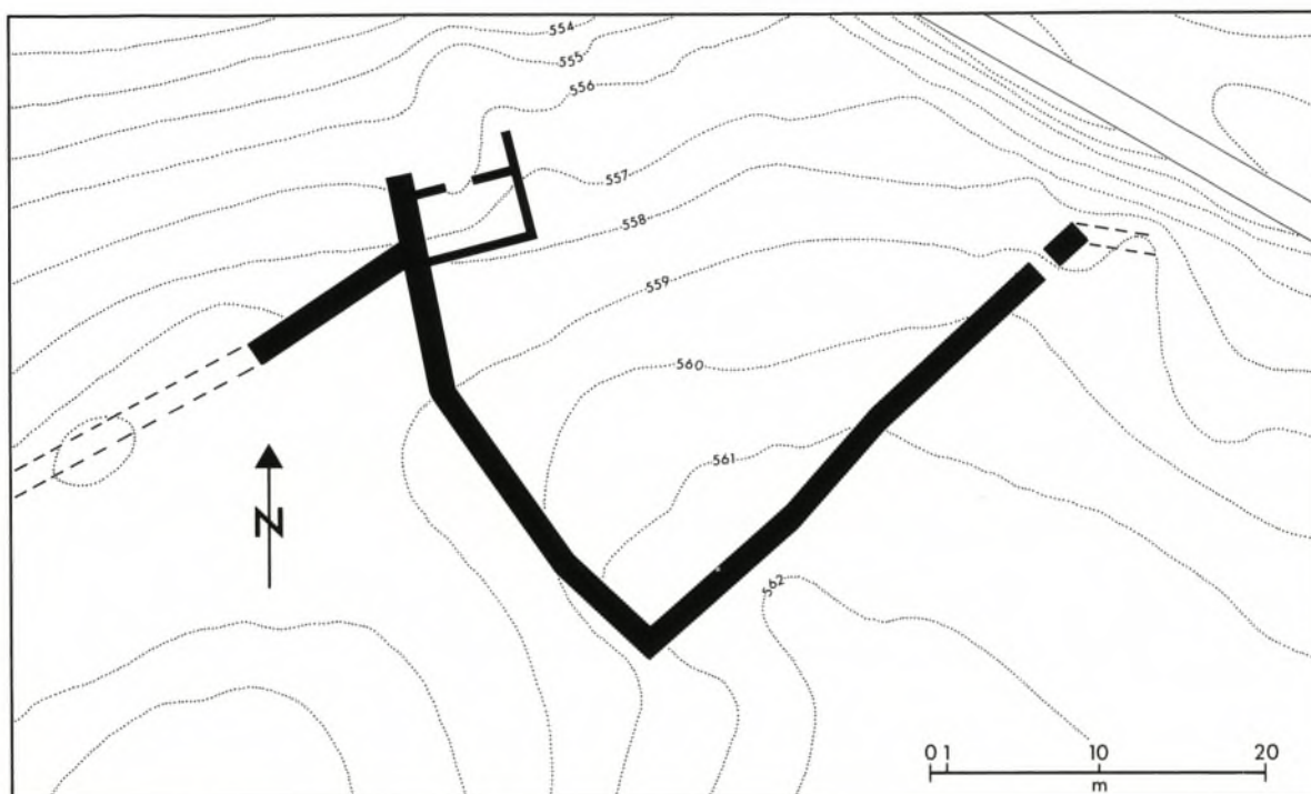
Abb. 5. Martinj hrib (Logatec). Spätantike Befestigungsanlage (nach Petru).
