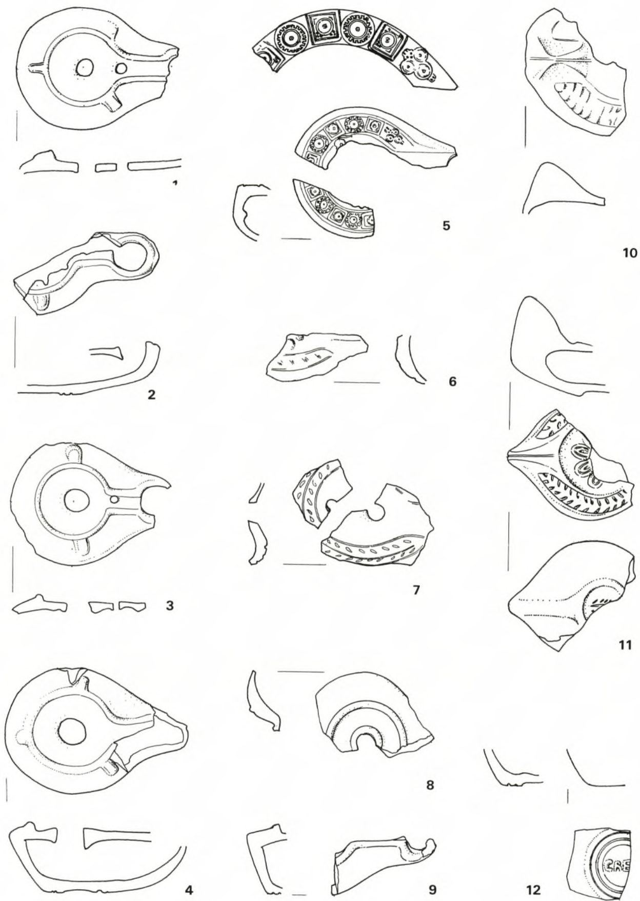
Öllampen: 1-4.9.12 Liste 35a; 5-8.10.11 Liste 35b. M. 1:2.
