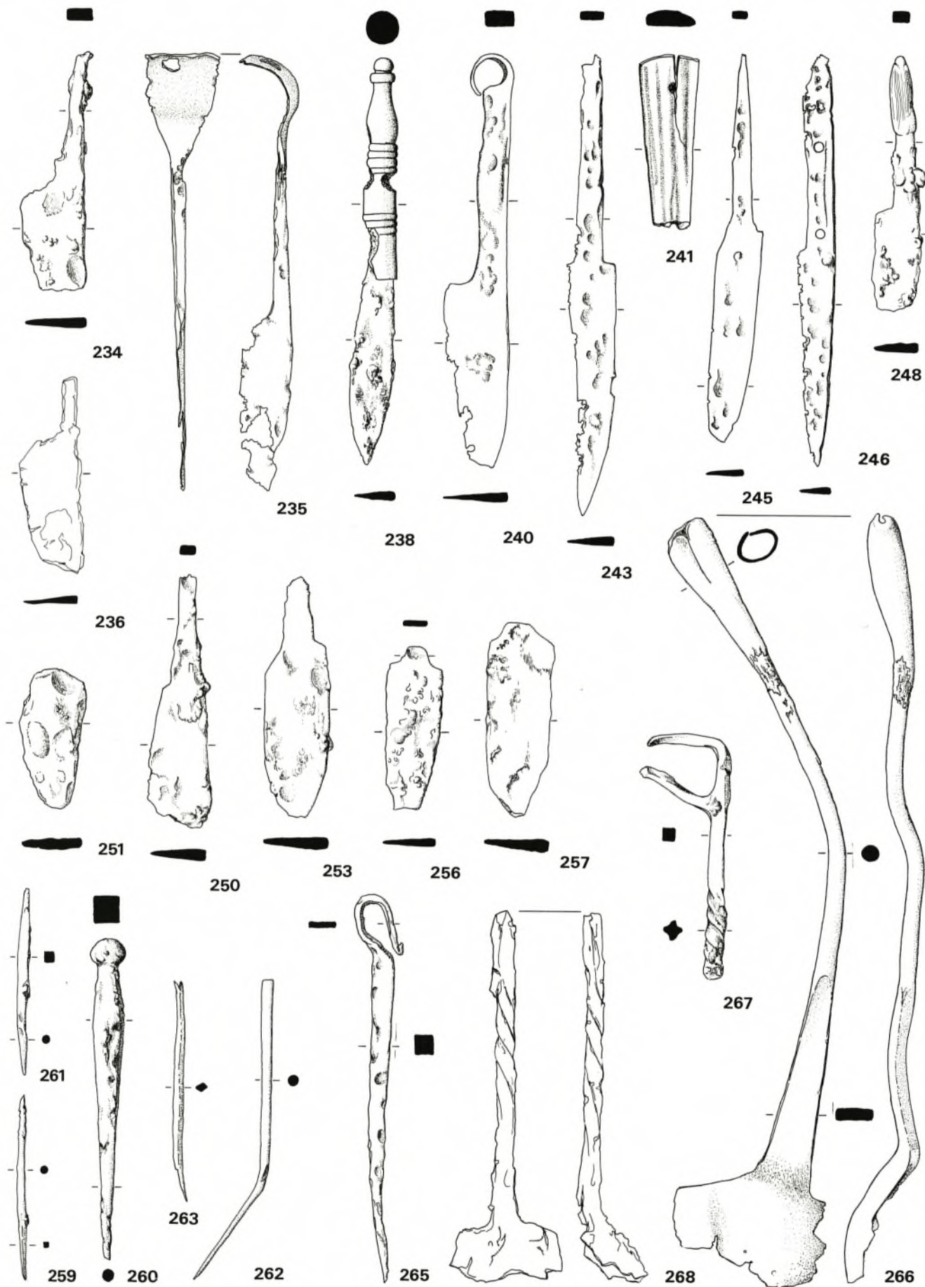
Scheren (Liste 18, 234–236), Messer (Liste 19a, 237–248), Messer mit breiter Klinge (Liste 19b, 249–257), Pfrieme (Liste 20, 258–265), Küchengerätschaften (Liste 21, 266–269). M. 1:2.
