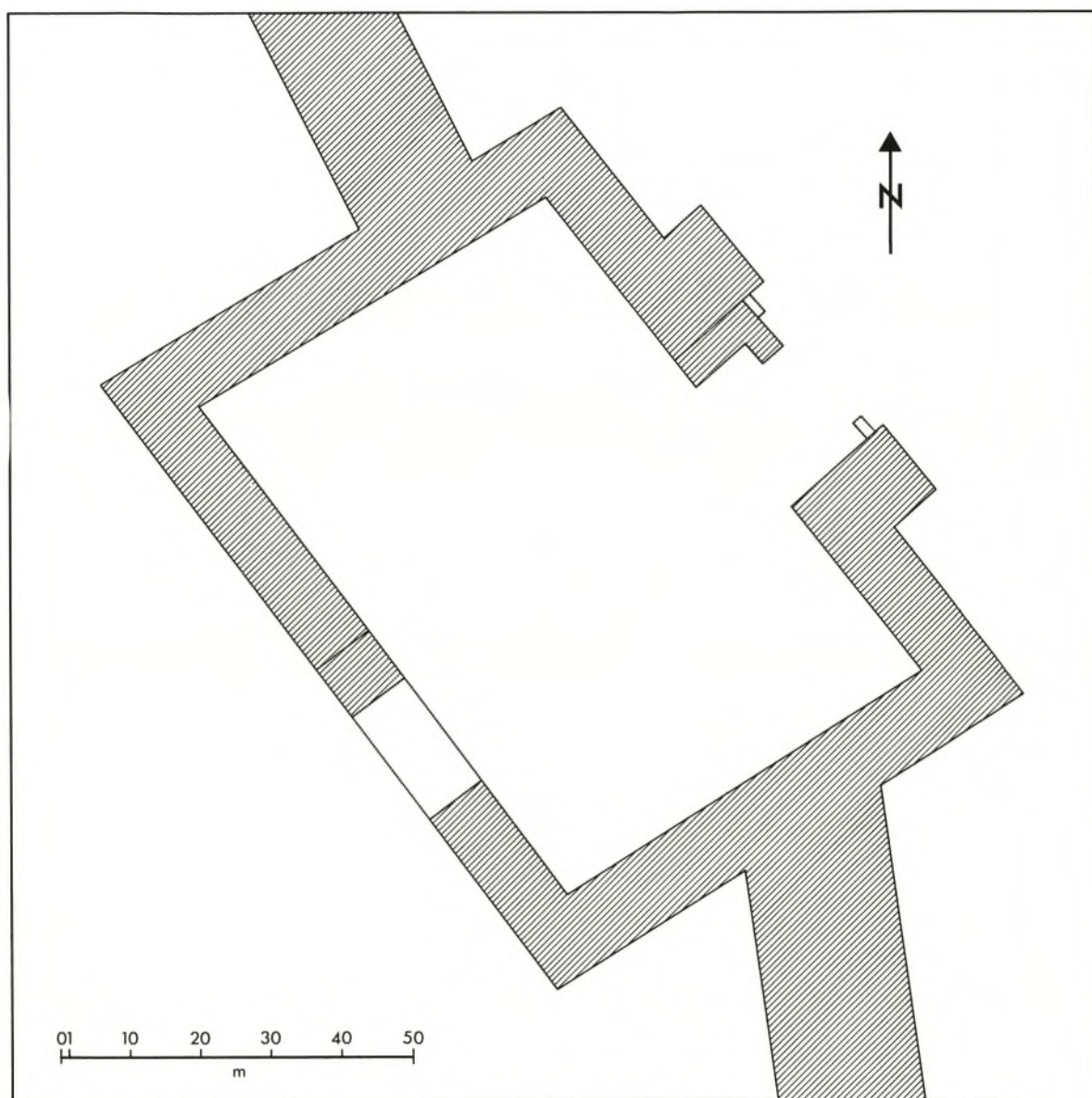
Abb. 19. Hrušica-Ad pirum. Straßen-Limestor, Grundriß.
