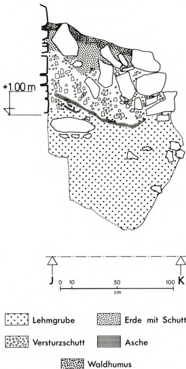
Abb. 18. Hrušica-Ad pirum. Straßen-Limestor, Außenprofil (Lage s. Beilage 4 B).
