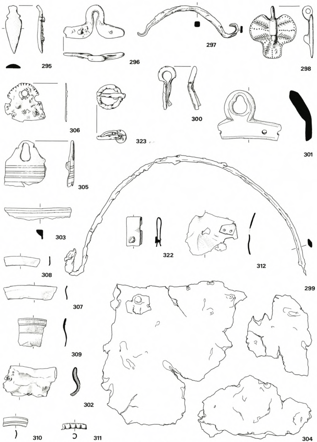
Metallgefäßteile und Metallbeschläge von Holzbehältern (Listen 24, 25, 295–324; Fortsetzung Taf. 28). M. 1 : 2.
