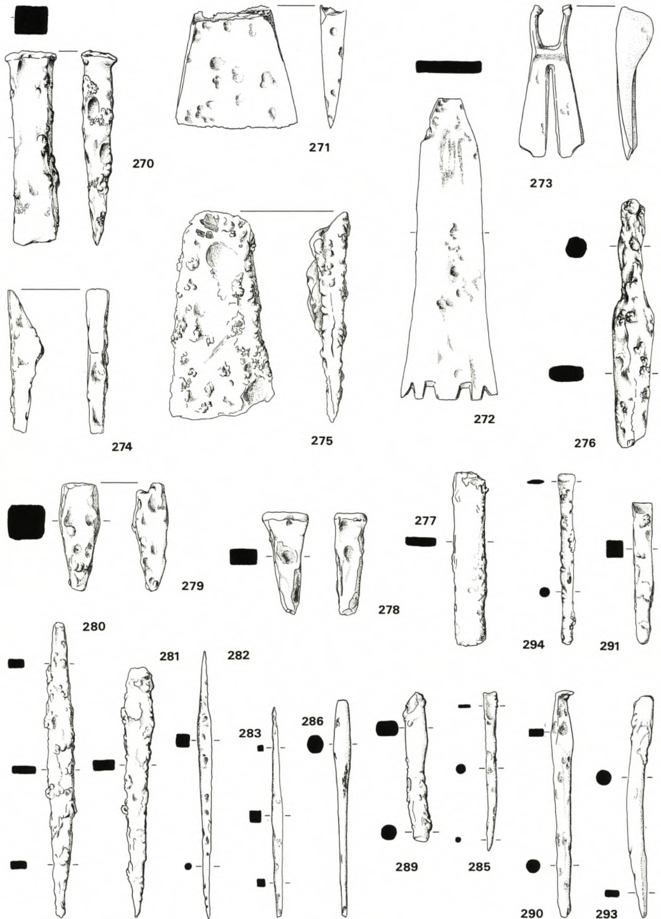
Werkzeuge zur Holzbearbeitung (Liste 22, 270–277) und Metallbearbeitung (Liste 23a, 278–281), Durchschläge (Liste 23b, 282–292), Flachmeißel (Liste 23c, 293, 294). M. 1:2.
