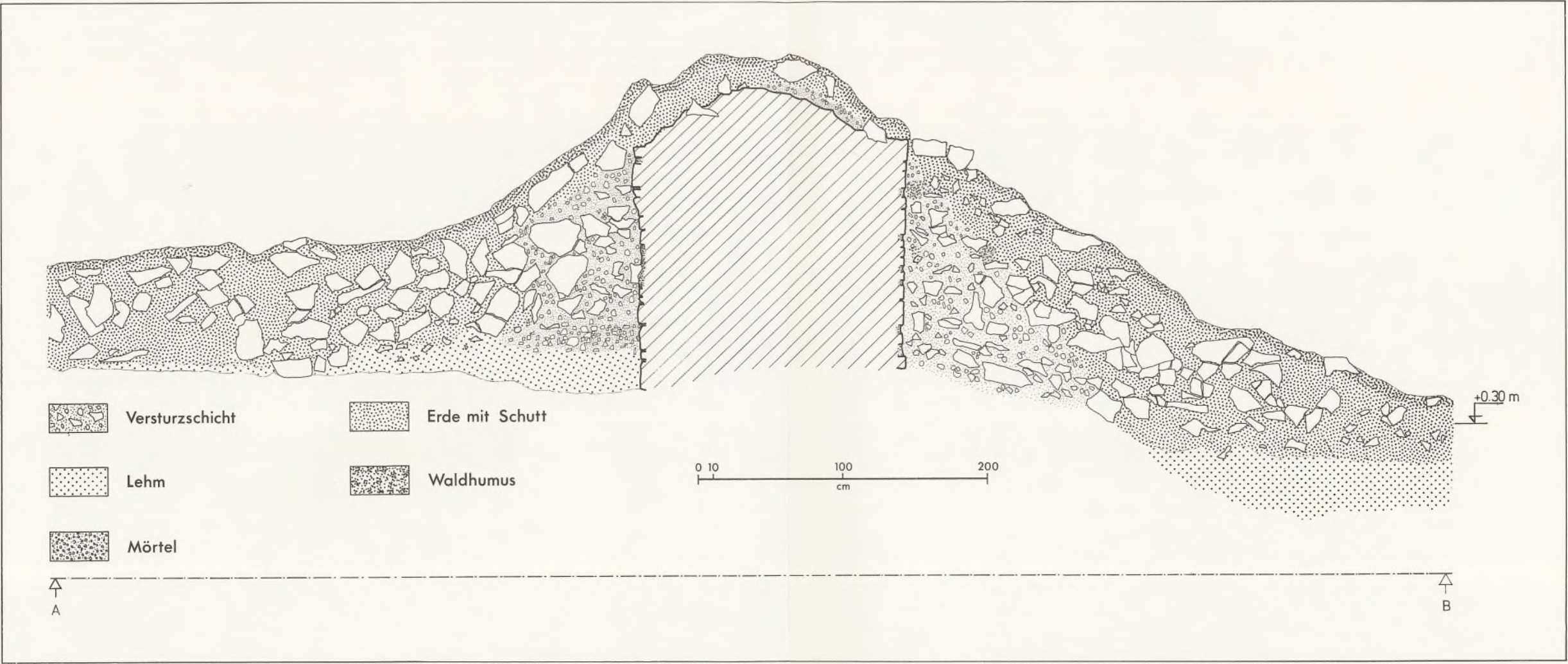
C. Hrušica-Ad pirum. Straßen-Limestor, Schnitt durch die Sperrmauer (Lage s. Beilage 4 B).
