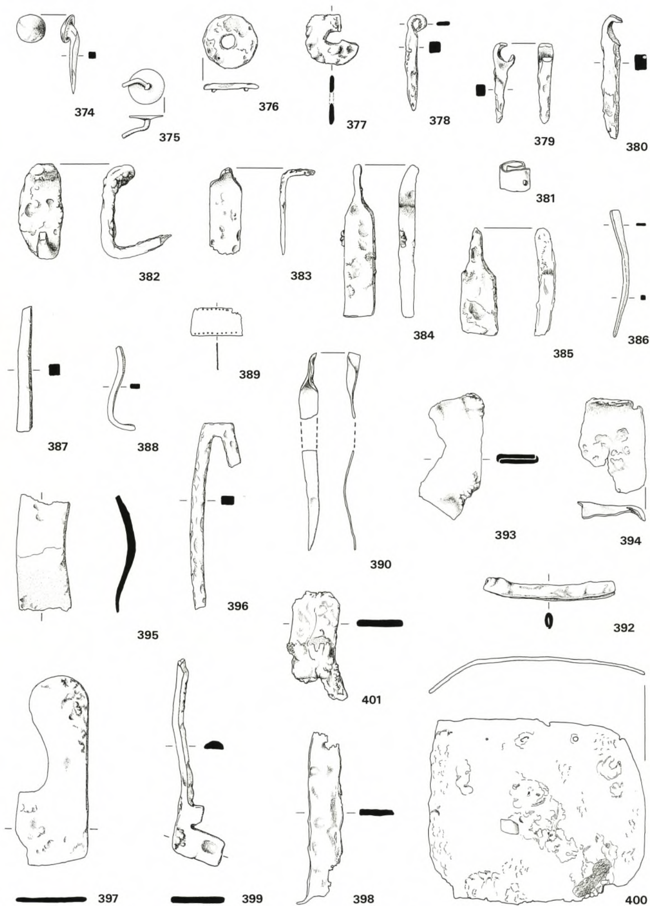
Niete und Nietscheiben (Liste 37,372-377), Geräte unbekannter Funktion und Fragmente (Liste 38,39,378-401). M. 1:2.
