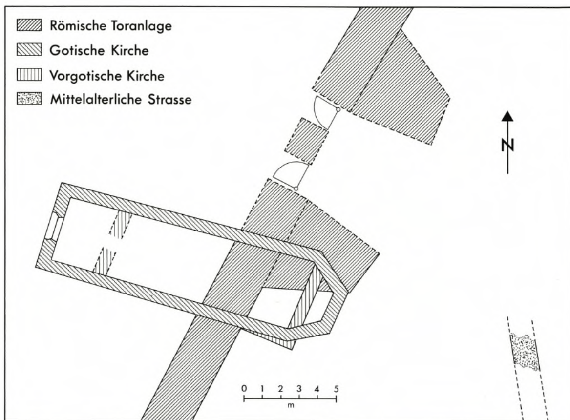
Abb. 14. Hrušica-Ad pirum. Schnitt X, Rekonstruktion der Architekturbefunde.
