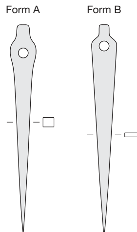
Abb. 122. Kopfformen A und B römischer Zeltheringe mit Öse. Die Ringe in den Ösen sind nicht dargestellt. – M. ca. 1:3.
