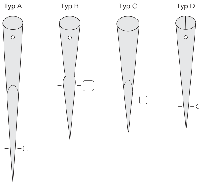
Abb. 99. Septimer. Typologie eiserner Lanzenschuhe. – Typ A mit vierkantiger, lang ausgezogener Spitze. Typ B mit vierkantiger, leicht abgesetzter Spitze. – Typ C mit vierkantiger, nicht abgesetzter Spitze. Typ D mit runder, nicht abgesetzter Spitze. – M. ca. 1:3.
