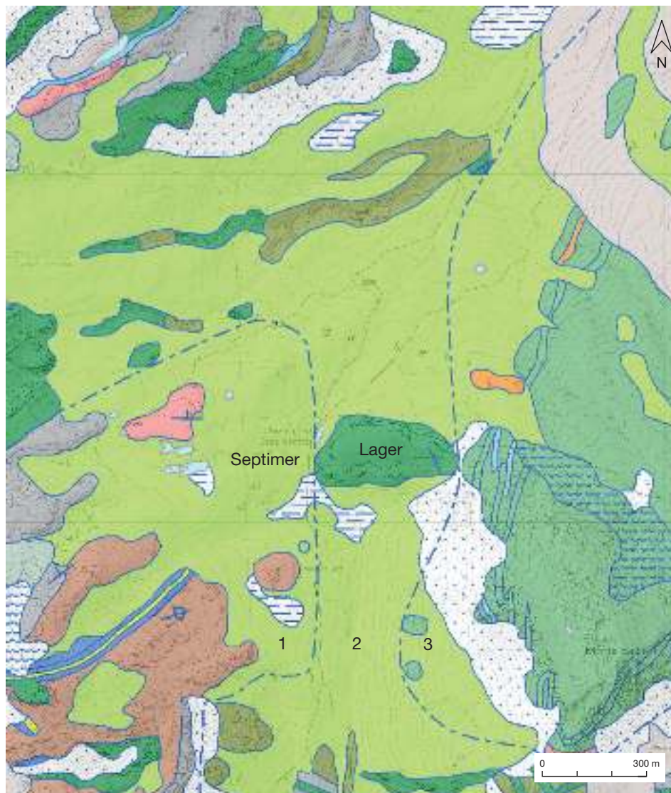
Abb. 8. Geologische Karte des Gebietes im Bereich des Septimerpasses. Ausschnitt der Karte M. 1:10.000. Hellgrün = Moräne; dunkelgrün = Grünschiefer, Amphibolith. – 1 Margna-Decke (Gneis, Glimmerschiefer). 2 Platta-Decke (Ophiolithe). – 3 Err-Decke (Sedimentgesteine). – Blaue gestrichelte Linien = Deckengrenzen. M. ca. 1:15.000.
