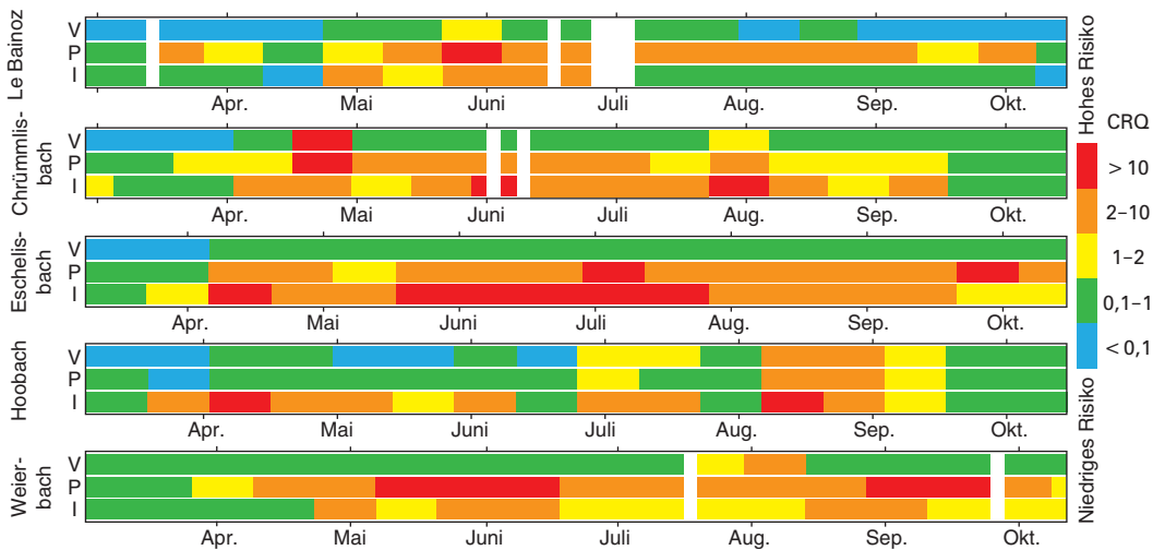
Abb. 3. Chronische Mischungsriskquotienten ( CRQ_{mix} ) der gemessenen Konzentrationen an Pflanzenschutzmitteln (14-Tages-Mischproben) an den NAWA-SPEZ-2017-Probenahmestellen. V: Vertebraten (v. a. Fische), P: Pflanzen, I: Invertebraten; weiße Abschnitte: keine Proben konnten genommen werden; Farben: Höhe des RQ für die jeweilige Organismengruppe und den Zeitraum. – Junghans et al. 2019.
