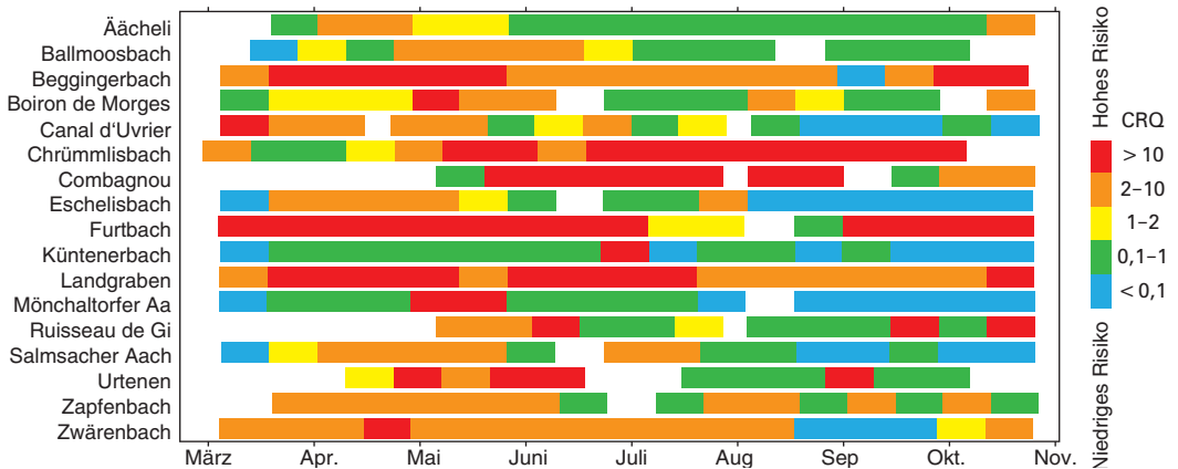
Abb. 4. Chronische Mischungsrisikoquotienten ( CRQ_{mix} ) der gemessenen Konzentrationen an Pyrethroid- und Organophosphat-Insektiziden (14-Tages-Mischproben von März bis Oktober 2019) an 17 Probenahmestellen. Farben: Höhe des CRQ_{mix} für aquatische Organismen für den jeweiligen Zeitraum. – Nach Daouk et al. 2022.
