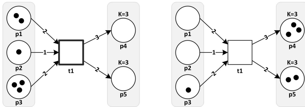
Abbildung 2.6: Stellen/Transitions-Netz: (links) vor dem Schrittvorgang und (rechts) nach dem Schrittvorgang
