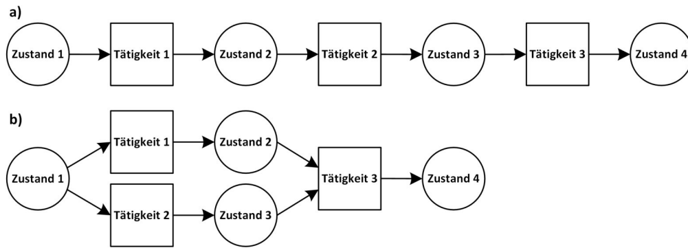
Abbildung 2.1: a) Sequenzieller Prozess b) Nebenläufiger Prozess
