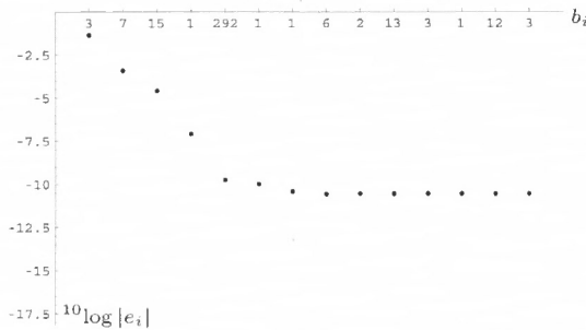
Abb. 1. ^{10}\log -Fehler-Graph für den Kettenbruch zum Näherungswert 31415926535/10000000000
