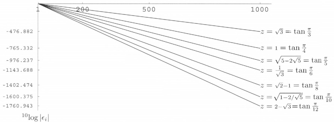
Abb. 9. ^{10}\log -Fehler-Graphen des Lambertschen \arctan z -Kettenbruchs für einige Werte von z
