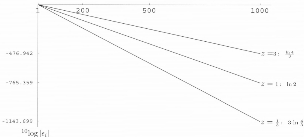
Abb. 10. {}^{10}\log -Fehler-Graphen des Gaußschen Kettenbruchs \ln(1+z)/z = F(1,1; 2; -z) für einige Werte von z
