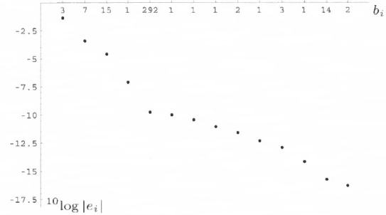
Abb. 2. ^{10}\log -Fehler-Graph für die ersten 14 Terme des banal entwickelten \pi -Kettenbruchs
