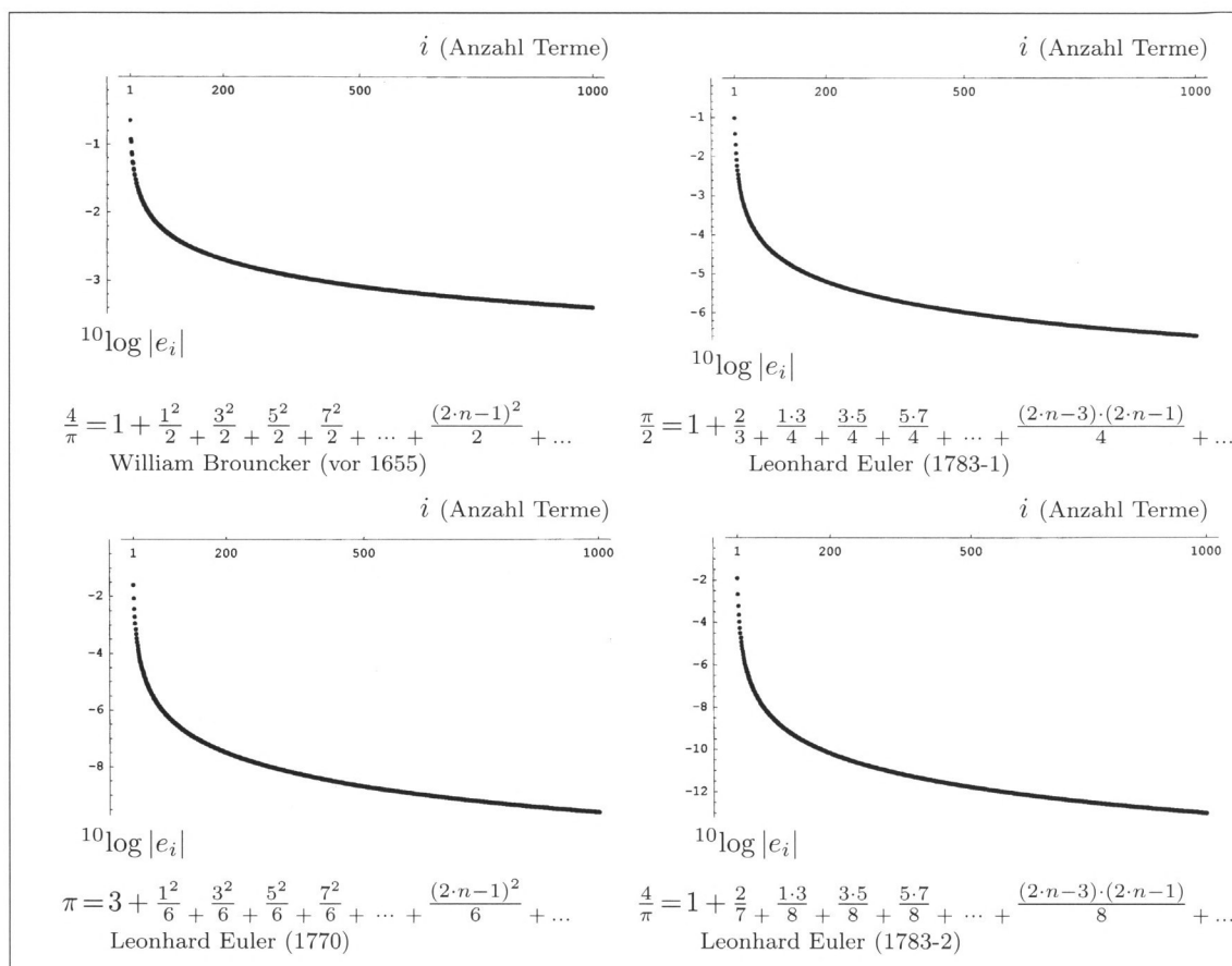
Abb. 5. Kettenbrüche, deren 10 \log |e_i| -Graph logarithmische Konvergenz anzeigt.
