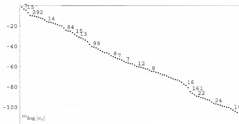
Abb. 3. 10 \log -Fehler-Graph für die ersten 100 Terme des banal entwickelten \pi -Kettenbruchs. Grob-linearer Verlauf, nach der ‘Metrischen Theorie’ von Alexander Khintchine (1894–1959).
