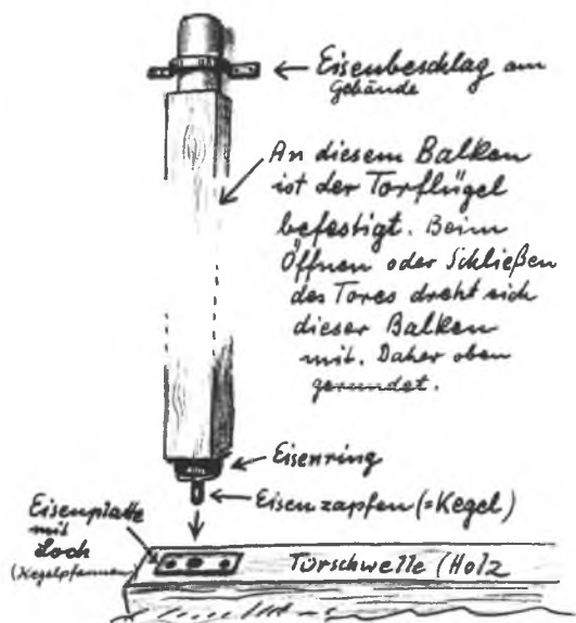
Abb. 11: Kegelpfanne als Kegellager in der Tür- od. Torschwelle (Gottfrieding DGF).
