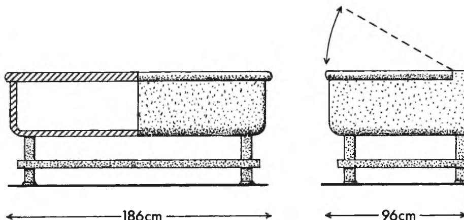
Abb. 9: Truhenbett (Vorderansicht, Seitenansicht) aus Wölkham WS, nach Volkswerk. Jb. des Staatlichen Museums für Dt. Vkde 1943, Jena 1944, 196.
