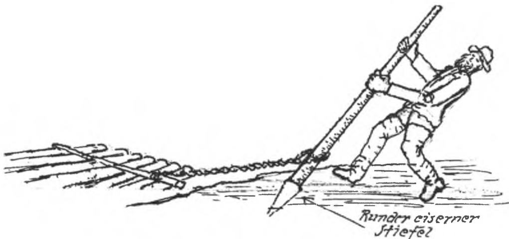
Abb. 10: Hakenpfahl mit 8 bis 10 m langem Seil zum Länden des Floßes (Reichersbeuern TÖL).
