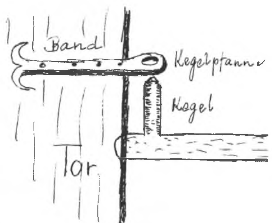
Abb. 12: Kegelpfanne als Halterung für Türen u. Tore (Altenbuch LAN).
