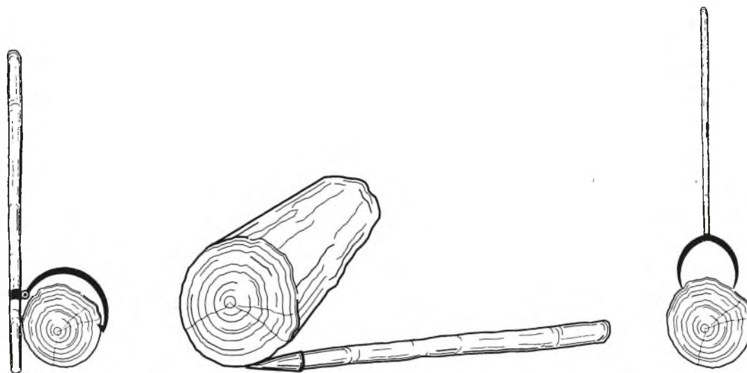
Abb. 2: Beißer (Hebelstange mit Eisenschuh, Krallen od. Zange) aus Künzing VOF, Altenbuch LAN, Ering PAN.
