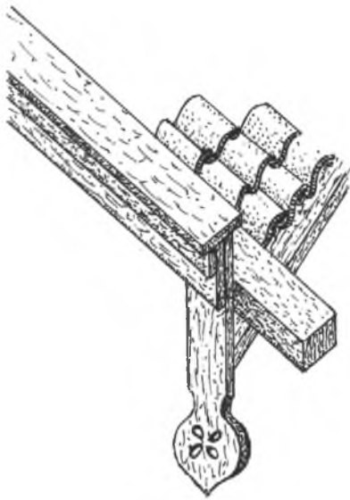
Abb. 23: Furmblatl 'geschnitztes Zierbrett am Ortgang', nach BRUNNER Samerbg I10.
