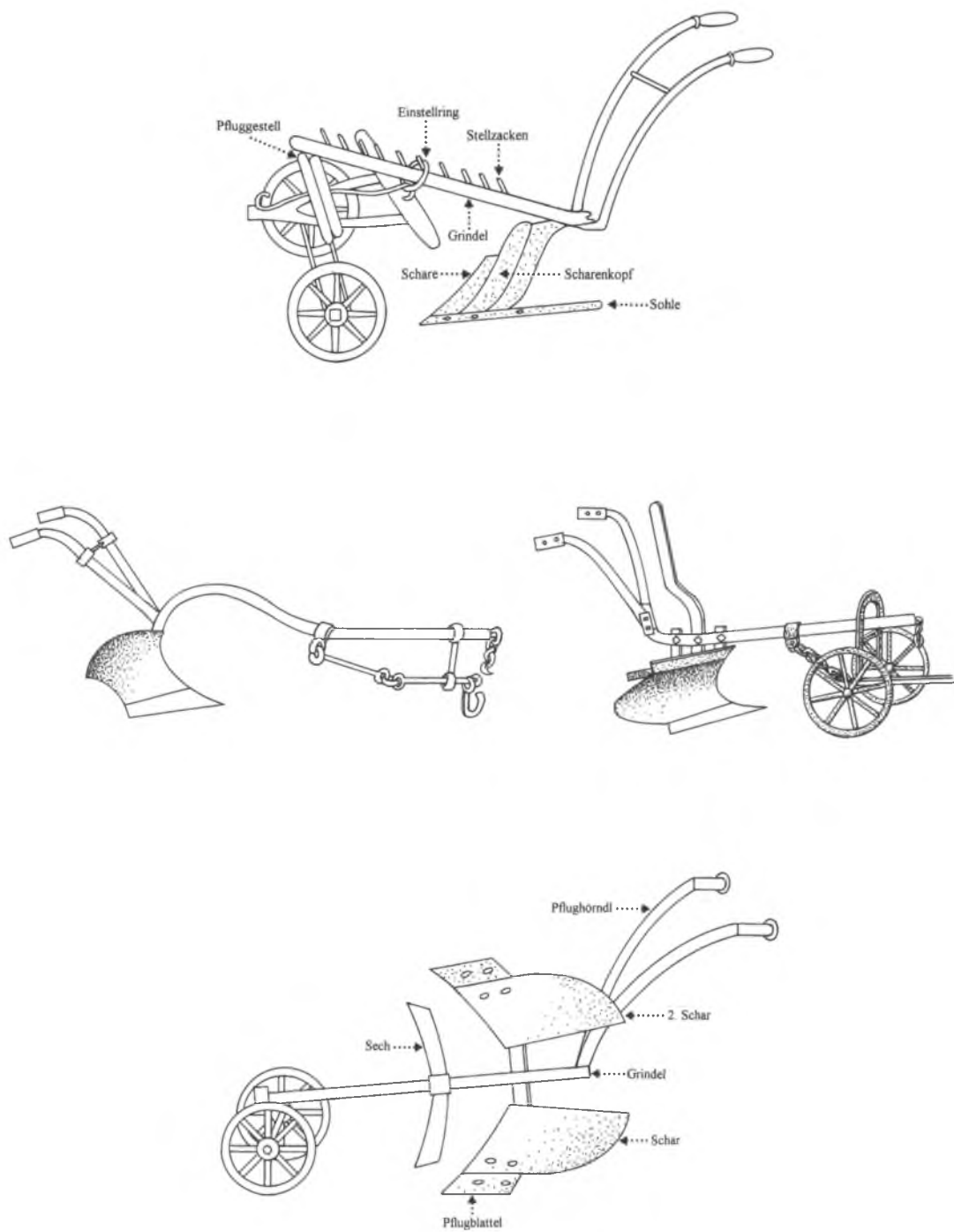
Abb. 17: (Oben) einfacher Pflug (Weissenburg), (Mitte links) einschariger Schwingpflug u. (Mitte rechts) Drehpflug mit wendbarer Schar (Kehseon EBE), (unten) Drehpflug mit zwei Scharen (Hirnsbg RO).
