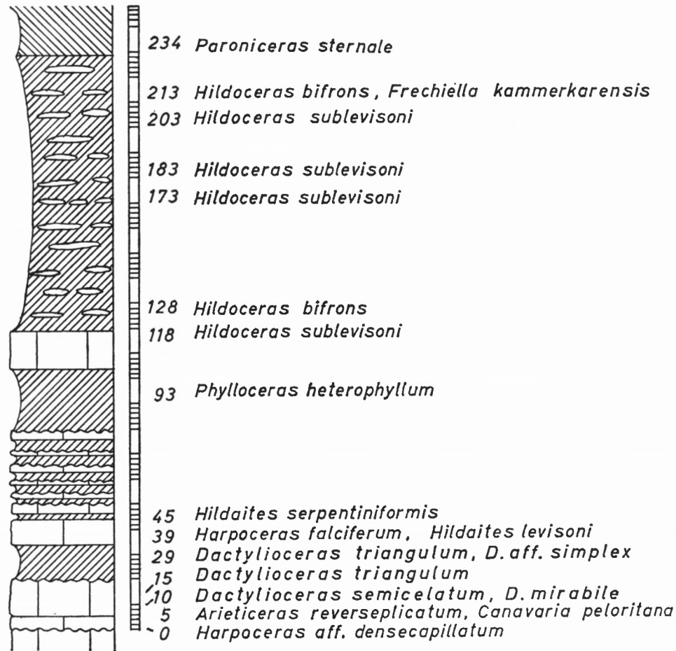
Abb 1. Profil Scheibelberg. – Die Zahlen geben die Lage der Fundniveaus in Zentimetern über der Basis des Profils an. Zur Wiedererkennung des Profils Scheibelberg im Gelände dient der Geländeknick an der Grenze der aus Kalkbänken aufgebauten Felsenkanzel zu den überlagernden, mehr mergeligen und daher mäßiger geböschten Schichten; er befindet sich im Niveau 20.
