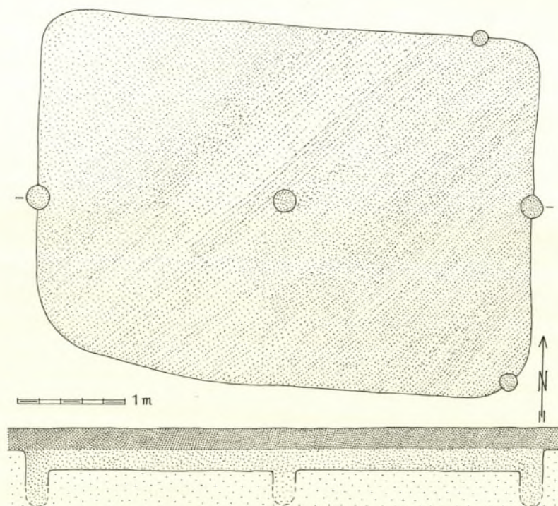
Abb. 3. Dingolshausen (18). Hausgrundriß mit Profil. M. 1:50.
