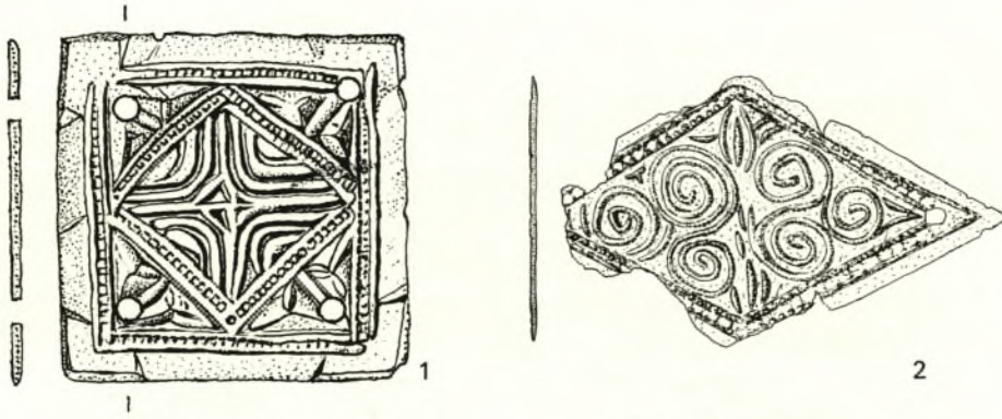
Abb. 16. 1 Frankenwinheim (29); 2 Düllstadt (22). Bronze. M. 1:1.
