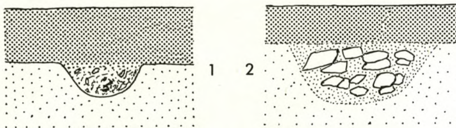
Abb. 6. Altendorf (1): 1 Brandgrube 33; 2 Brandgrube 39. M. 1:20.
