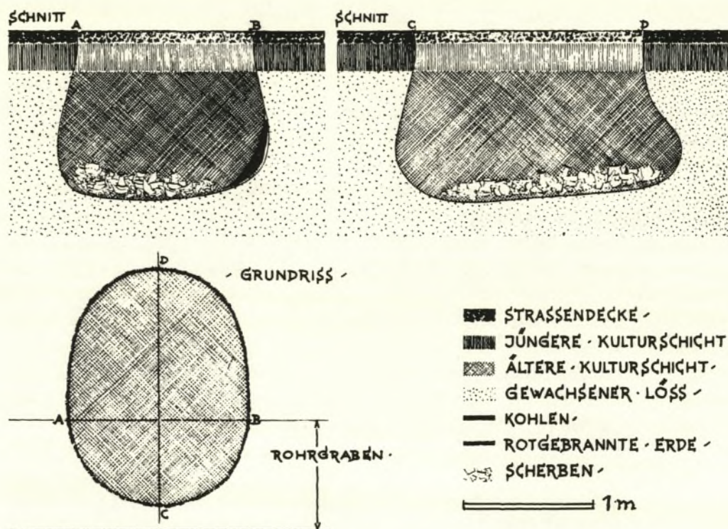
Abb. 4. Eßleben (28). Grube mit der Terra-nigra-Keramik (Taf. 67). M. 1:50
