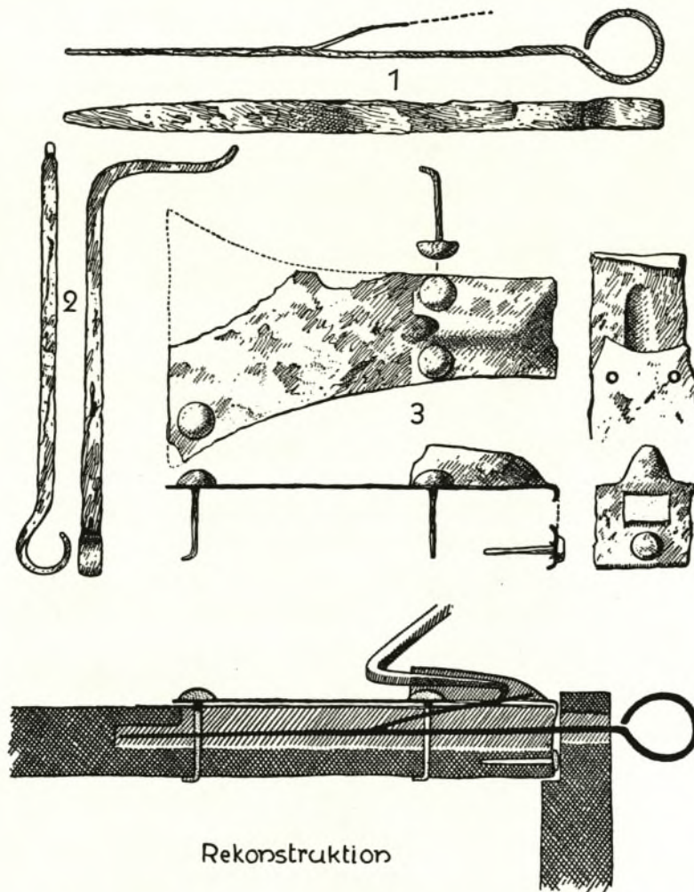
Abb. 20. Eiserne Schloßbestandteile von Wetzendorf, Kr. Querfurt. Nach W. Schulz. M. 1:2.
