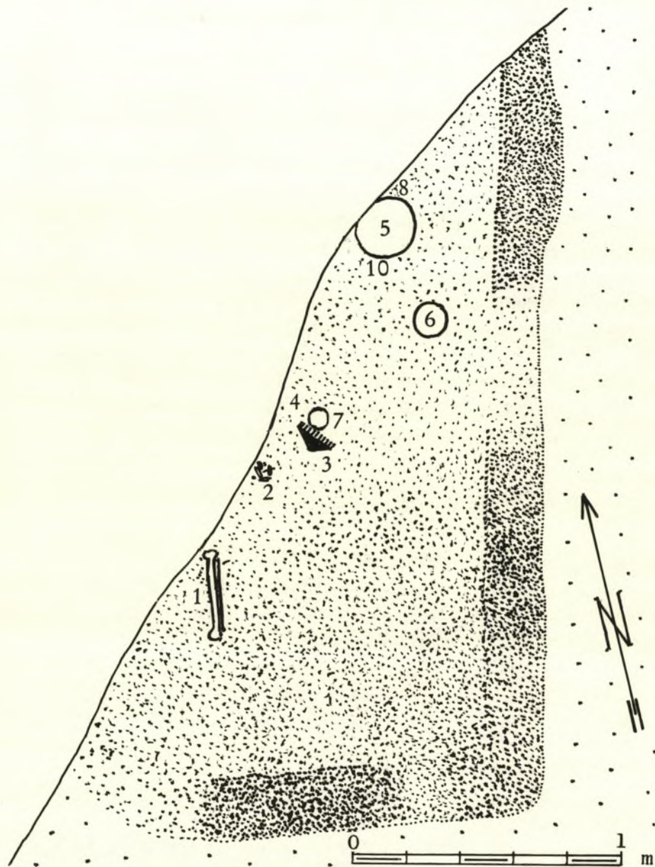
Abb. 8. Altendorf (1) Körpergrab 74 (Taf. 10) M. 1:20.
