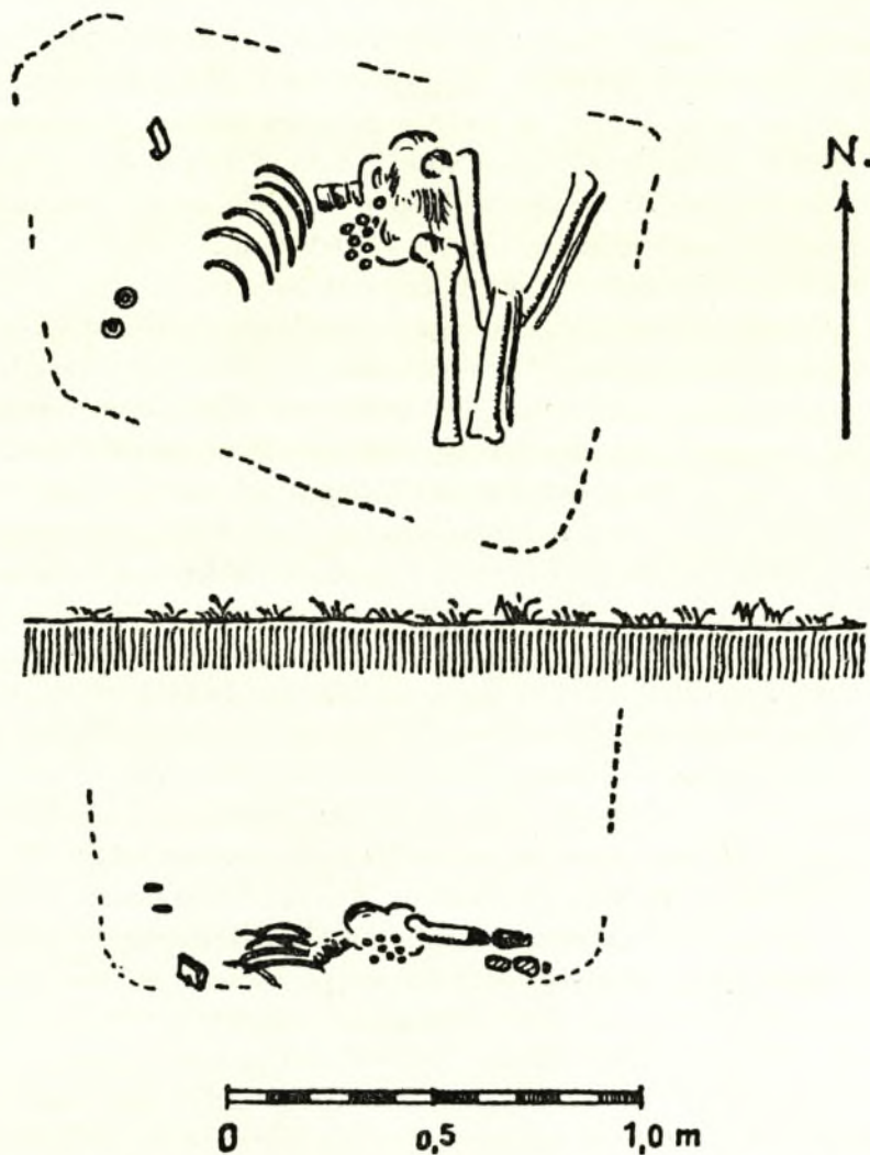
Abb. 19. Grabplan (nach H. Neubauer) von Otzing (141). M. 1 : 20.
