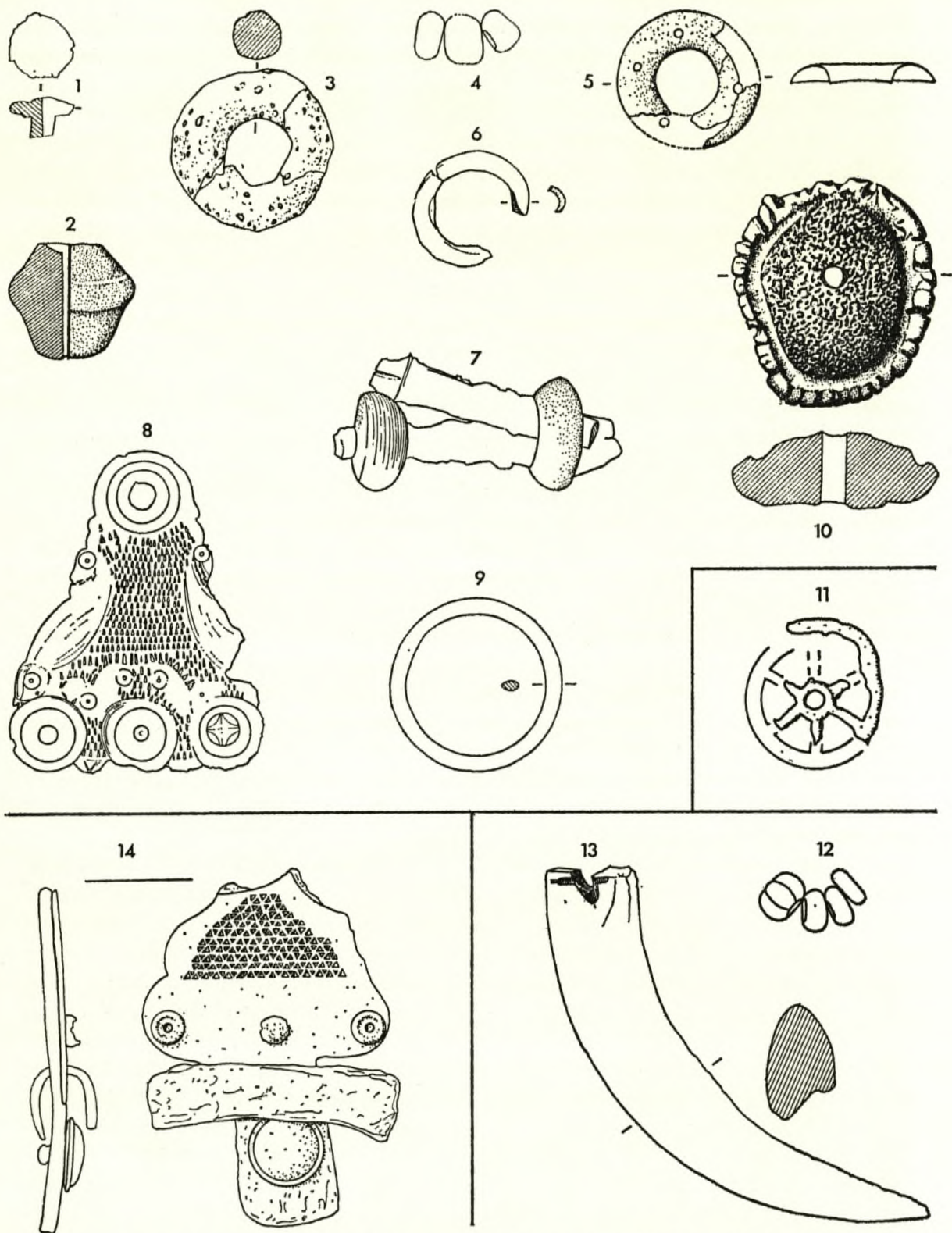
Abb. 9. 1-10 Münsingen (2) Grab 6; 11 Münsingen (2) Grab 27; 12-13 Münsingen (2) Grab 1; 14 Ensérune (Hérault). - 4 Glas; 12 Glas und Bernstein; 6 Hirschhorn; 13 Tierzahn; 7 Eisen, Knochen und Bronze; 2, 3 Ton; 1 Eisen; sonst Bronze. M. 3 : 4.
