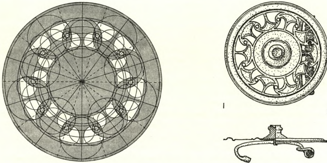
Abb. 22. Die Scheibenfibel vom Dürrnberg bei Hallein Grab 42/1 und ihre geometrische Konstruktion. Fibel M. 1 : 1.
