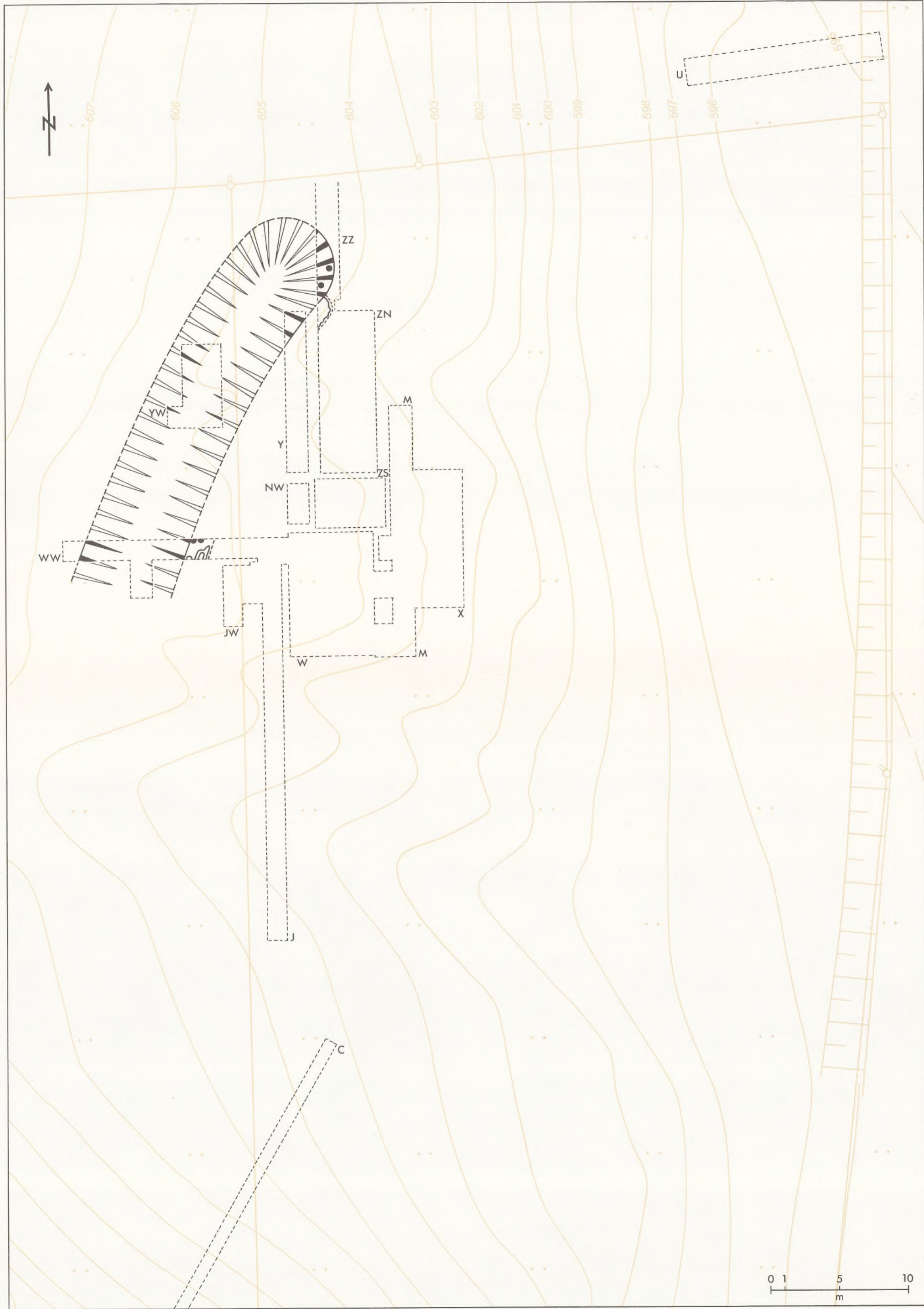
Goldberg, Gemeinde Türkheim, Lkr. Unterallgäu · Bronzezeit. Maßstab 1: 250.
