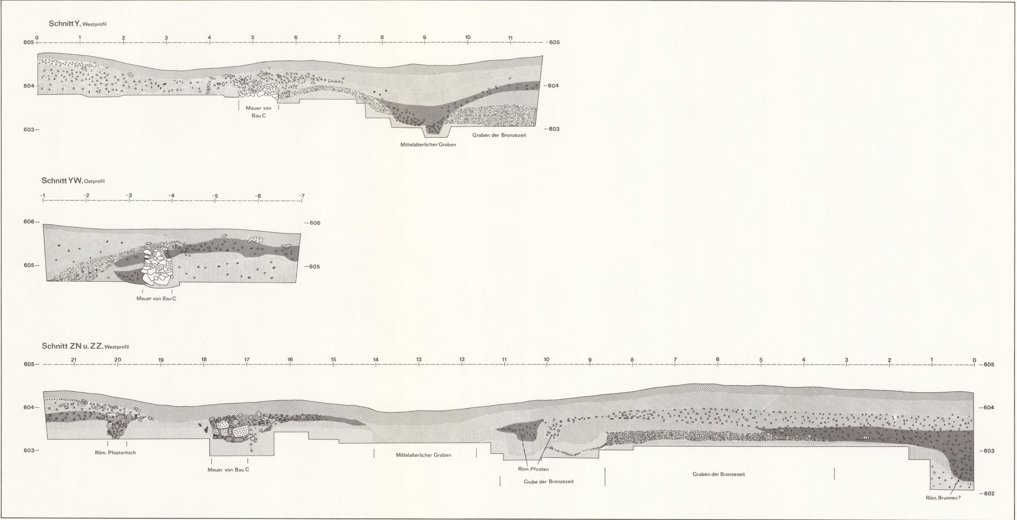
Goldberg, Gemeinde Türkheim, Lkr. Unterallgäu · Profile Schnitte Y, YW und ZN-ZZ. Maßstab 1:50.
