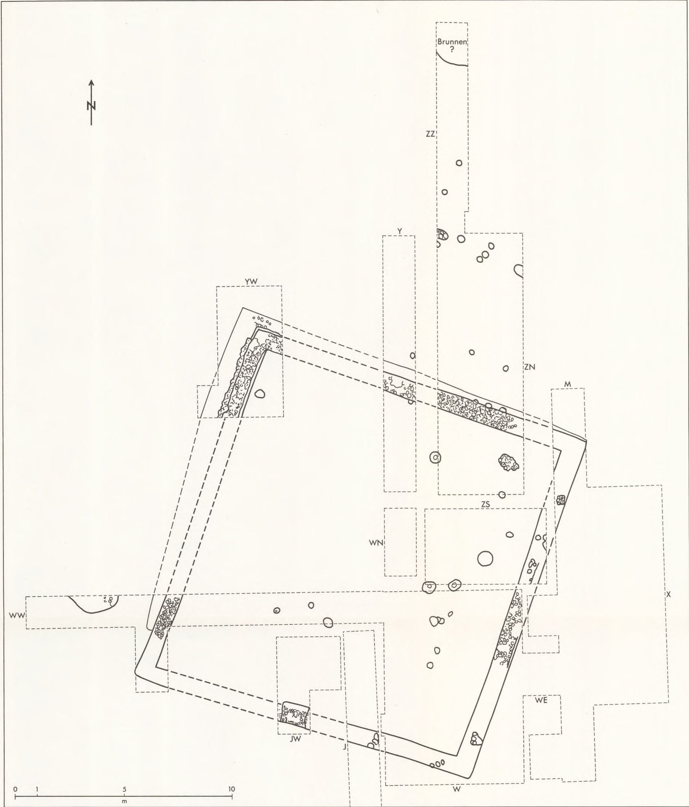
Goldberg, Gemeinde Türkheim, Lkr. Unterallgäu · Bau C der spätrömischen Befestigung. Maßstab 1:100.
