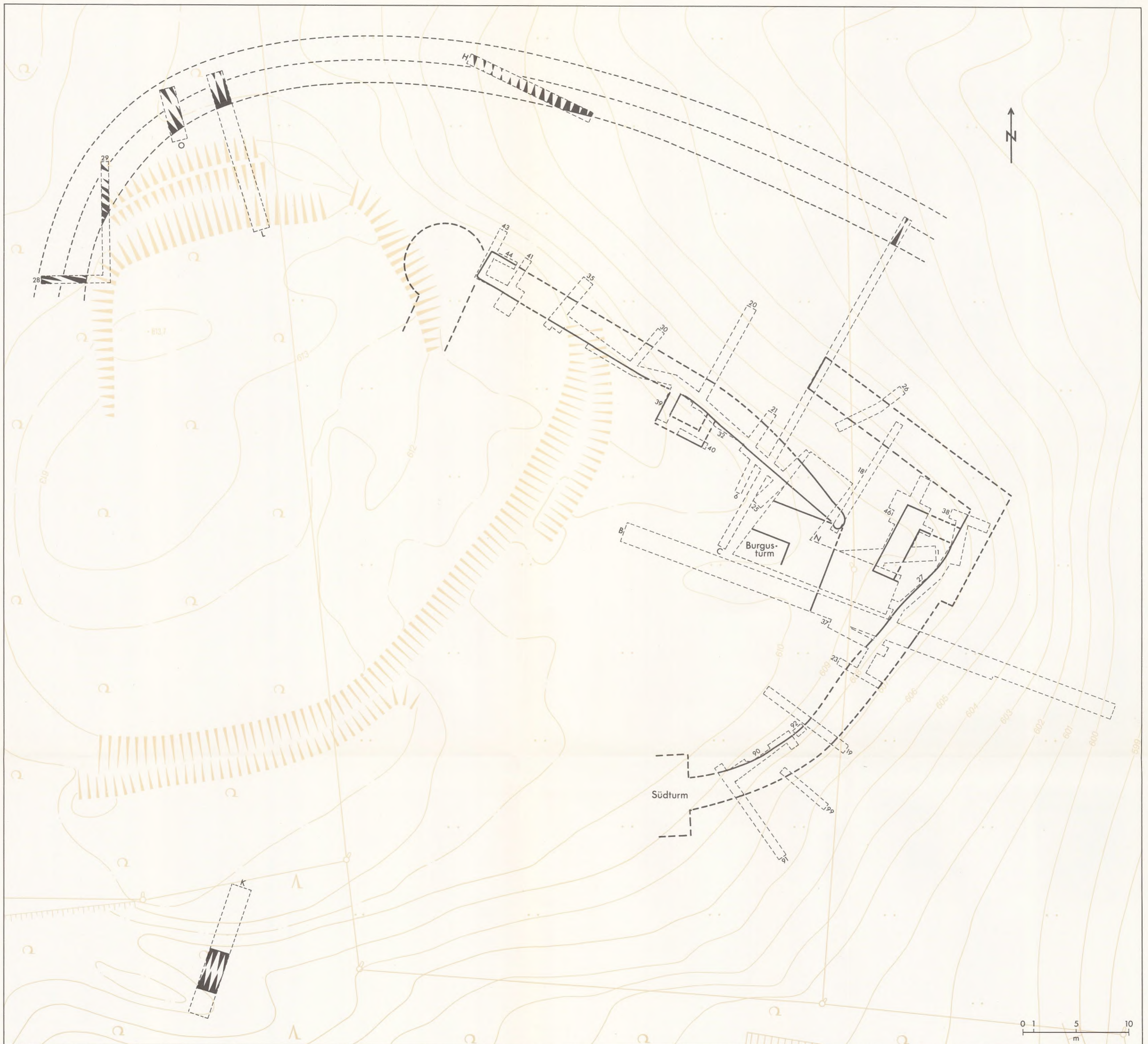
Goldberg, Gemeinde Türkheim, Lkr. Unterallgäu · Südostmauer - Nordmauer der spätrömischen Befestigung. Maßstab 1:250.
