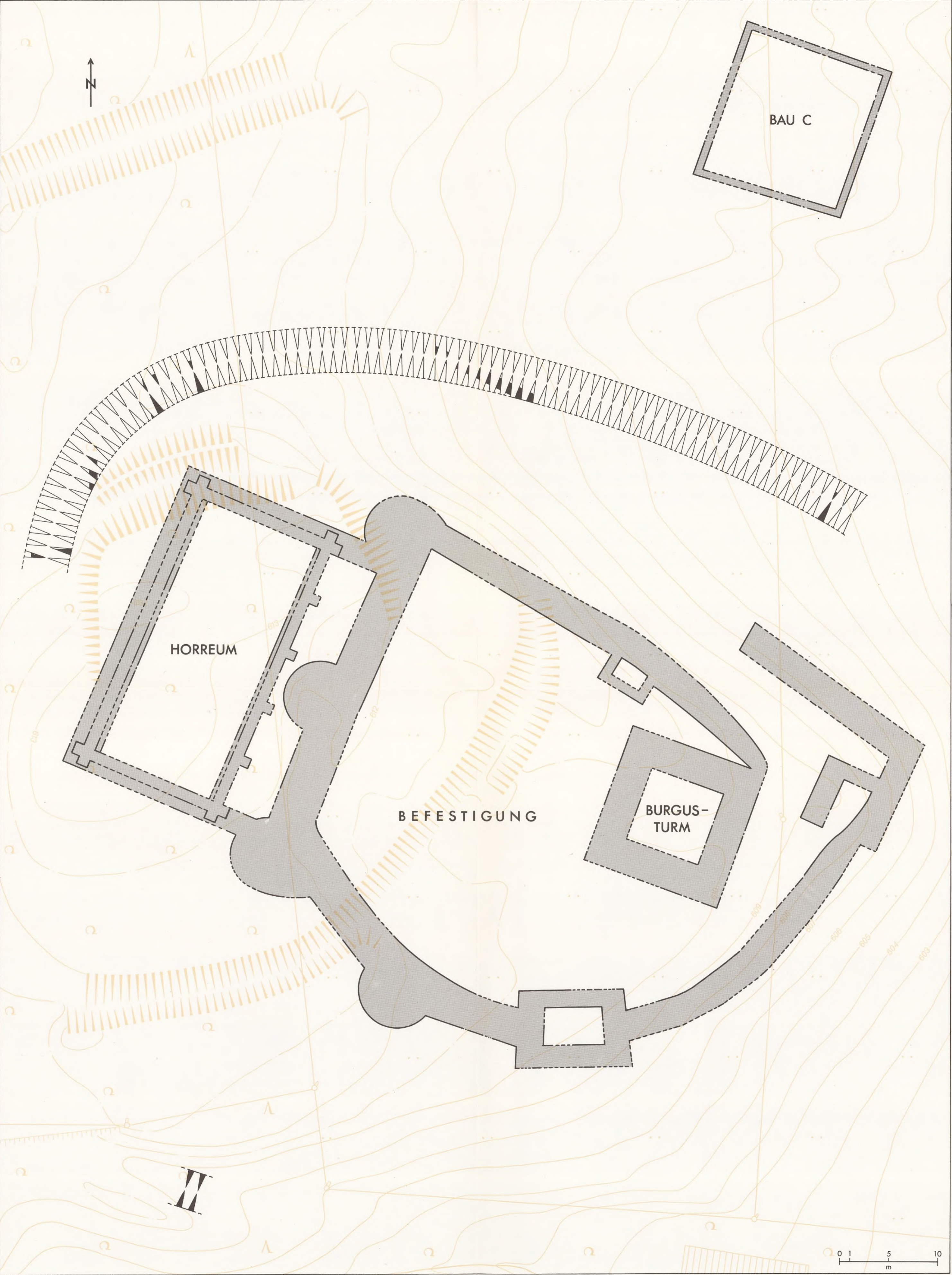
Goldberg, Gemeinde Türkheim, Lkr. Unterallgäu · Gesamtplan der spätrömischen Befestigung. Maßstab 1:250.
