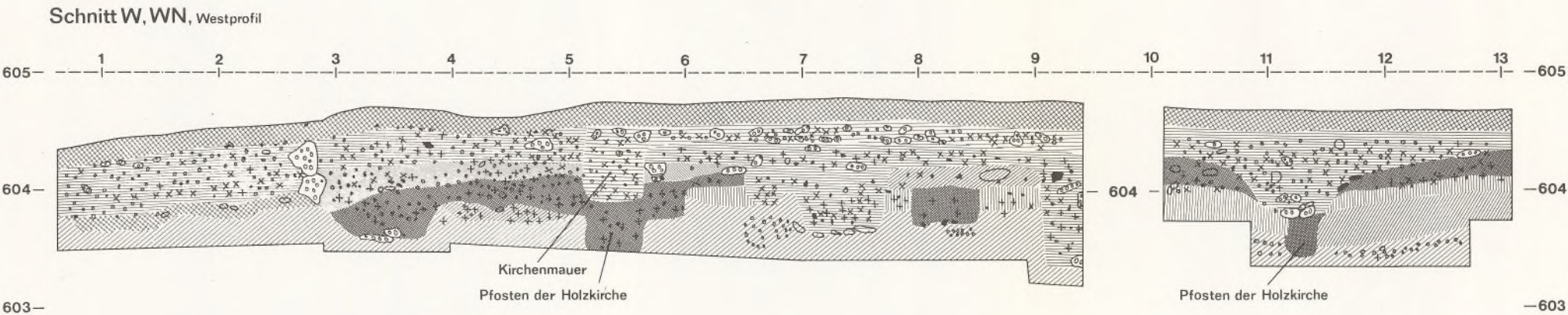
Goldberg, Gemeinde Türkheim, Lkr. Unterallgäu · Profile Schnitte LN, WW und W-WN. Maßstab 1:50.
