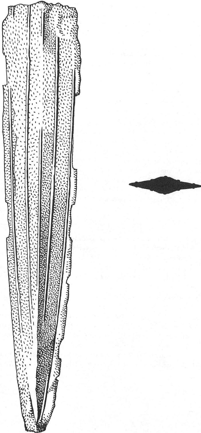
Abb. 21. Sichemfund Nr. 10. Von einem Kurzschwert gebrochene Klinge (F.G.) mit Mittelrippe und fünf Graten. München ÄS 2918. Länge noch 20,1 cm.
