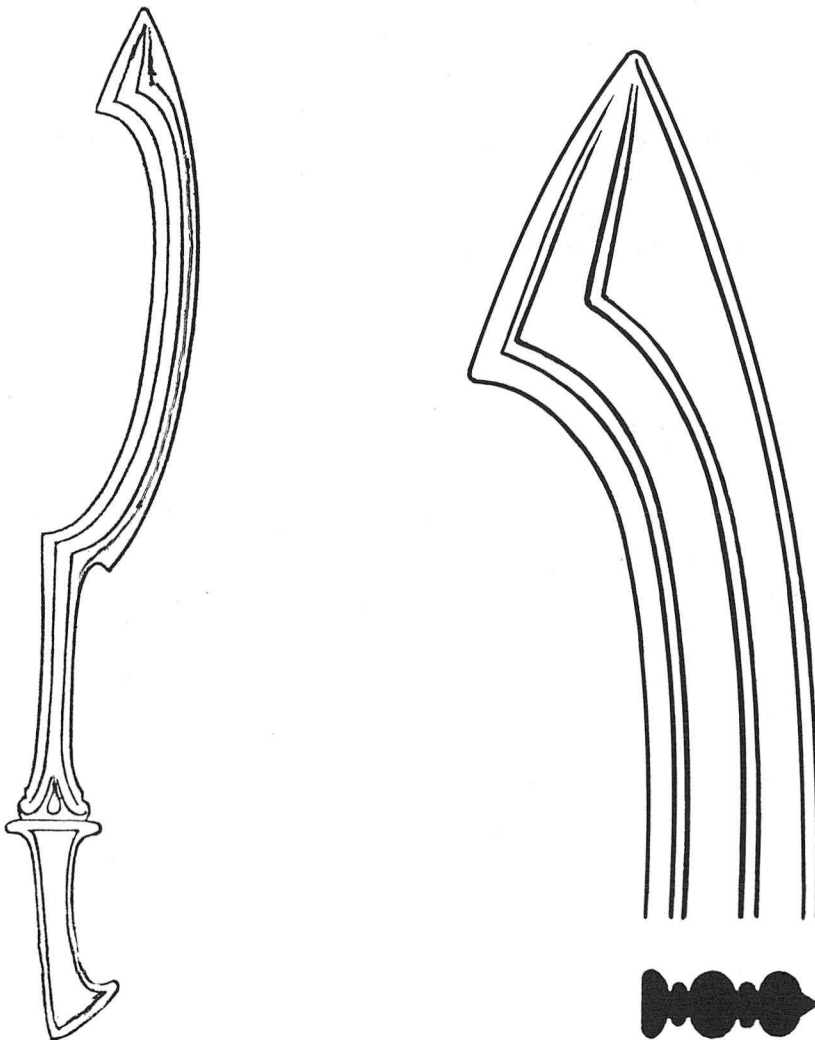
Abb. 41 A. Oberes Klingende des „Schweren Sichelschwertes“ Tutanchamun's. Gruppe IV A, 13. (Verf.).
