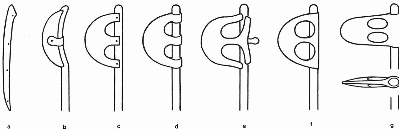
Abb. 5 a–g. Vorderasiatische Beilklingen des 3. und frühen 2. Jahrtausends v. C. (F.G.).
