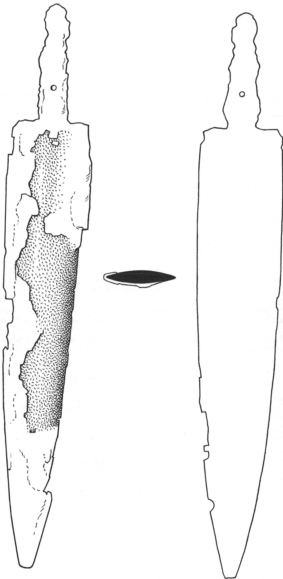
Abb. 12. Sichefund Nr. 7. Glatte Kurzschwertklinge mit Dorn (F.G.). München ÄS 2916. Länge 25,7 cm.
