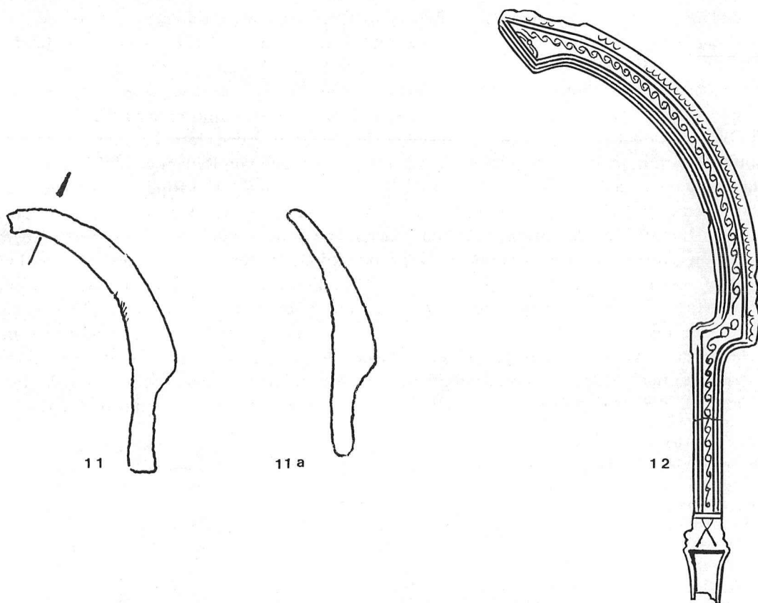
Abb. 39, 11–12. Die Sichelschwerter der Gruppe III, 11–12.
