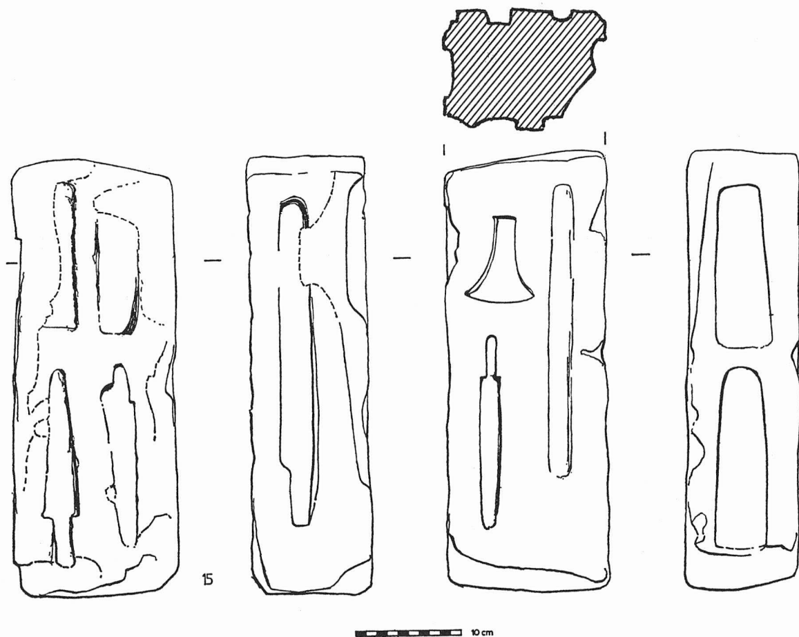
Abb. 32. Gußform aus Sellin's Ausgrabungen in Sichem. Unter der Bezeichnung „Haus des Blinden“ im Rijksmuseum van Oudheden, Leiden: V.J. Kerkhof, OMRO L, 1962, p. 98 fig. 30 no 15.
