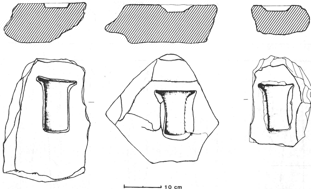
Abb. 33. Gußformen aus Serabit el-Khadim/Sinai. Frühe 18. Dynastie. Nach I. Beit Arie in: Levant XVII , 1985, p. 98 fig. 6, no 1, 2, 4.
