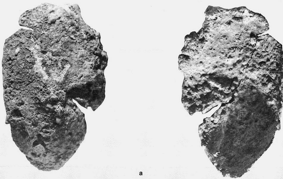
a) Sichemfund Nr. 14. Gußrest aus einem Schmelztiegel. München ÄS 2911. Größter Dm 11,5 cm.
