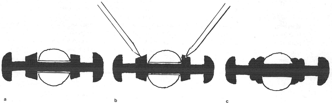
Abb. 8a–c. Querschnitte durch den Stiel des Sichelschwertes aus Sichem zur Veranschaulichung der Tauschier Technik der Mittelrippe. (Verf.).
