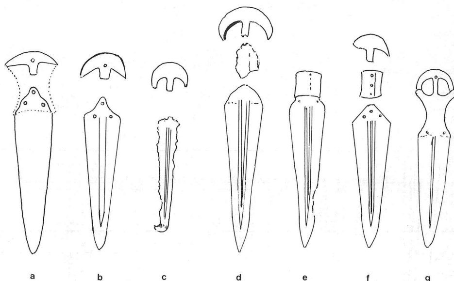
Abb. 16a–g. Dolchklängen mit den zugehörigen mondsichelförmigen Knäufen (Verf.). – a/b) Aus Ras Shamra-Ugarit. Nach C. F. A. Schaeffer, Ugaritica I, p. 50 fig. 18 no 23–25. – c) Aus Kôm el-Hisn/Westdelta, Nach ASAE XXXXVI, 1947, pl. LVI. – d) Aus Aniba/Nubien. Nach G. Steindorff, Aniba I, Taf. 70, 1. – e) Aus Byblos. Nach M. Dunand, Fouilles de Byblos II, pl. LXVIII, no 9666. – f) Aus Aniba/Nubien. Nach G. Steindorff, o.c. Taf. 70, 2. – g) Aus Byblos. Nach M. Dunand, o.c. II, pl. LXII no 9158.
