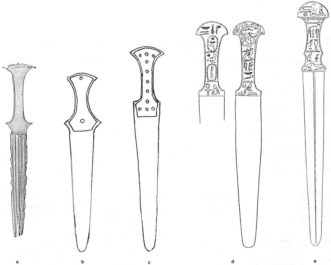
Abb. 20. Griffformen der Kurzscherer der Hyksoszeit. 17. Jahrh. – 1550 v. C.
